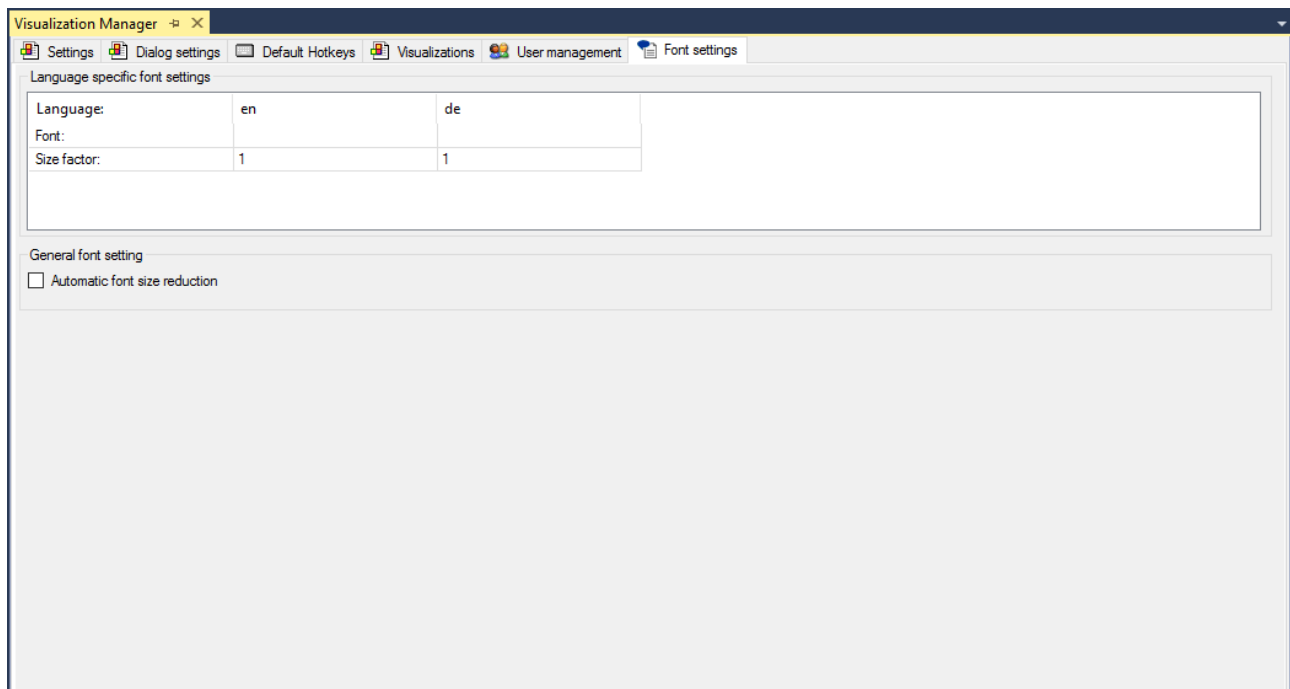
Sprachspezifische Schriftarteinstellungen
