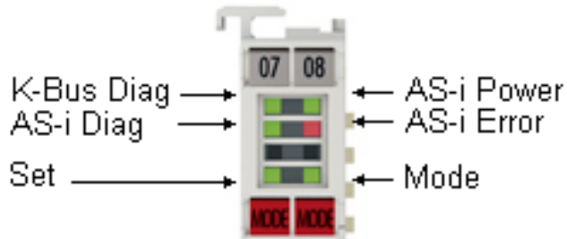
Fig. 37: LEDs
