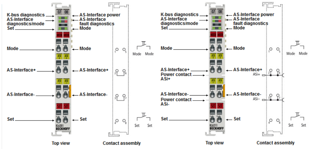
Fig. 1: KL6201, KL6211
