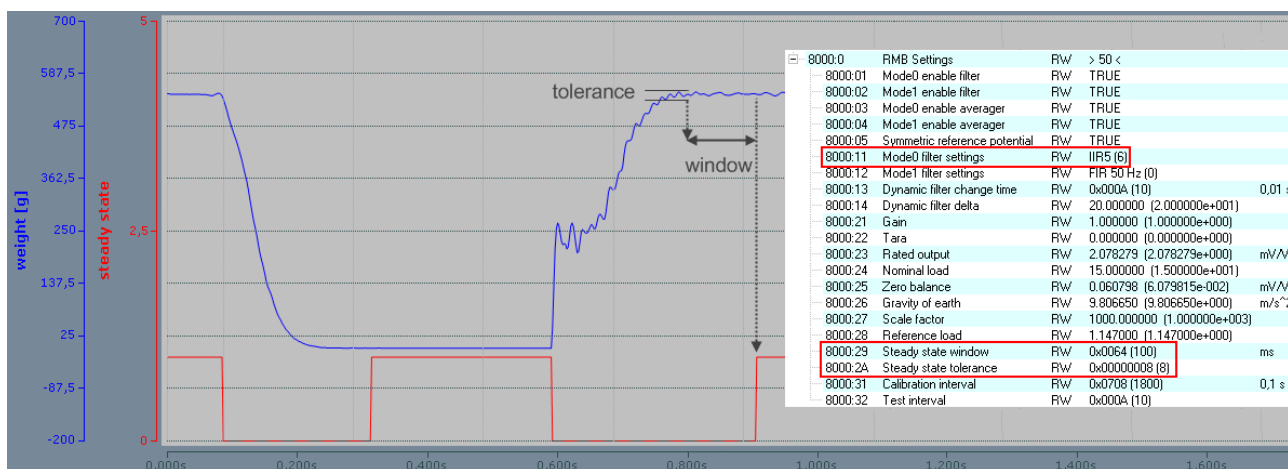
Abb. 19: Sprunghafte Entlastung und anschließende erneute Belastung einer Wägezelle
