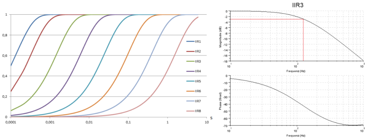
Abb. 5: Sprungantwort und Bodediagramm der IIR-Filter
