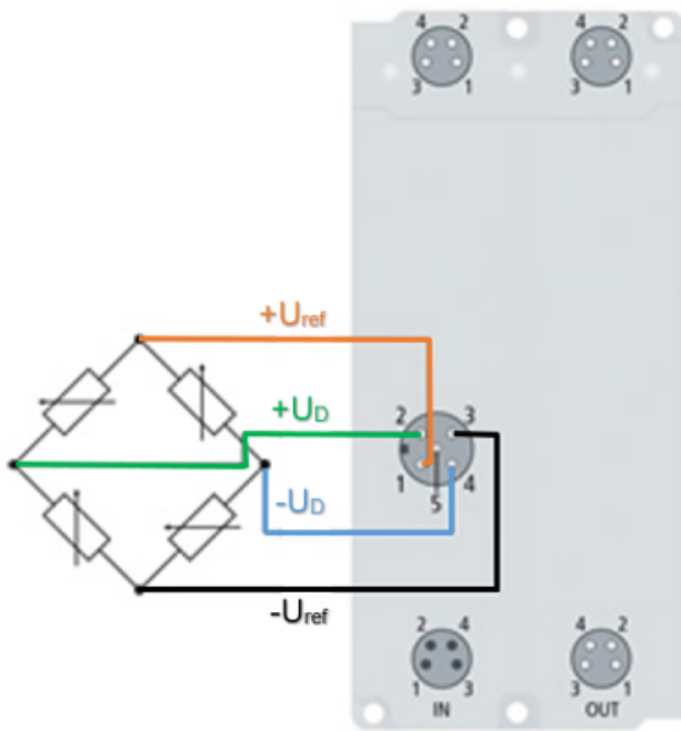
Abb. 22: EP3356: Anschluss des Lastsensors/Vollbrücke
