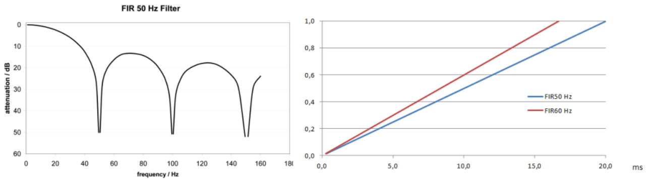
Abb. 4: Notch-Kennlinie/Amplitudengang und Sprungantwort der FIR-Filter
