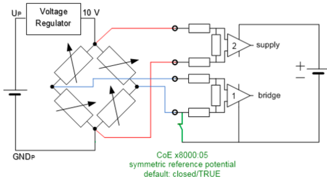
Abb. 17: Interner Schalter zur Erhöhung der Messgenauigkeit
