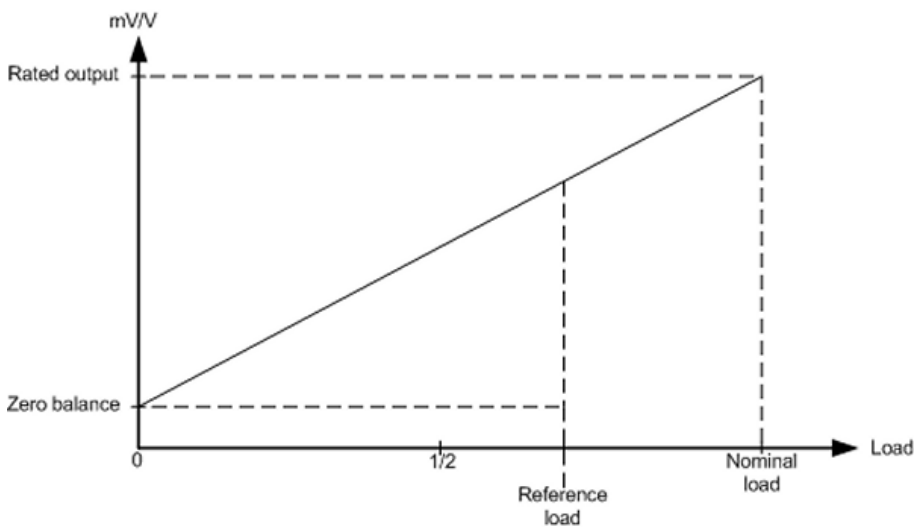
Abb. 20: Anpassen an die Sensorkennlinie
