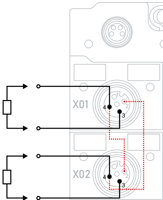
Zwei Aktoren mit zwei Kabeln
