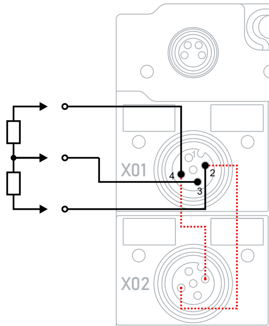
Zwei Aktoren mit nur einem Kabel
