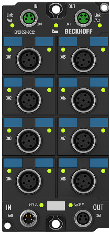
Abb. 2: EPX1058-0022 - Achtkanalige, digitale EtherCAT Box für NAMUR-Sensoren, Ex i
