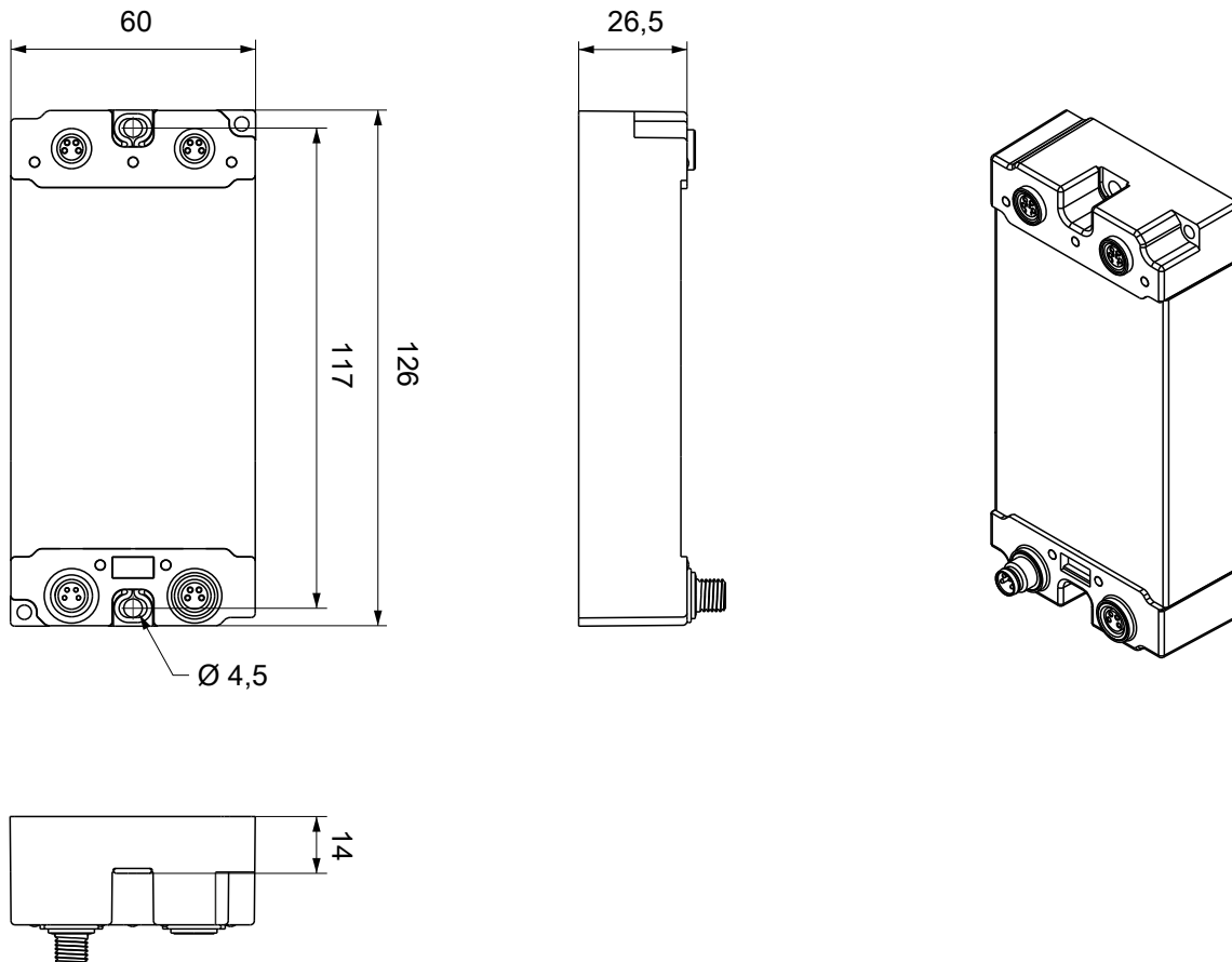
Abb. 3: EPX-EtherCAT-Box - Abmessungen
