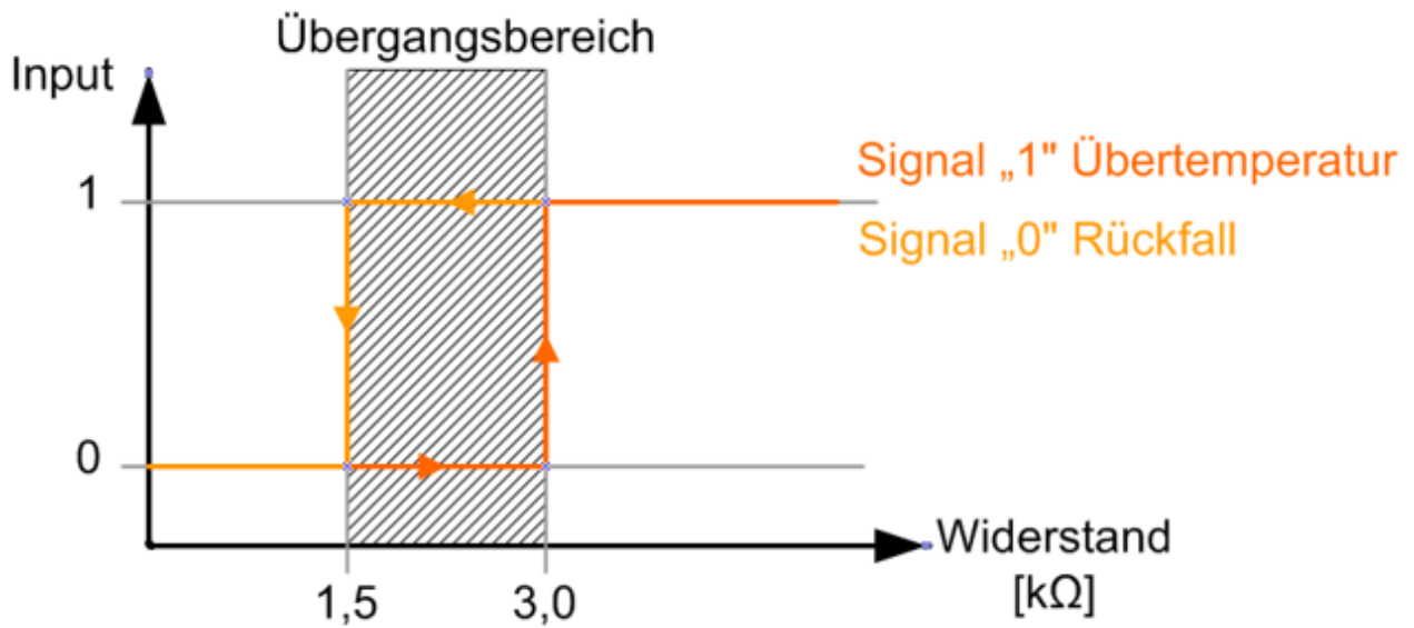
Abb. 135: Schaltverhalten
