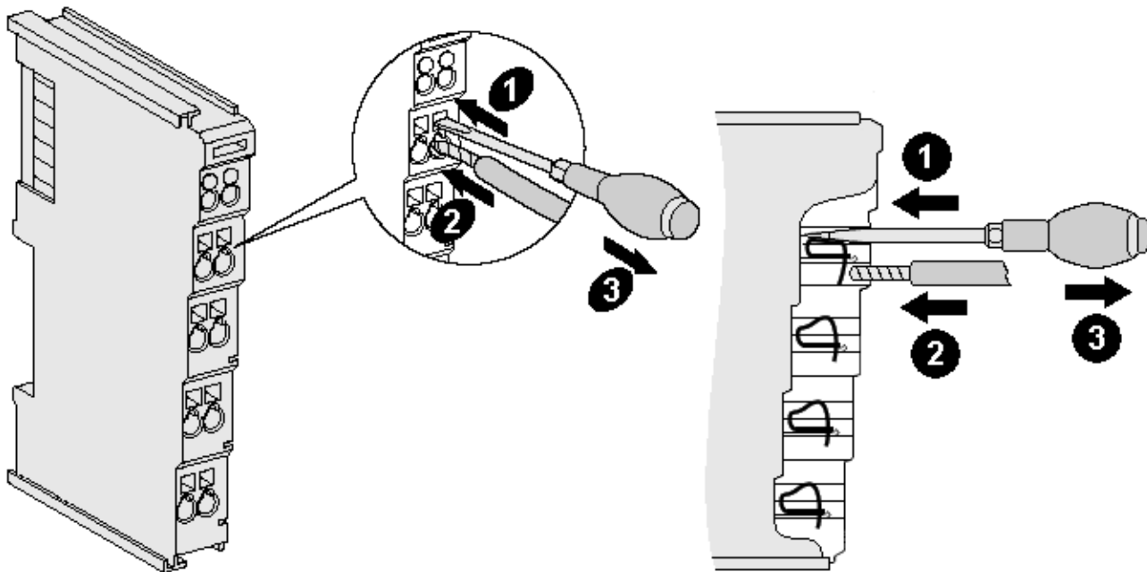
Abb. 19: Anschluss einer Leitung an eine Klemmstelle
