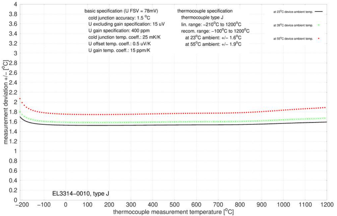
附图 40: EL3314-0010、EL3314-0020 和 EL3314-0030（等同于 EL3314-0010），J 型
