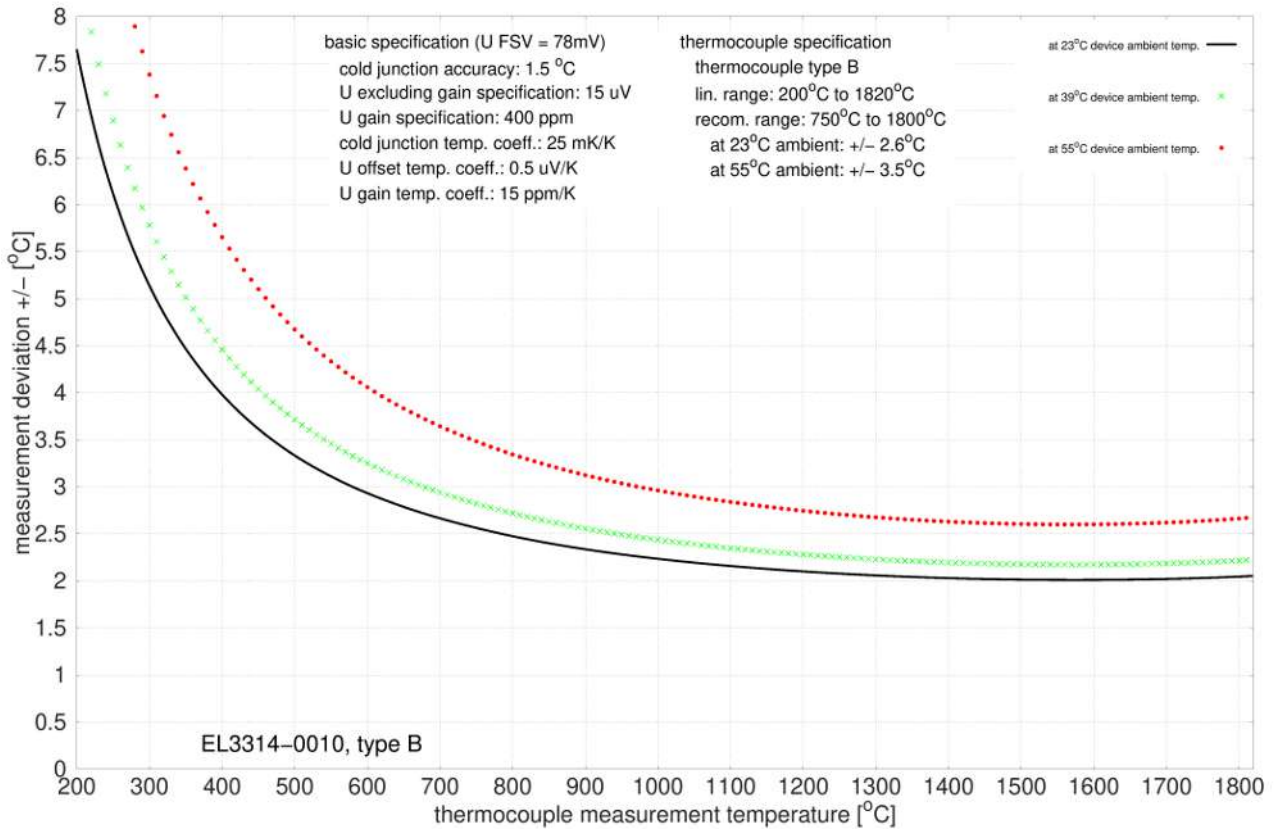
附图 24: EL3314-0010、EL3314-0020 和 EL3314-0030 (等同于 EL3314-0010) , B 型
