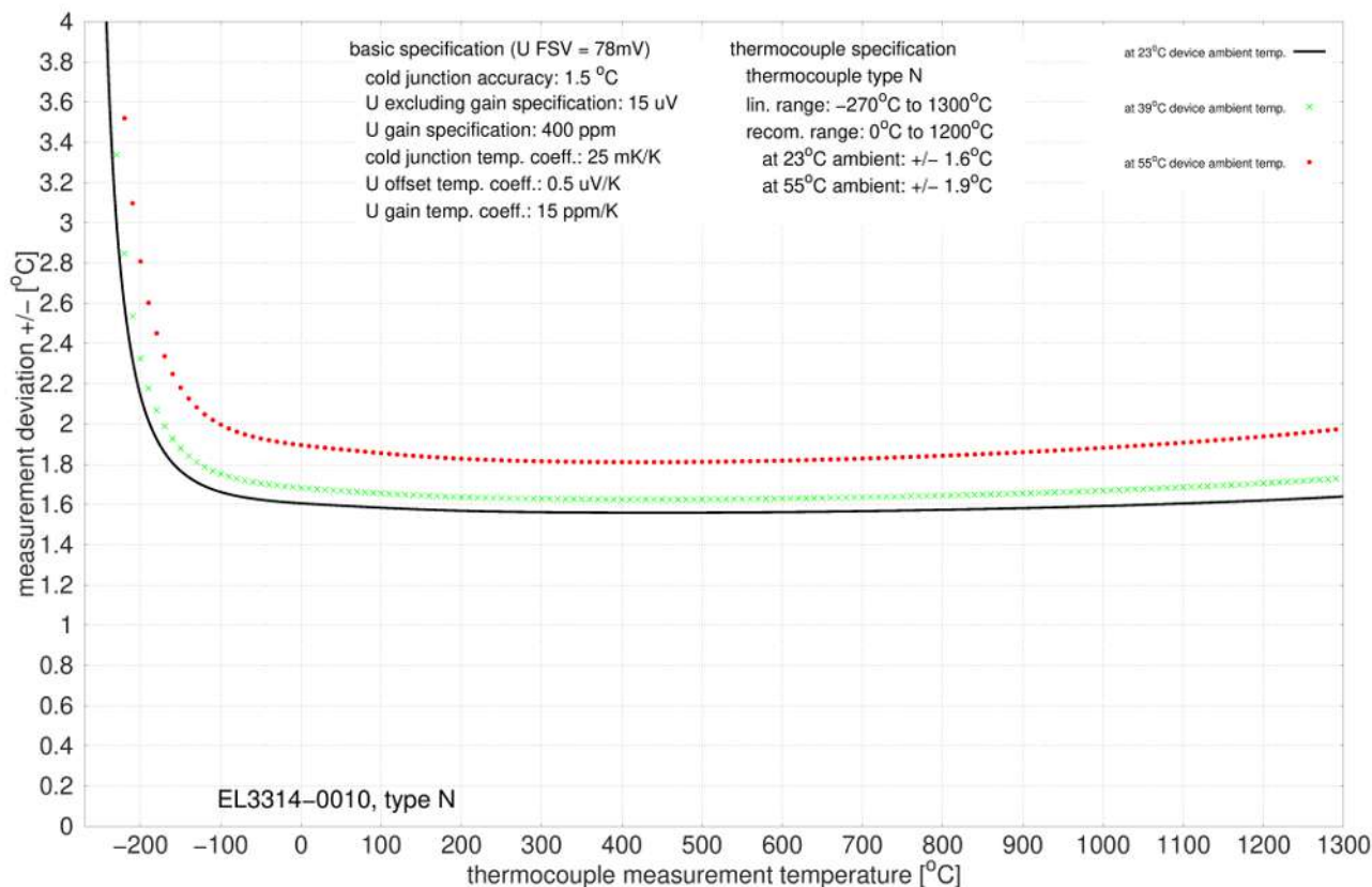
附图 43: EL3314-0010、EL3314-0020 和 EL3314-0030（等同于 EL3314-0010），N 型
