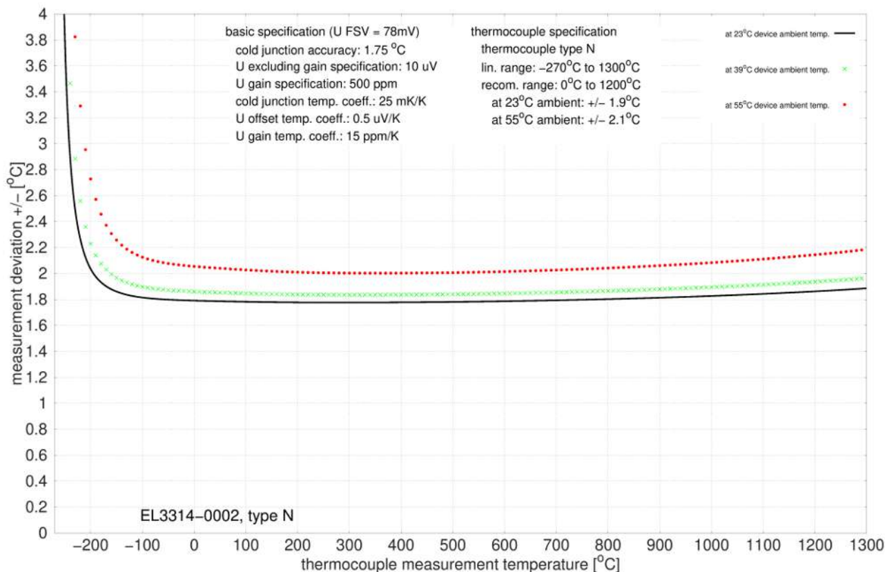
附图 17: EL3314-0002 和 EL3314-0092 (对应 EL3314-0002), N 型
