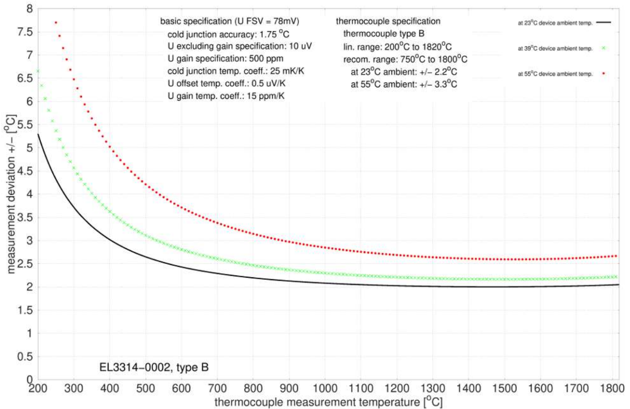
附图 65: EL3314-0002 和 EL3314-0092 (对应 EL3314-0002), B 型
