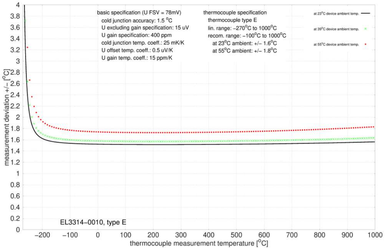
附图 52: EL3314-0010、EL3314-0020 和 EL3314-0030 (等同于 EL3314-0010) , E 型
