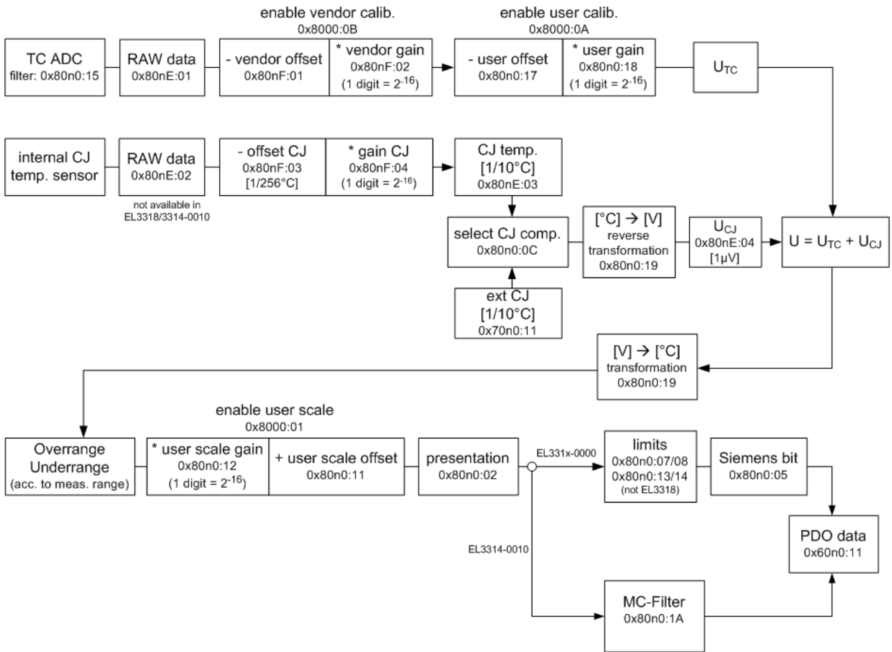
附图 214: EL33xx 数据流
