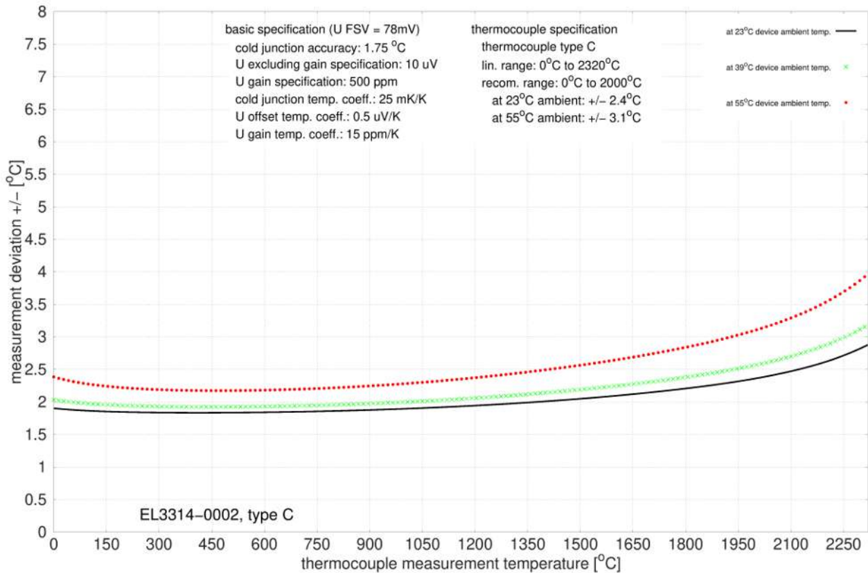
附图 12: EL3314-0002 和 EL3314-0092 (对应 EL3314-0002), C 型
