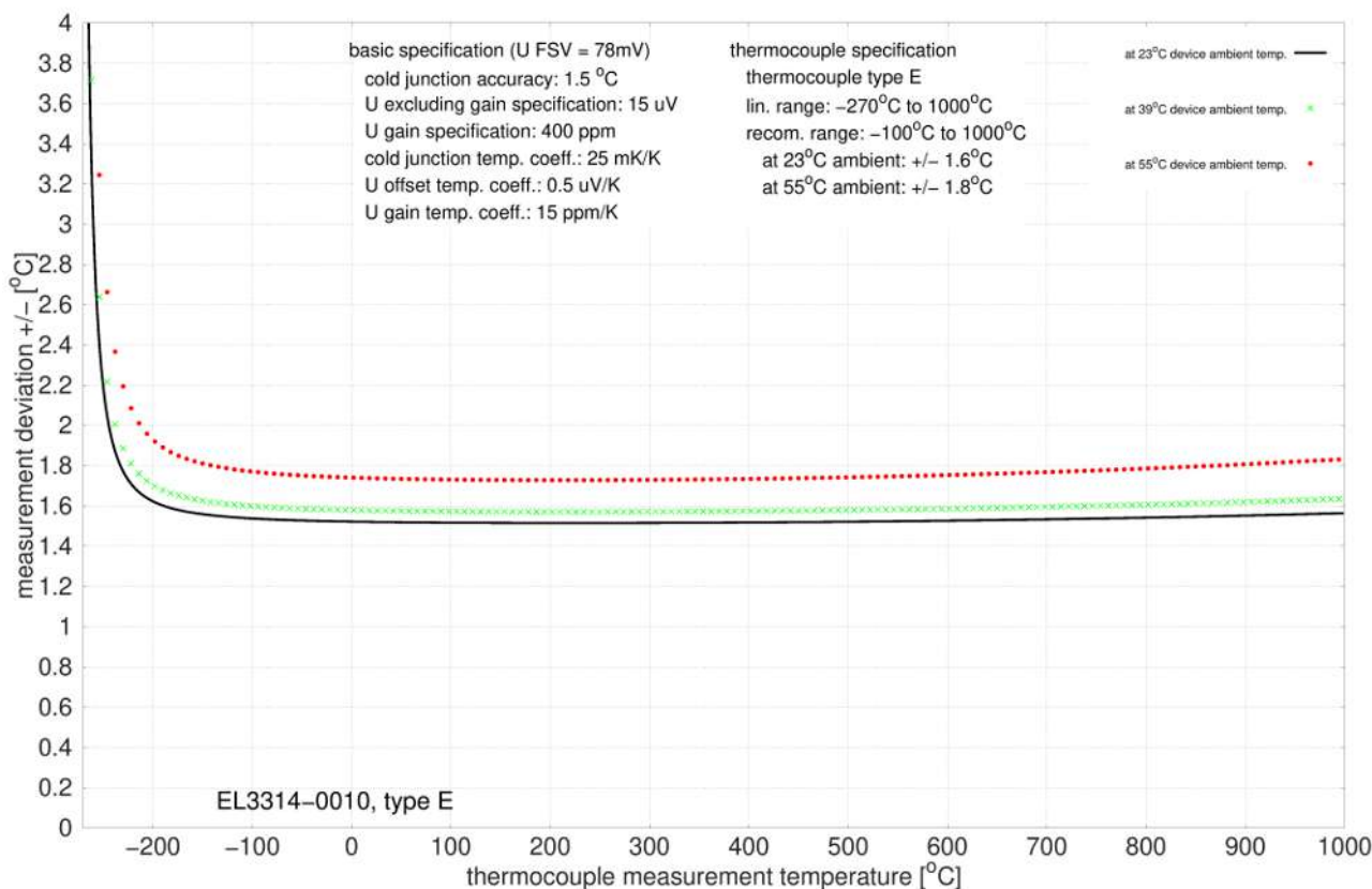
附图 39: EL3314-0010、EL3314-0020 和 EL3314-0030 (等同于 EL3314-0010) , E 型
