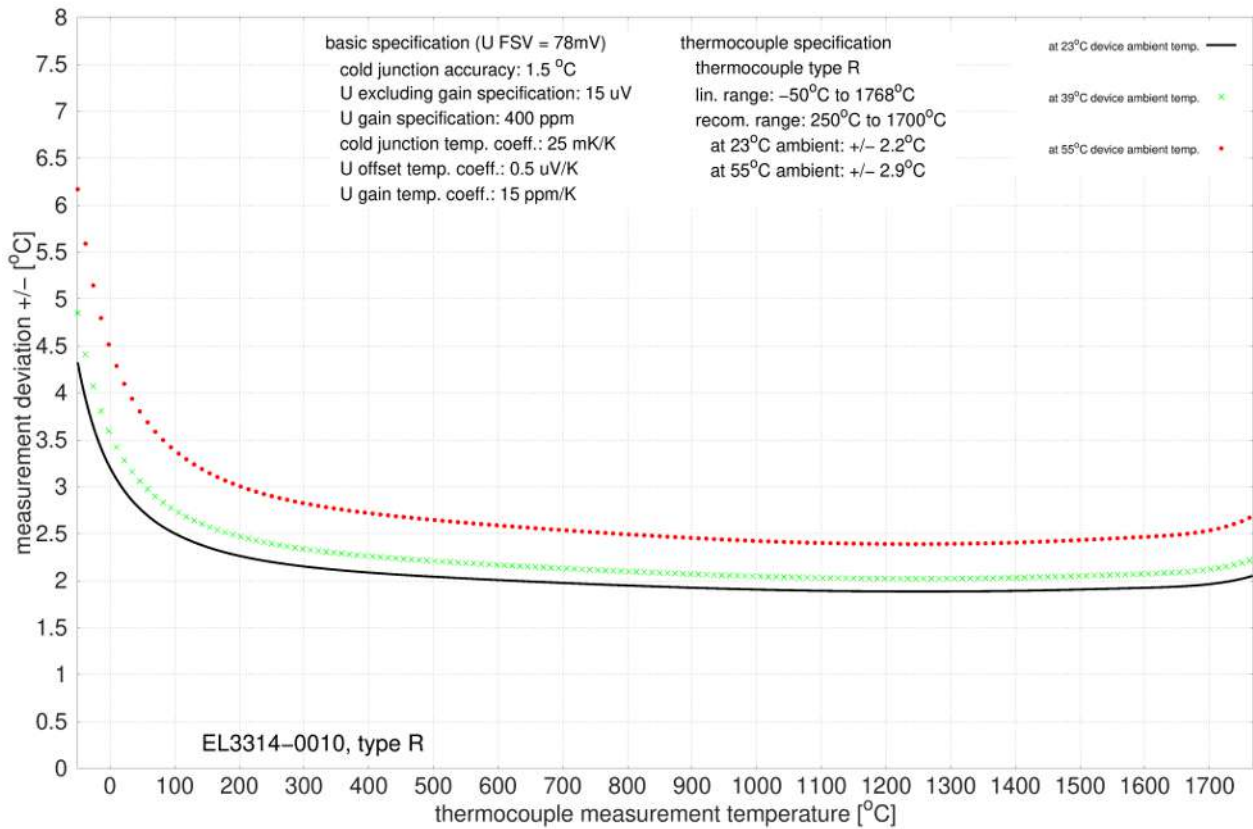
附图 44: EL3314-0010、EL3314-0020 和 EL3314-0030 (等同于 EL3314-0010), R 型
