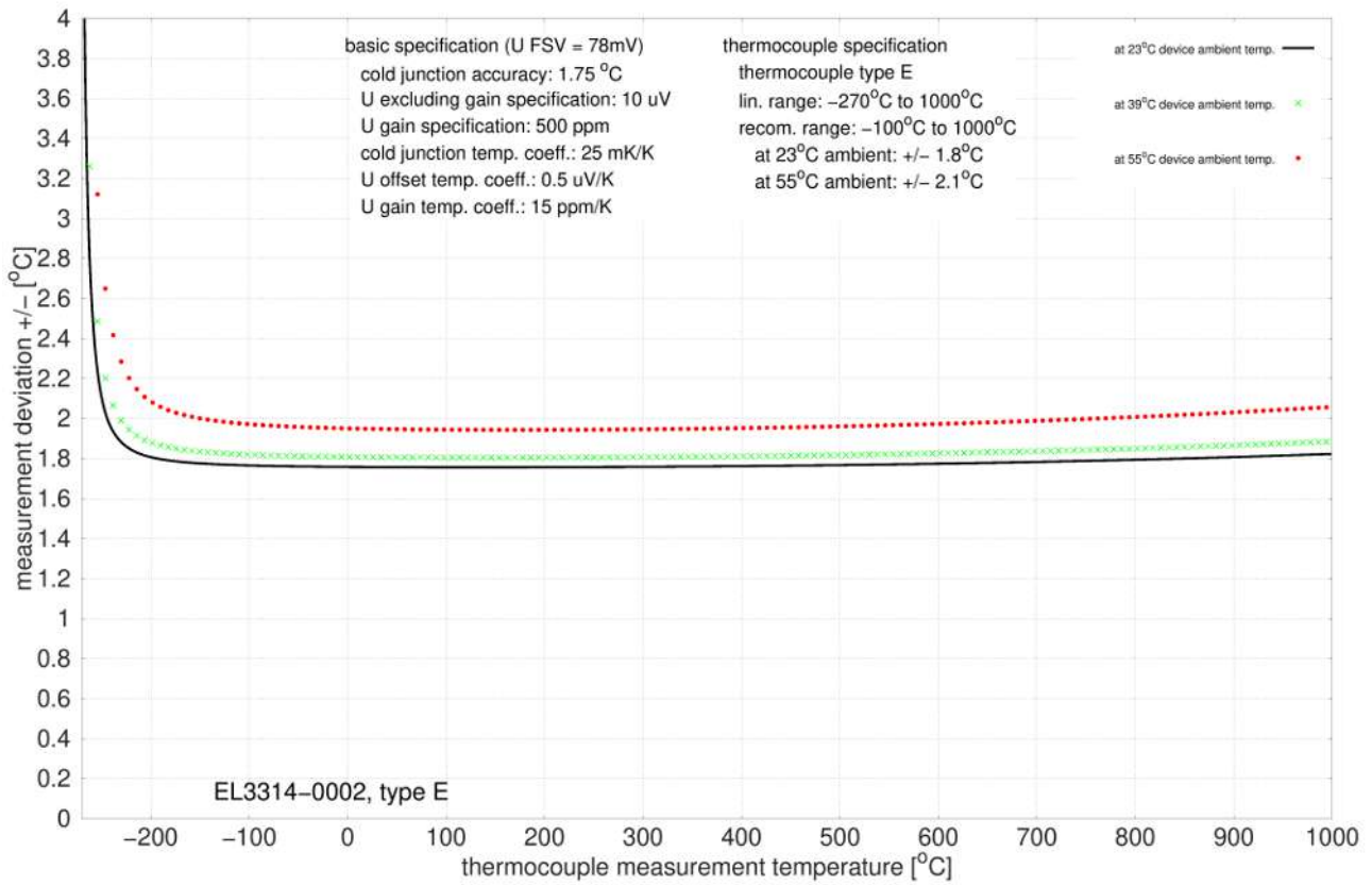
附图 67: EL3314-0002 和 EL3314-0092 (对应 EL3314-0002), E 型
