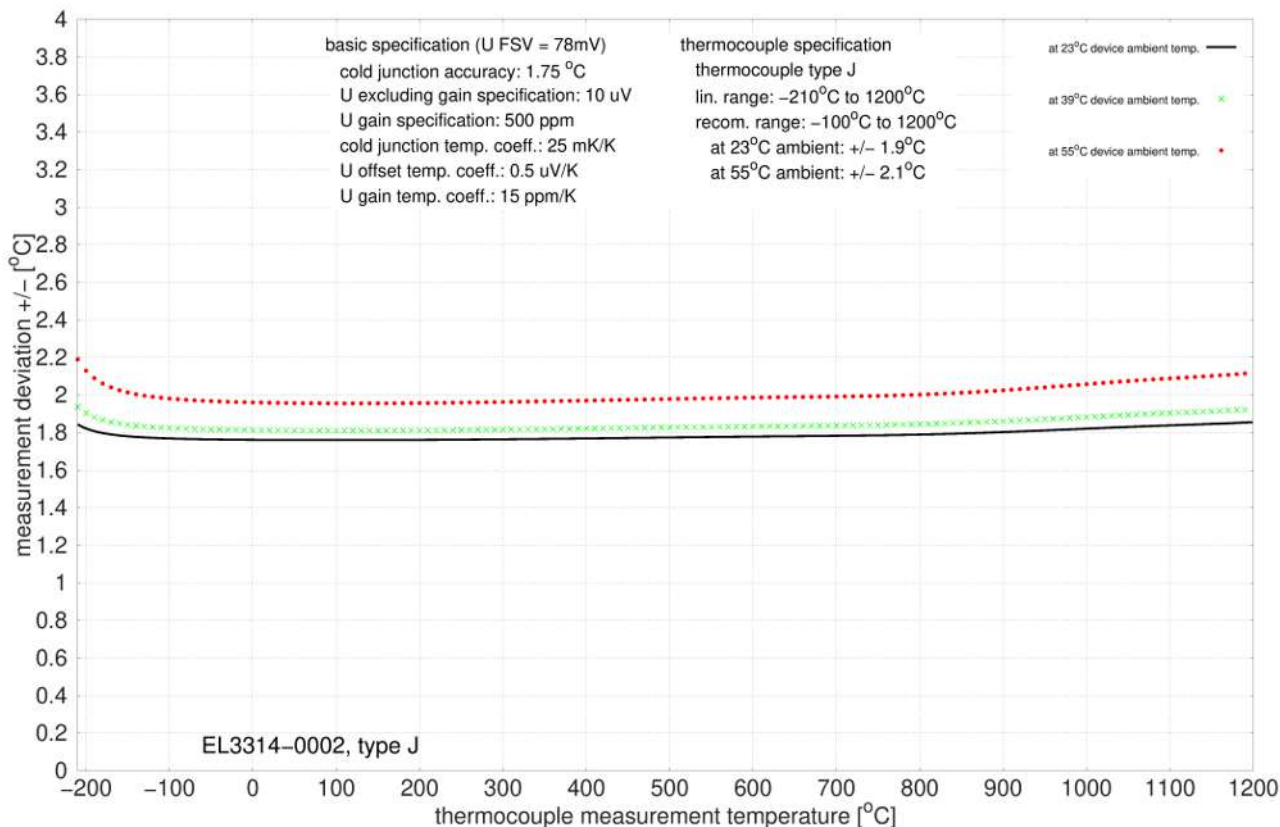
附图 68: EL3314-0002 和 EL3314-0092 (对应 EL3314-0002), J 型
