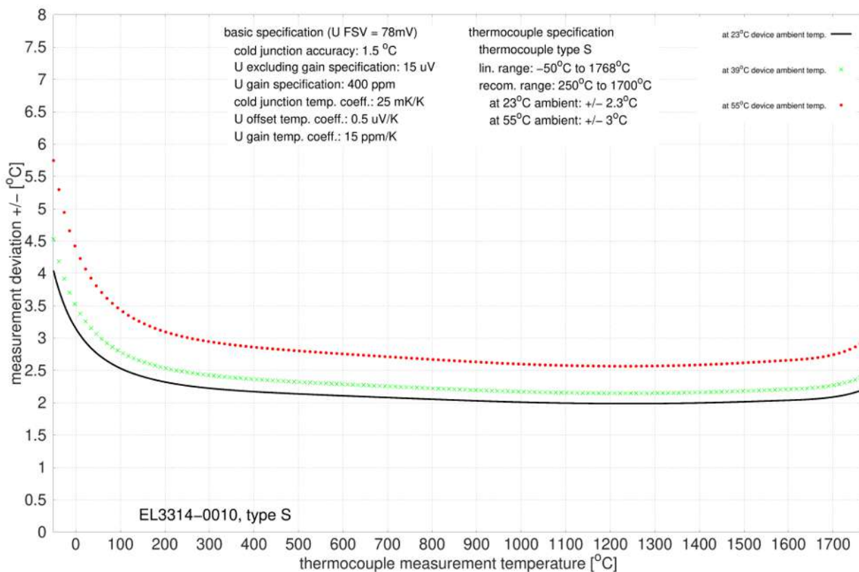
附图 45: EL3314-0010、EL3314-0020 和 EL3314-0030（等同于 EL3314-0010），S 型
