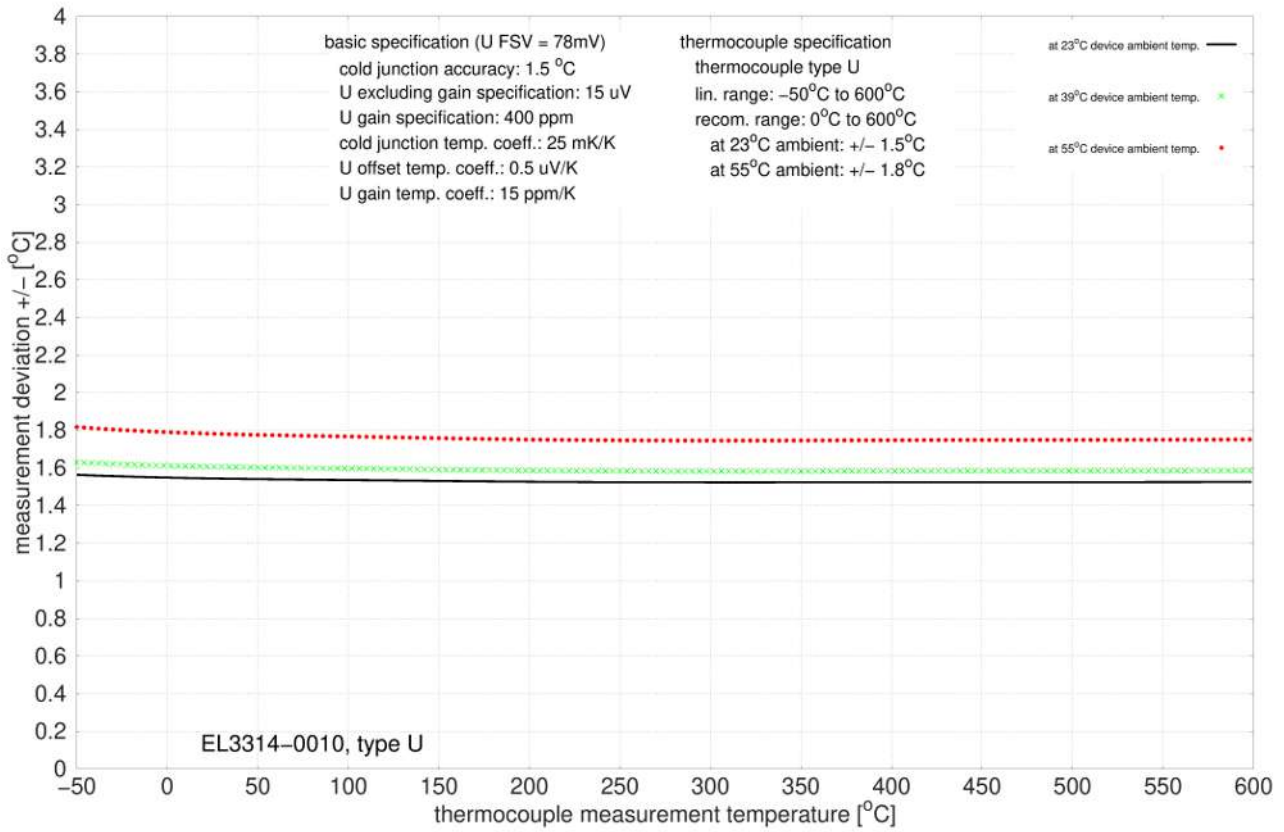
附图 60: EL3314-0010、EL3314-0020 和 EL3314-0030 (等同于 EL3314-0010), U 型
