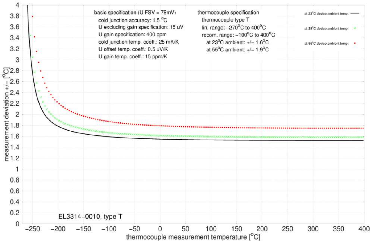
附图 59: EL3314-0010、EL3314-0020 和 EL3314-0030 (等同于 EL3314-0010), T 型
