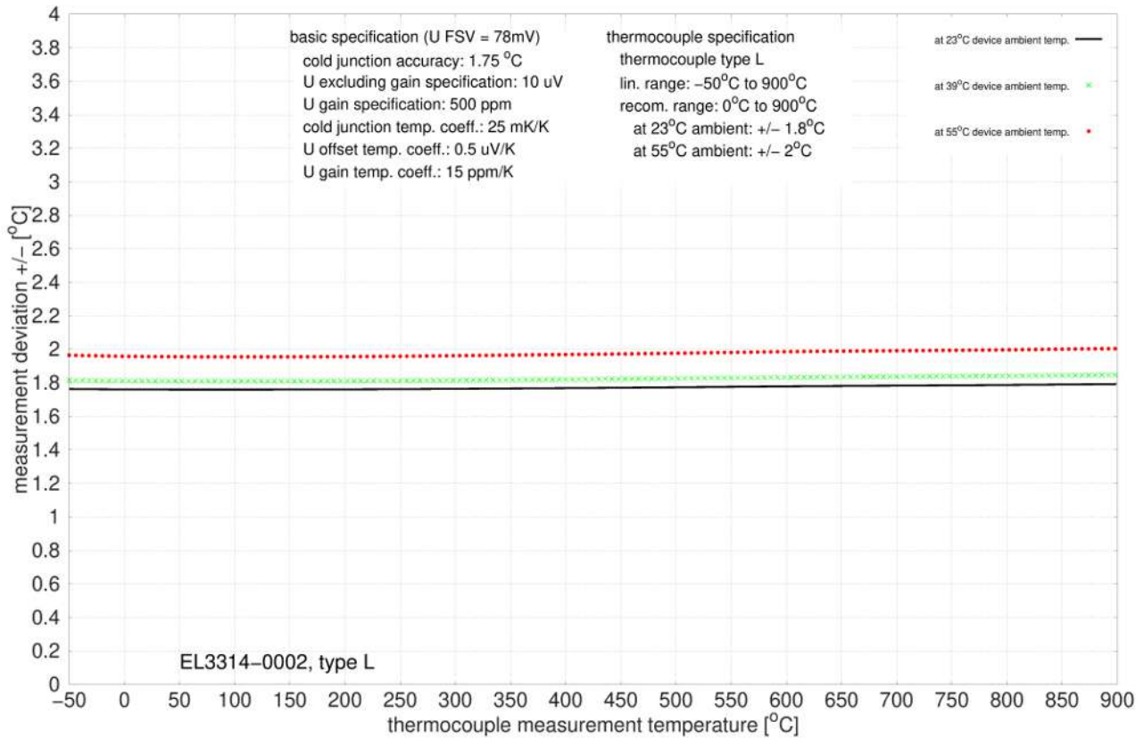
附图 70: EL3314-0002 和 EL3314-0092 (对应 EL3314-0002), L 型
