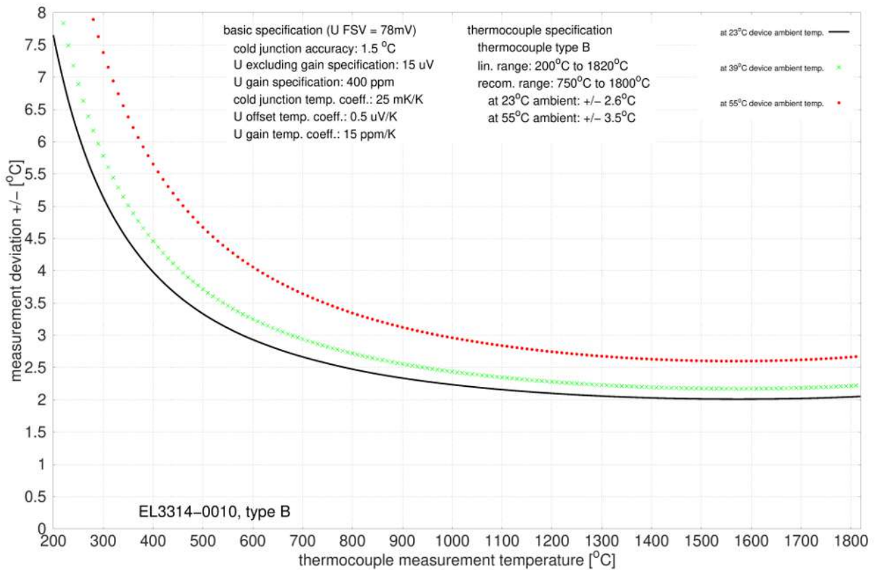
附图 50: EL3314-0010、EL3314-0020 和 EL3314-0030（等同于 EL3314-0010），B 型
