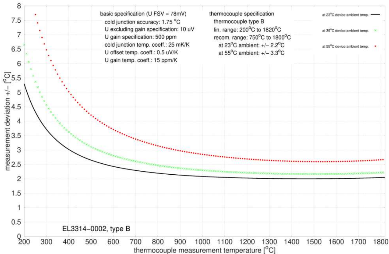
附图 11: EL3314-0002 和 EL3314-0092 (对应 EL3314-0002), B 型
