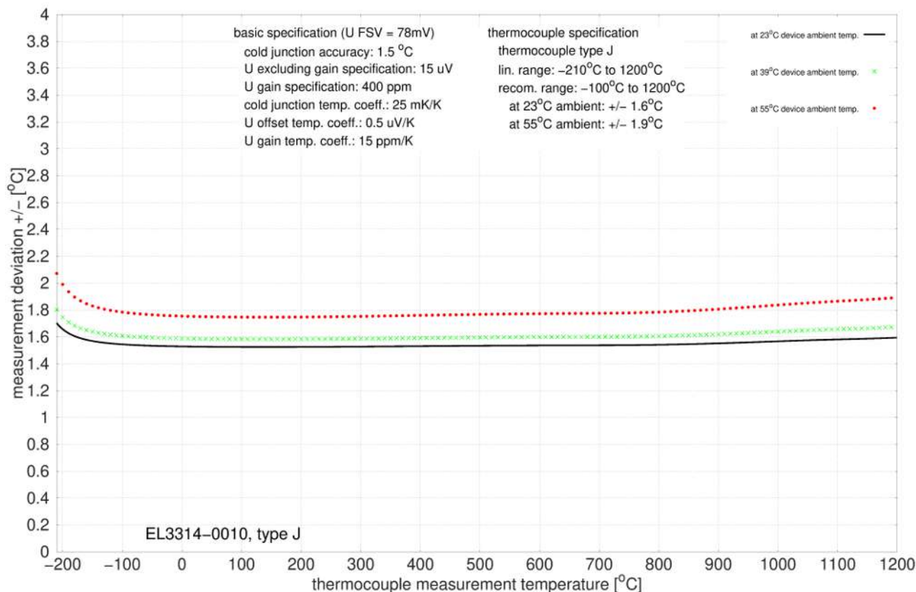
附图 53: EL3314-0010、EL3314-0020 和 EL3314-0030（等同于 EL3314-0010），J 型
