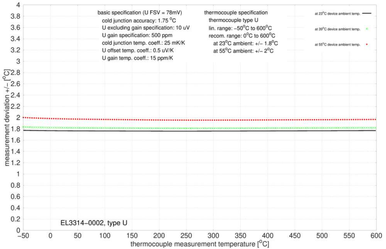
附图 21: EL3314-0002 和 EL3314-0092 (对应 EL3314-0002), U 型
