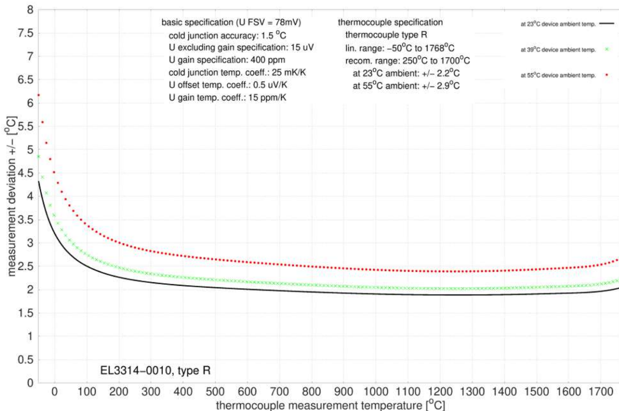
附图 31: EL3314-0010、EL3314-0020 和 EL3314-0030 (等同于 EL3314-0010), R 型
