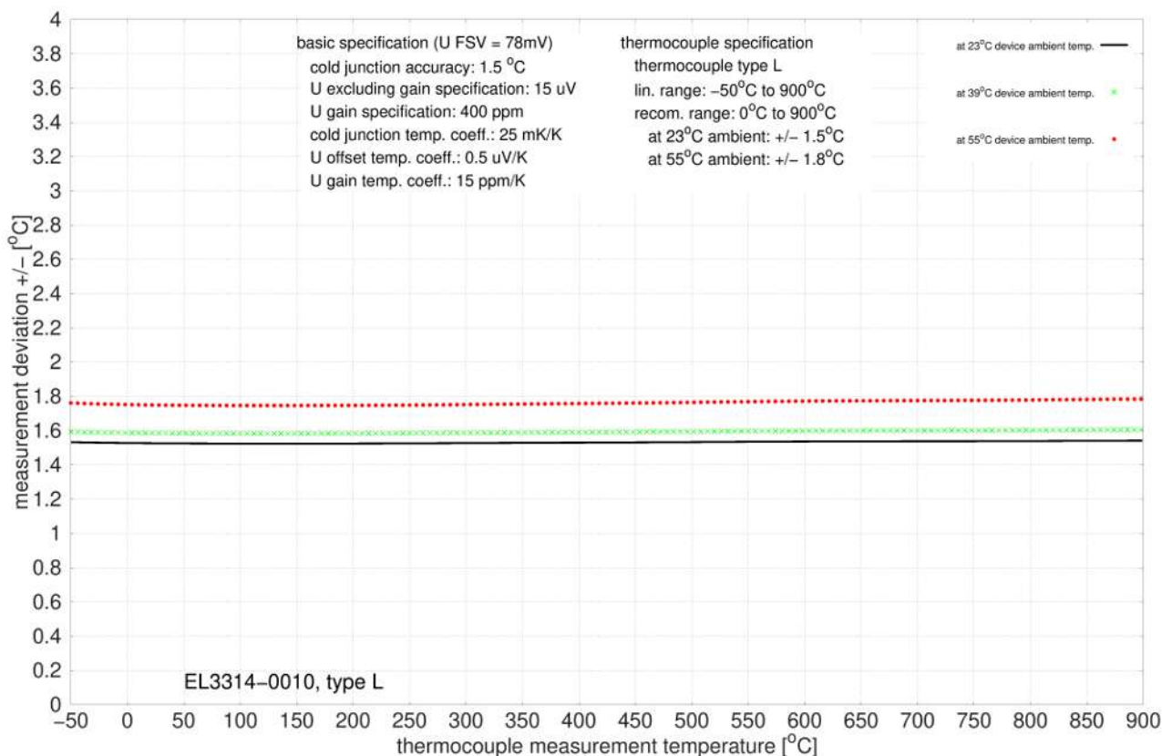
附图 55: EL3314-0010、EL3314-0020 和 EL3314-0030 (等同于 EL3314-0010), L 型
