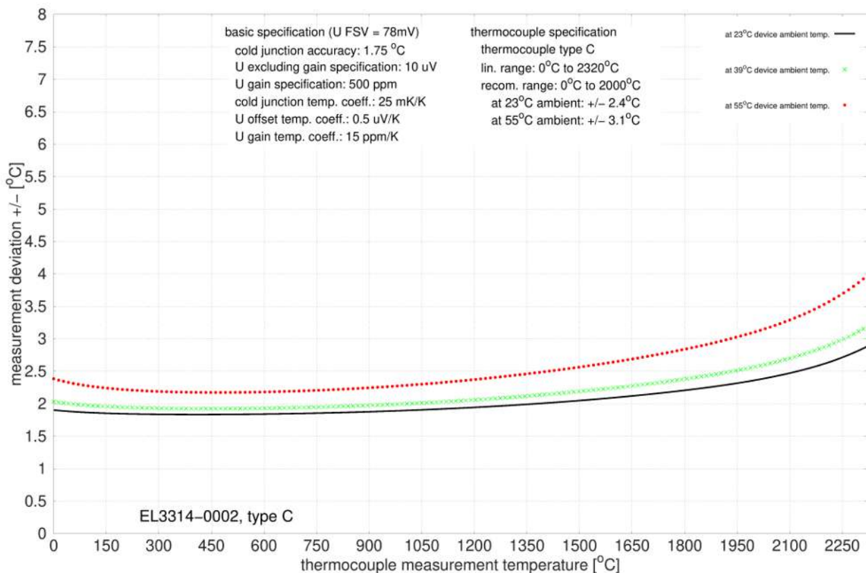
附图 66: EL3314-0002 和 EL3314-0092 (对应 EL3314-0002), C 型
