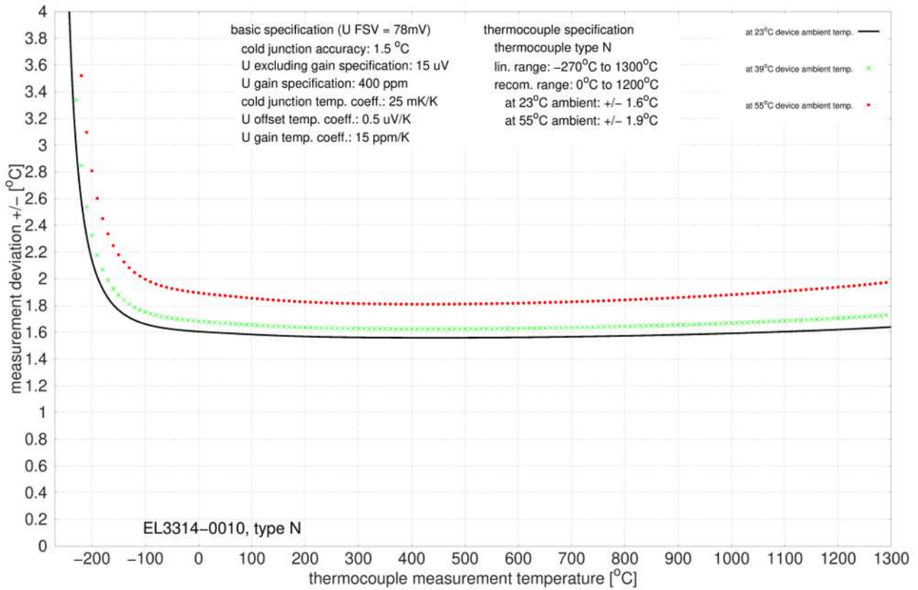
附图 56: EL3314-0010、EL3314-0020 和 EL3314-0030（等同于 EL3314-0010），N 型
