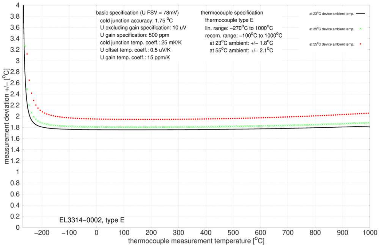
附图 13: EL3314-0002 和 EL3314-0092 (对应 EL3314-0002), E 型
