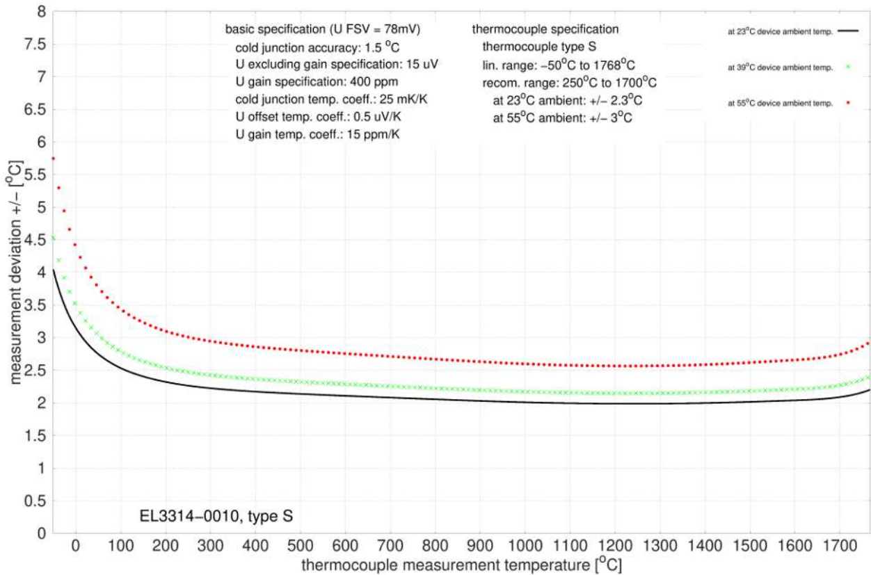
附图 32: EL3314-0010、EL3314-0020 和 EL3314-0030（等同于 EL3314-0010），S 型
