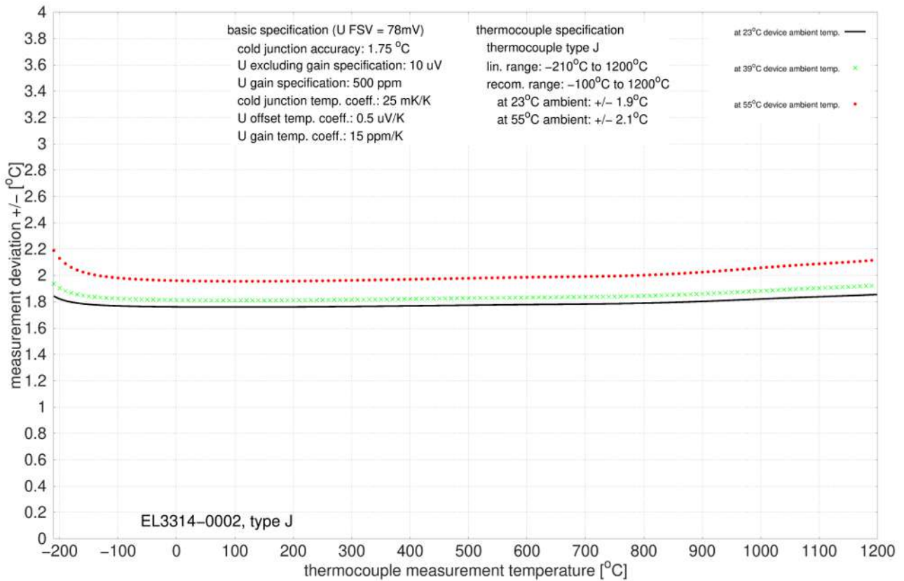
附图 14: EL3314-0002 和 EL3314-0092 (对应 EL3314-0002), J 型
