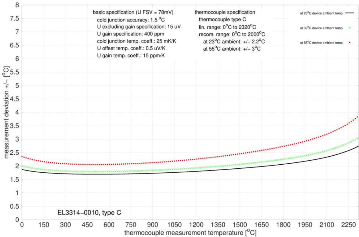
附图 38: EL3314-0010、EL3314-0020 和 EL3314-0030 (等同于 EL3314-0010), C 型
