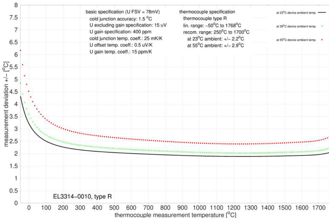
附图 57: EL3314-0010、EL3314-0020 和 EL3314-0030 (等同于 EL3314-0010), R 型
