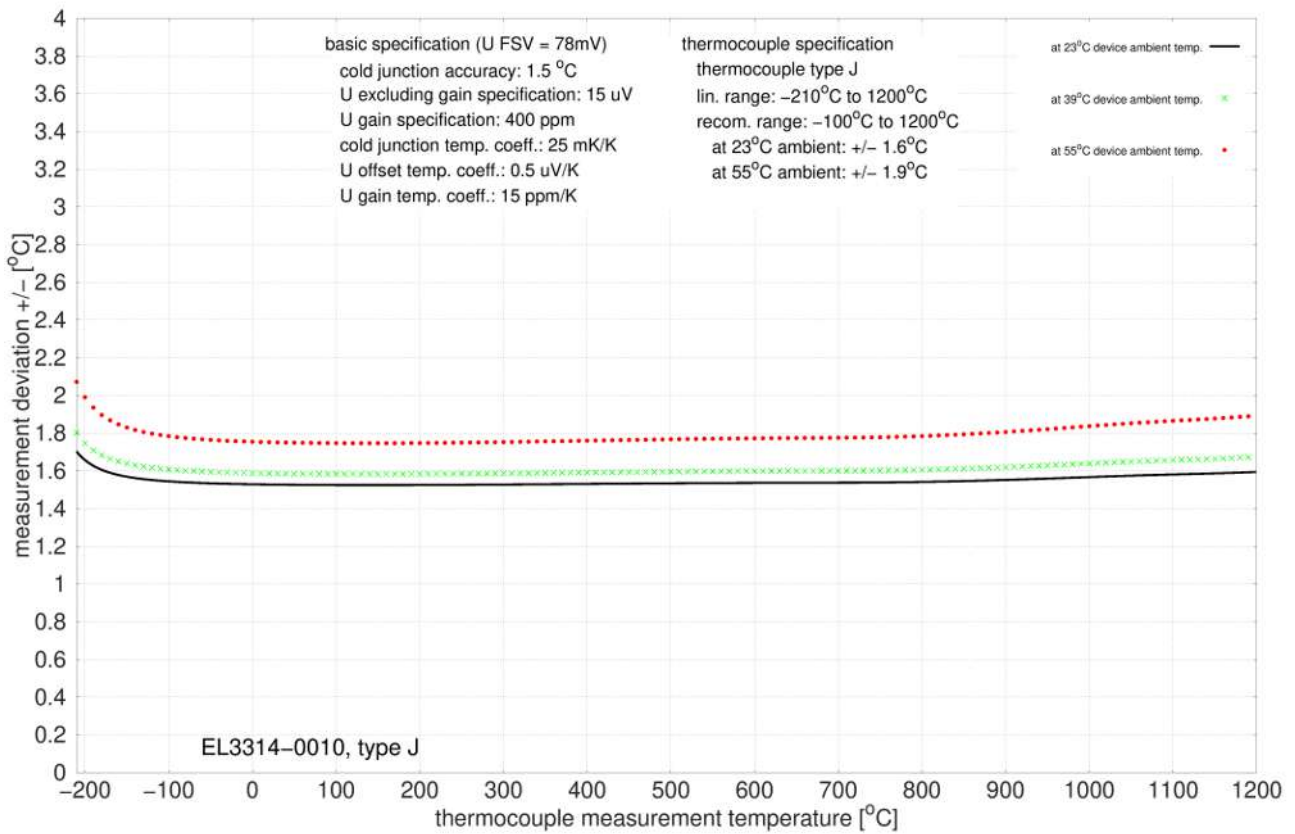
附图 27: EL3314-0010、EL3314-0020 和 EL3314-0030（等同于 EL3314-0010），J 型
