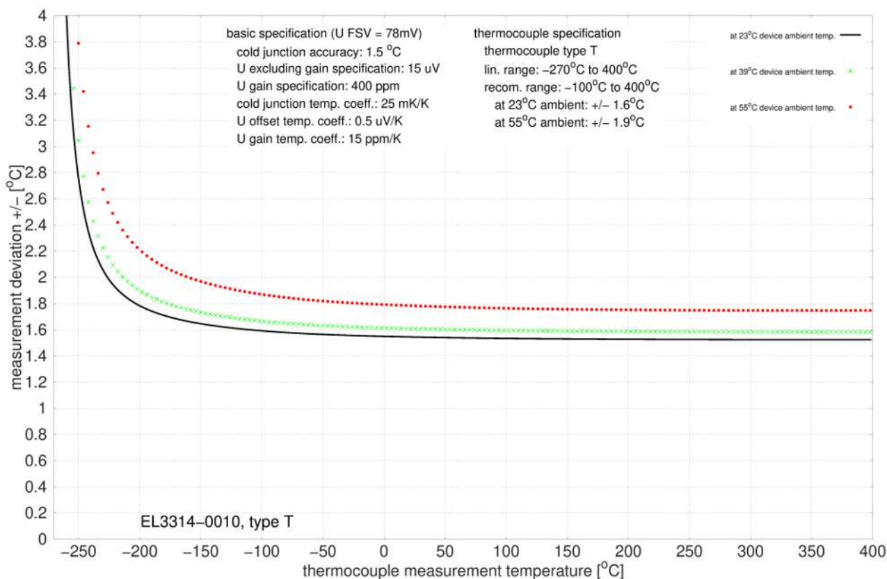
附图 33: EL3314-0010、EL3314-0020 和 EL3314-0030 (等同于 EL3314-0010) , T 型
