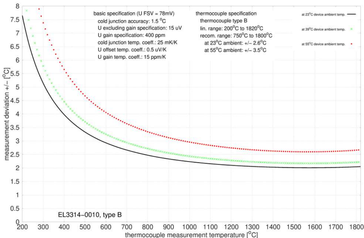
附图 37: EL3314-0010、EL3314-0020 和 EL3314-0030 (等同于 EL3314-0010) , B 型
