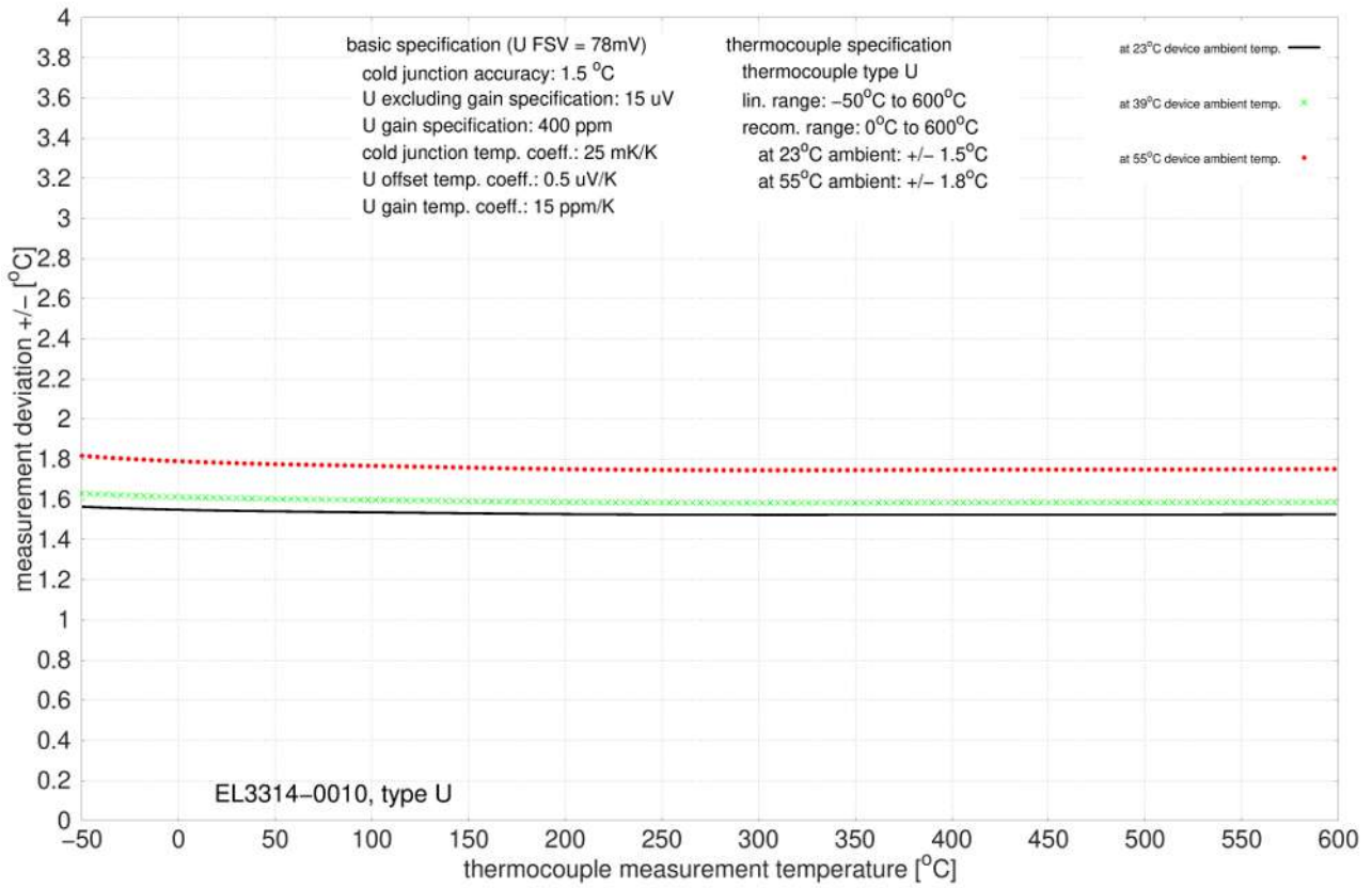
附图 47: EL3314-0010、EL3314-0020 和 EL3314-0030 (等同于 EL3314-0010) , U 型
