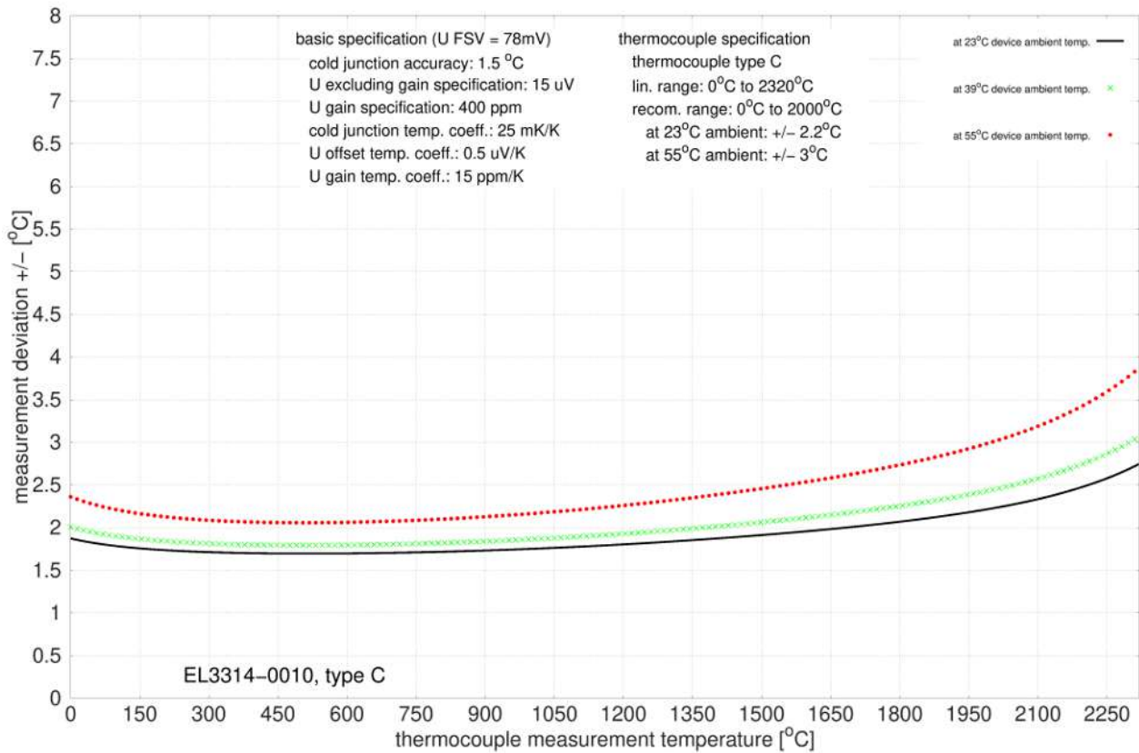
附图 51: EL3314-0010、EL3314-0020 和 EL3314-0030（等同于 EL3314-0010），C 型
