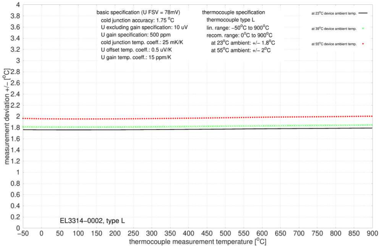
附图 16: EL3314-0002 和 EL3314-0092 (对应 EL3314-0002), L 型
