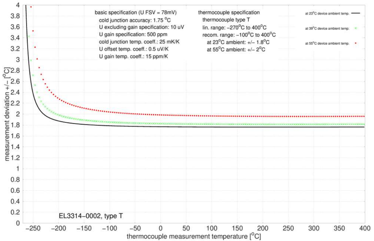
附图 20: EL3314-0002 和 EL3314-0092 (对应 EL3314-0002), T 型
