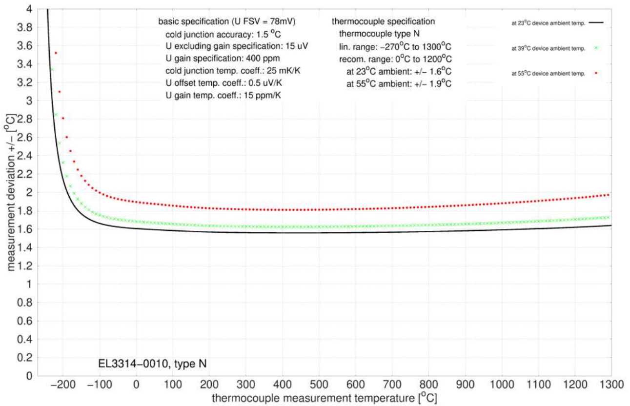
附图 30: EL3314-0010、EL3314-0020 和 EL3314-0030（等同于 EL3314-0010），N 型
