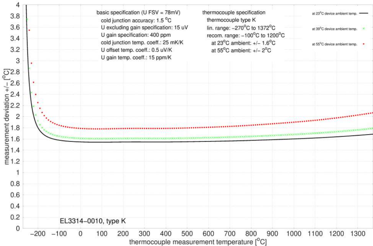
附图 41: EL3314-0010、EL3314-0020 和 EL3314-0030 (相当于 EL3314-0010) , K 型
