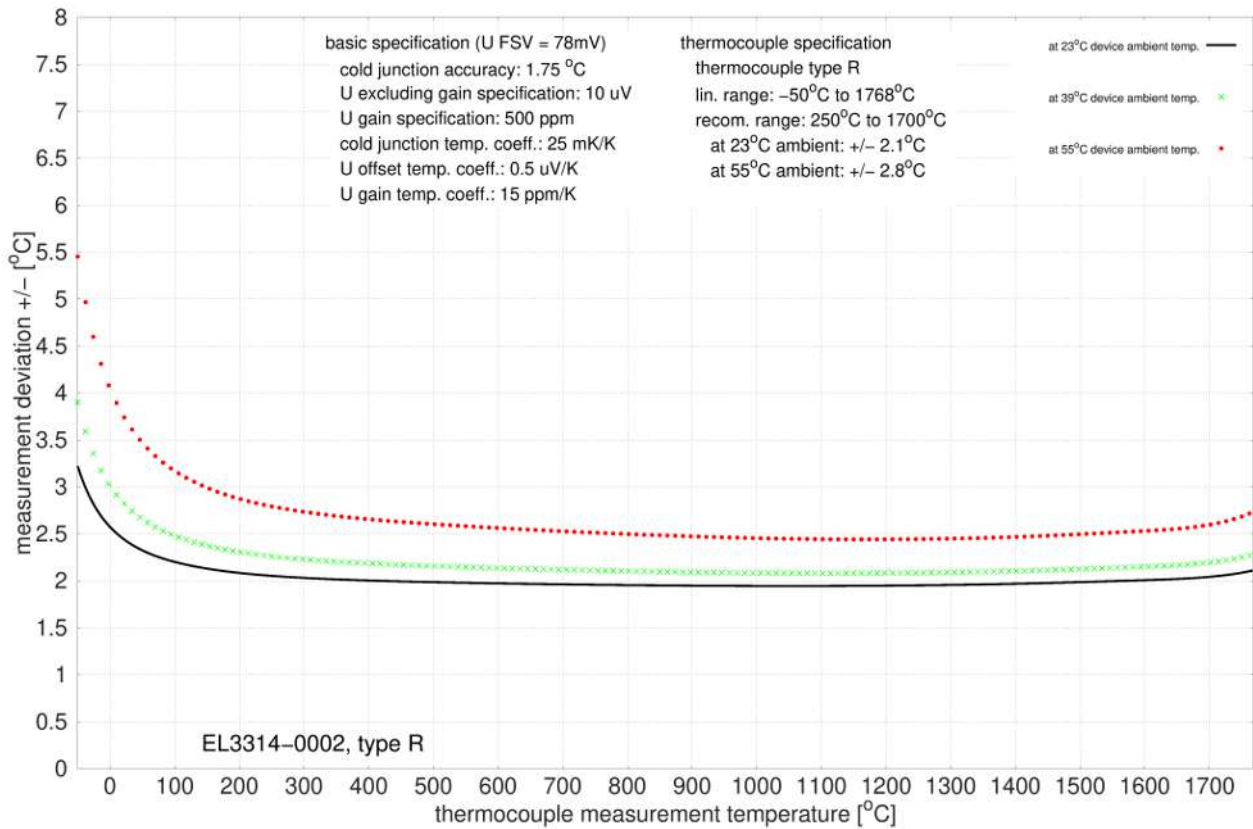
附图 72: EL3314-0002 和 EL3314-0092 (对应 EL3314-0002), R 型
