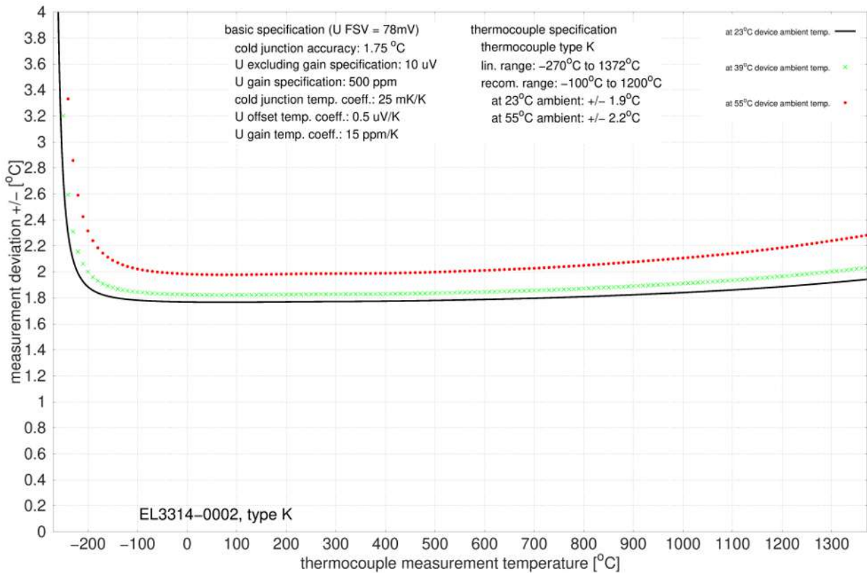
附图 15: EL3314-0002 和 EL3314-0092 (对应 EL3314-0002), K 型
