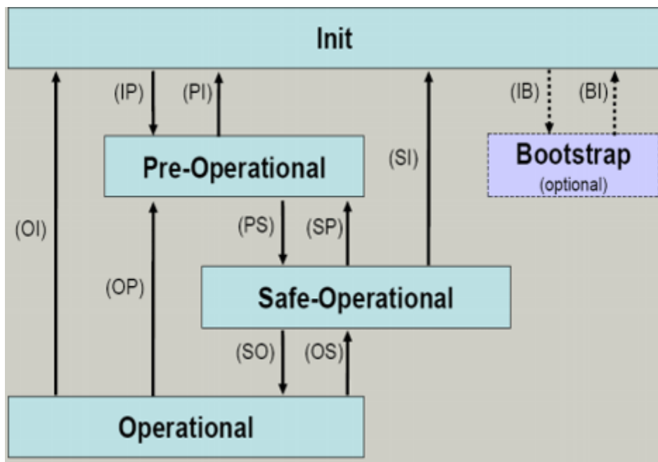
附图 84: EtherCAT 状态机的状态
