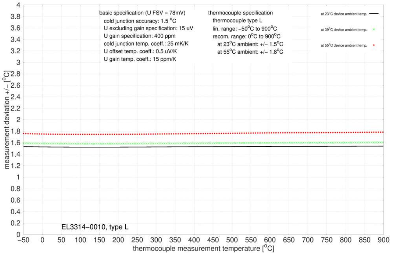
附图 29: EL3314-0010、EL3314-0020 和 EL3314-0030 (等同于 EL3314-0010), L 型
