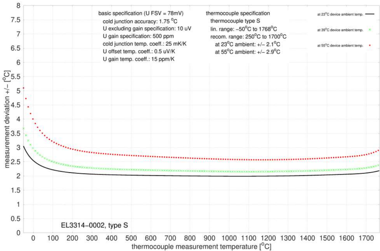
附图 19: EL3314-0002 和 EL3314-0092 (对应 EL3314-0002), S 型
