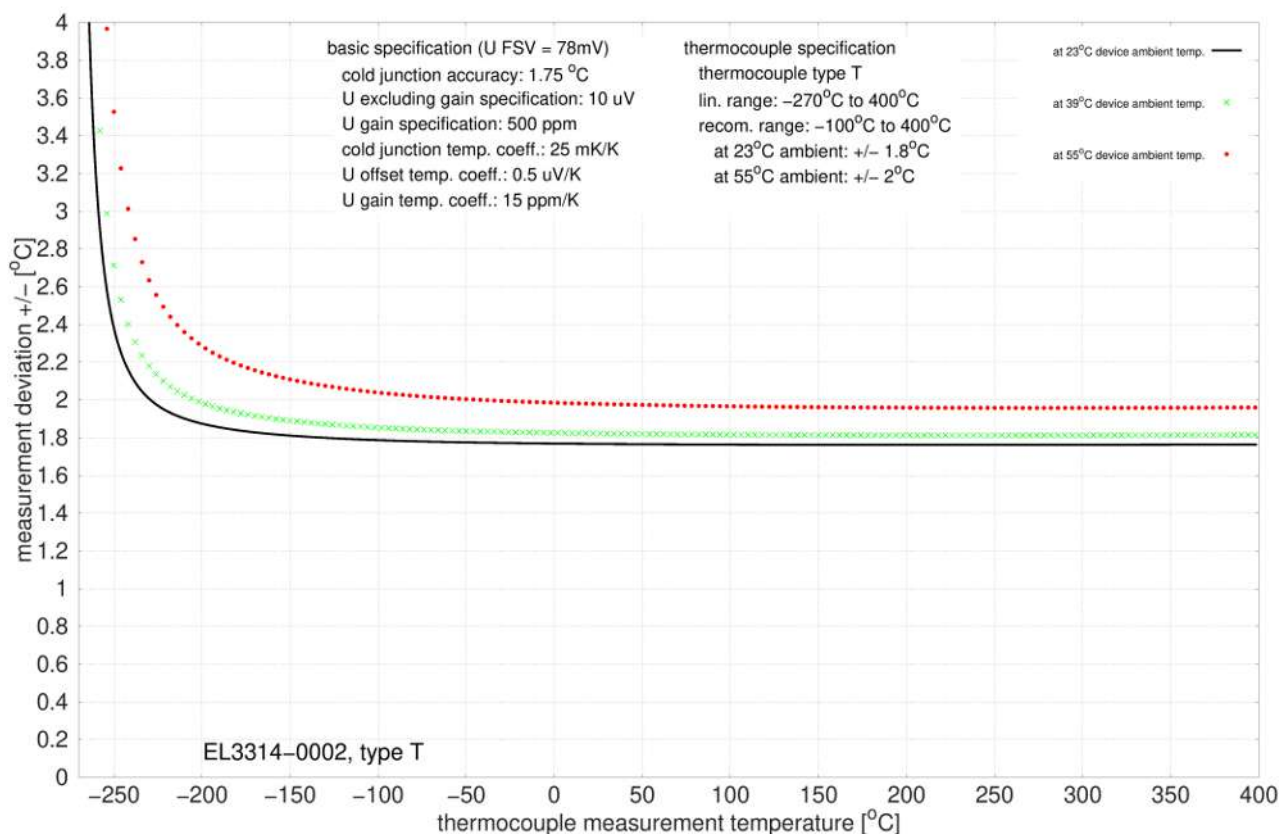
附图 74: EL3314-0002 和 EL3314-0092 (对应 EL3314-0002), T 型
