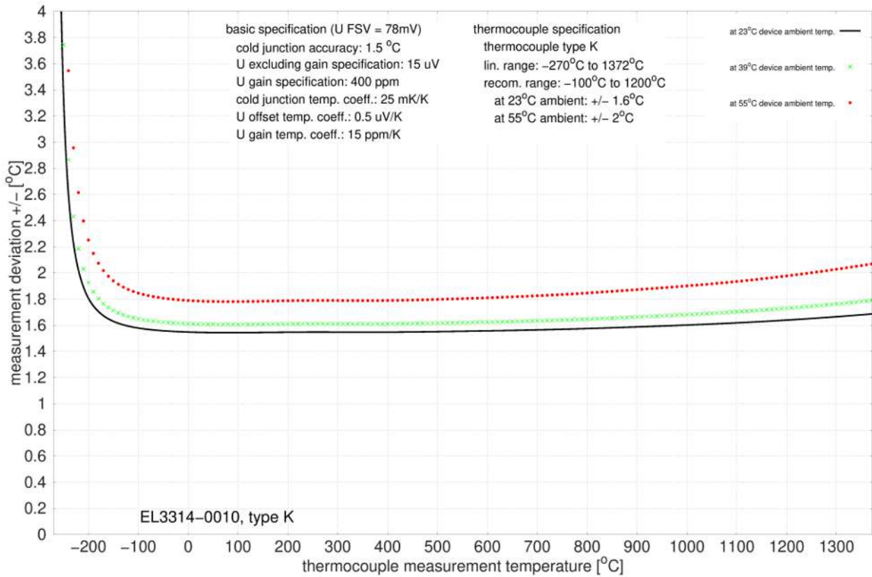
附图 28: EL3314-0010、EL3314-0020 和 EL3314-0030 (相当于 EL3314-0010) , K 型
