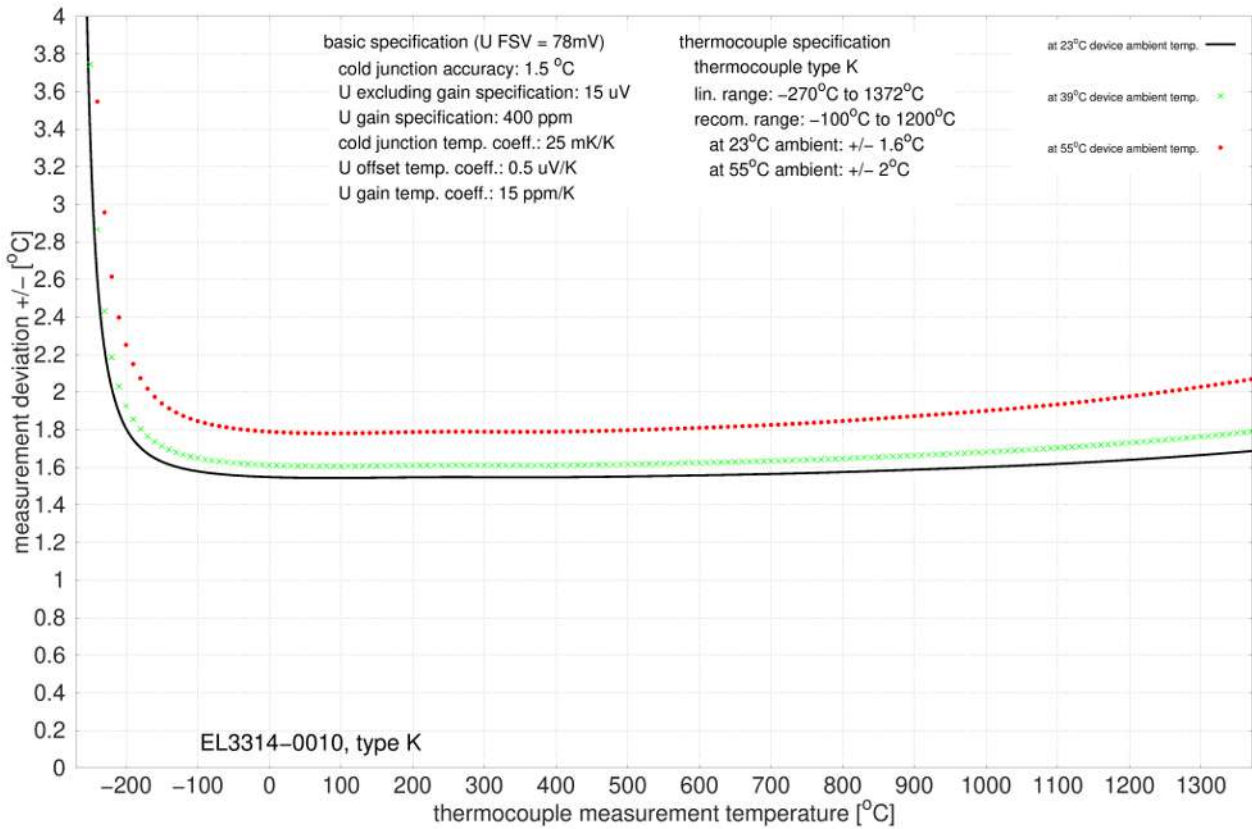
附图 54: EL3314-0010、EL3314-0020 和 EL3314-0030（相当于 EL3314-0010），K 型
