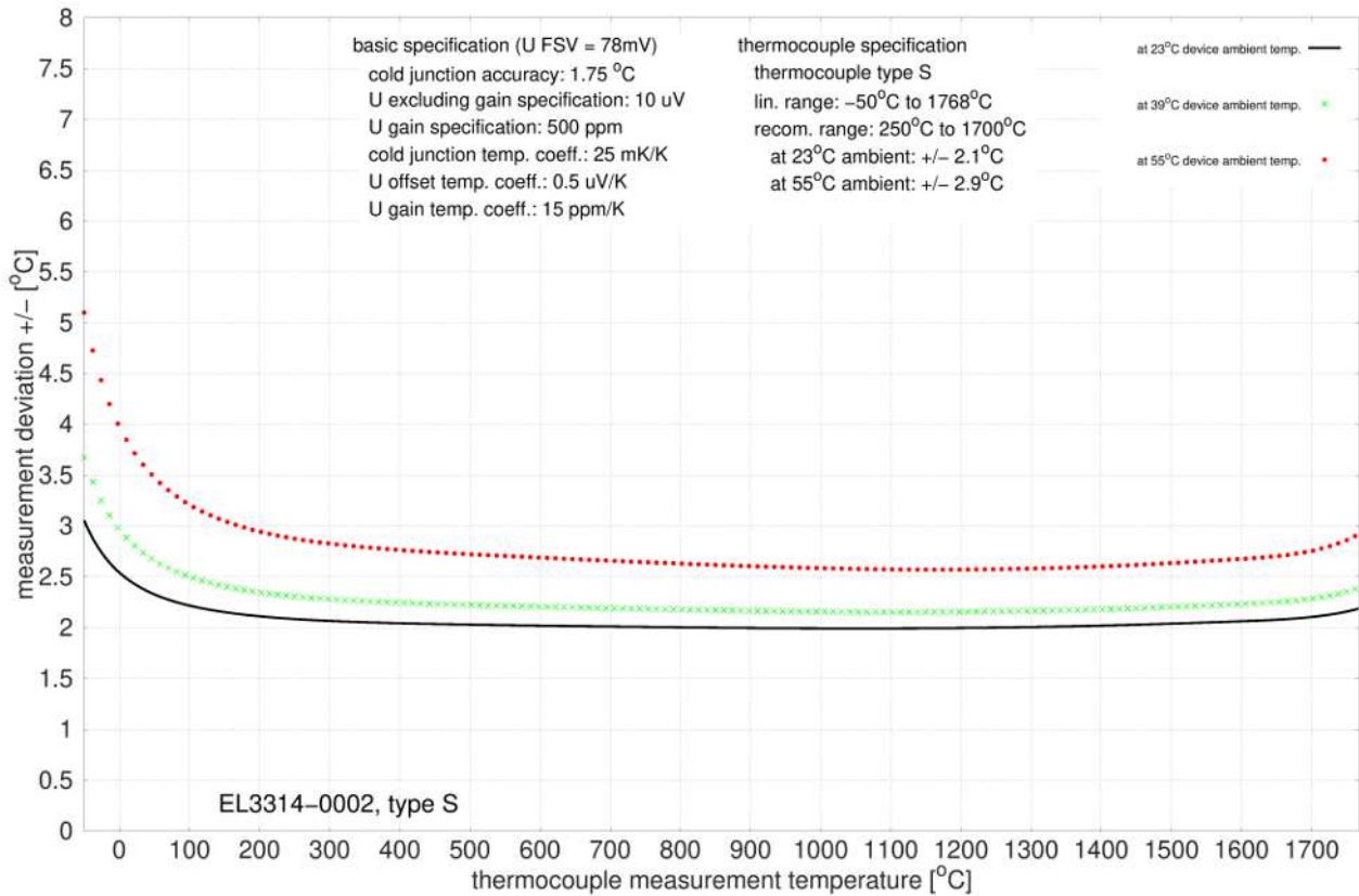
附图 73: EL3314-0002 和 EL3314-0092 (对应 EL3314-0002), S 型
