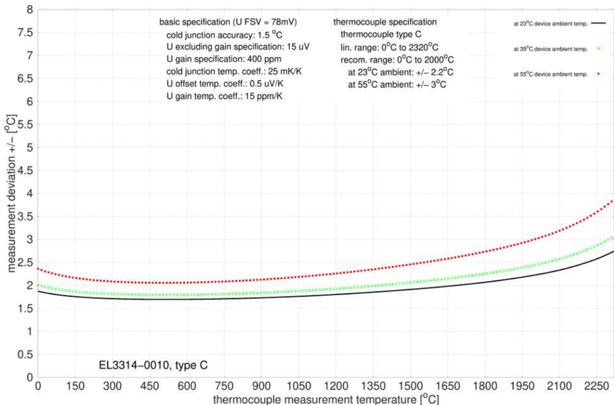
附图 25: EL3314-0010、EL3314-0020 和 EL3314-0030（等同于 EL3314-0010），C 型
