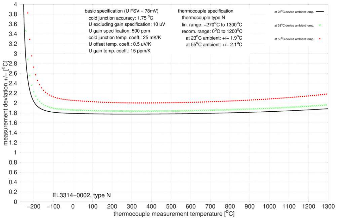
附图 71: EL3314-0002 和 EL3314-0092 (对应 EL3314-0002), N 型
