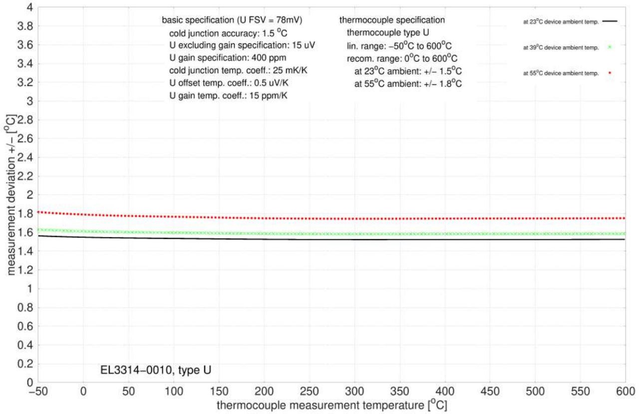
附图 34: EL3314-0010、EL3314-0020 和 EL3314-0030 (等同于 EL3314-0010), U 型
