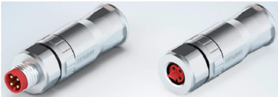
Abb. 35: EtherCAT P: Feldkonfektionierbare Steckverbinder
