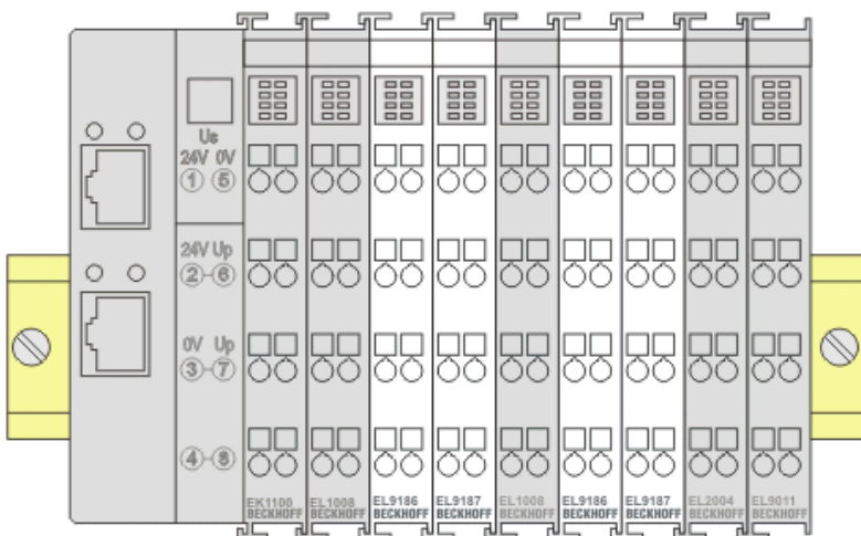
Abb. 26: Korrekte Positionierung
