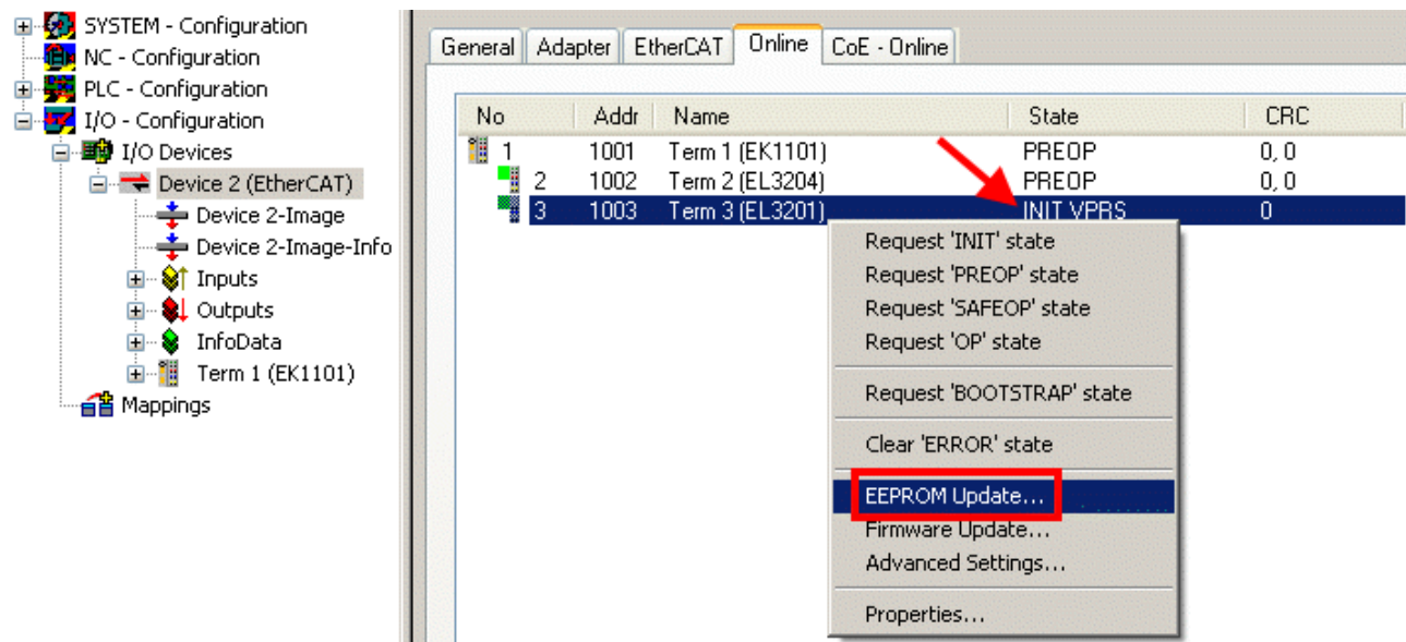
Abb. 52: EEPROM Update
