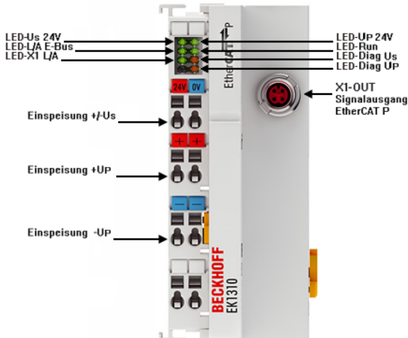
Abb. 28: EK1310 Anschlüsse Einspeisung
