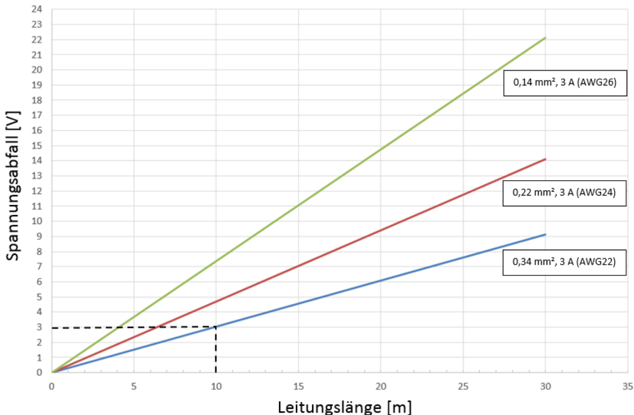
Abb. 37: Leitungsverluste auf den EtherCAT-P-Kabeln
