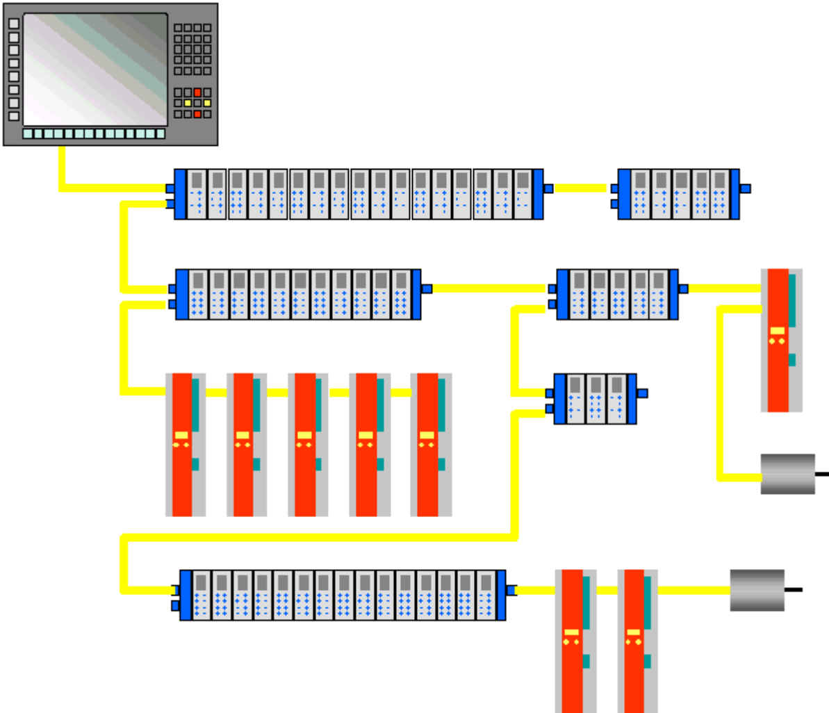
Abb. 12: EtherCAT Topologie
