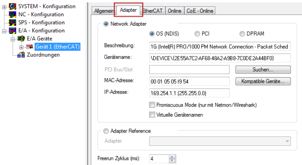
Abb. 54: Eigenschaften EtherCAT-Gerät (TwinCAT 2)
