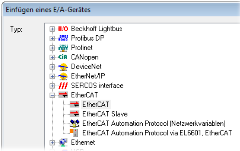
Abb. 52: Auswahl EtherCAT Anschluss (TwinCAT 2.11, TwinCAT 3)
