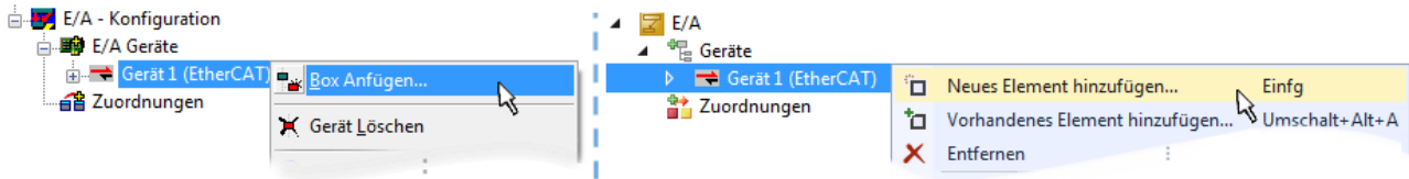
Abb. 55: Anfügen von EtherCAT-Geräten (links: TwinCAT 2; rechts: TwinCAT 3)
