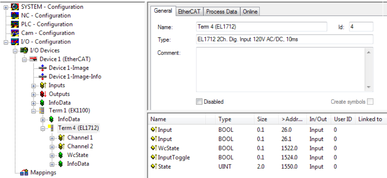
Abb. 12: EL1712 im TwinCAT-Baum
