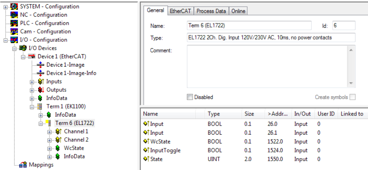
Abb. 18: EL1722 im TwinCAT-Baum
