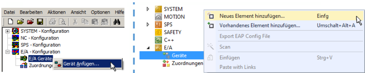
Abb. 51: Anfügen eines EtherCAT Device: links TwinCAT 2; rechts TwinCAT 3
