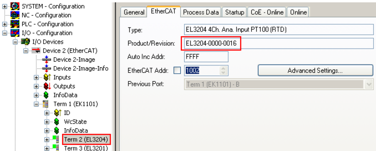
Abb. 96: Geräteerkennung aus Name EL3204-0000 und Revision -0016
