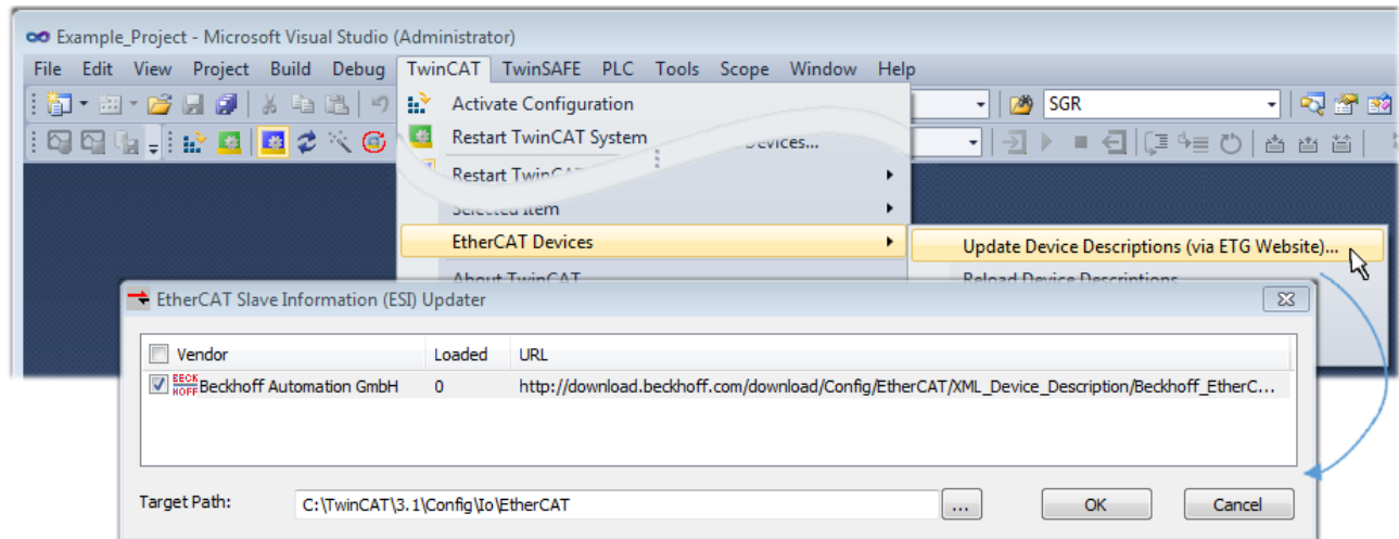
Abb. 50: Anwendung des ESI Updater (TwinCAT 3)
