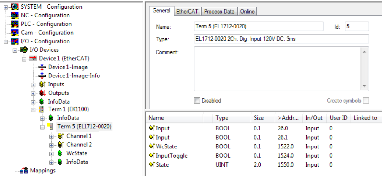
Abb. 15: EL1712-0020 im TwinCAT-Baum
