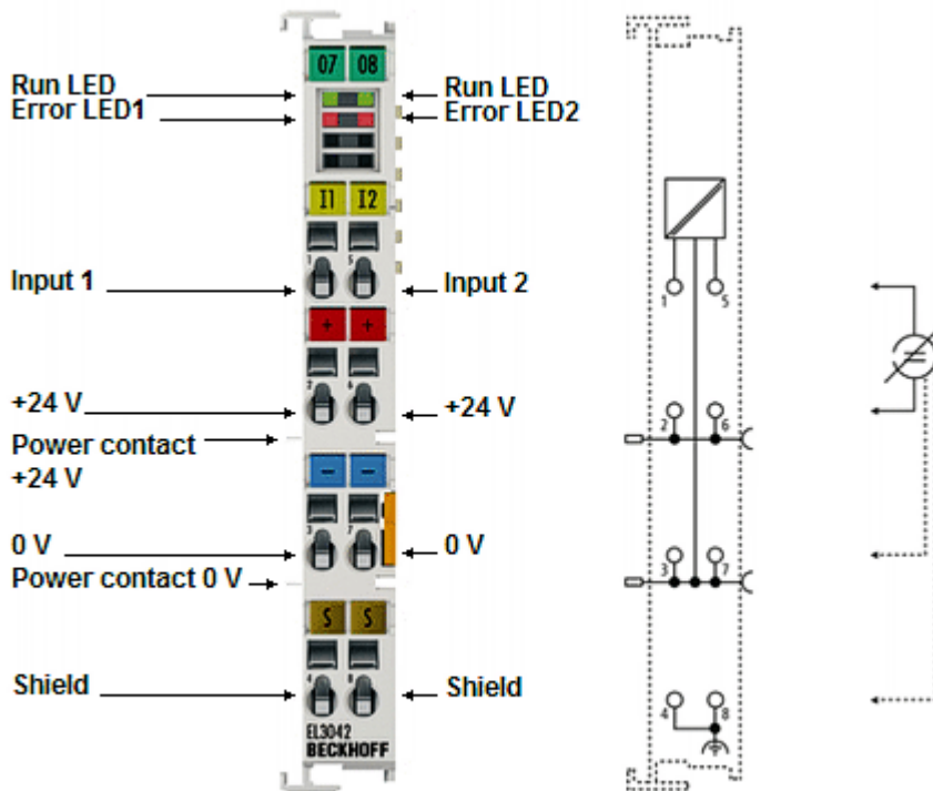
Fig. 26: EL3042
