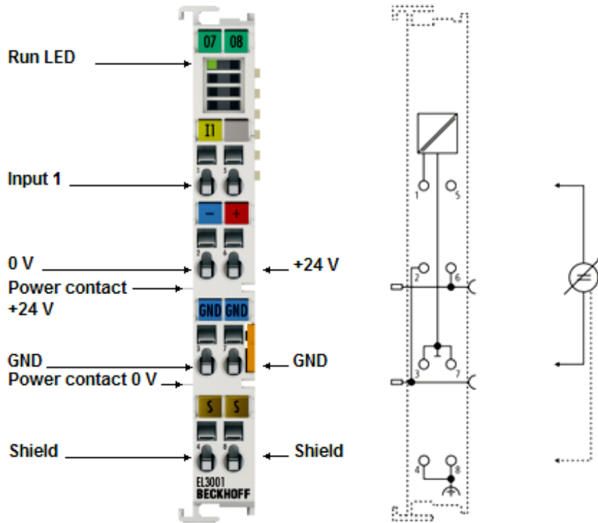
Fig. 4: EL3001
