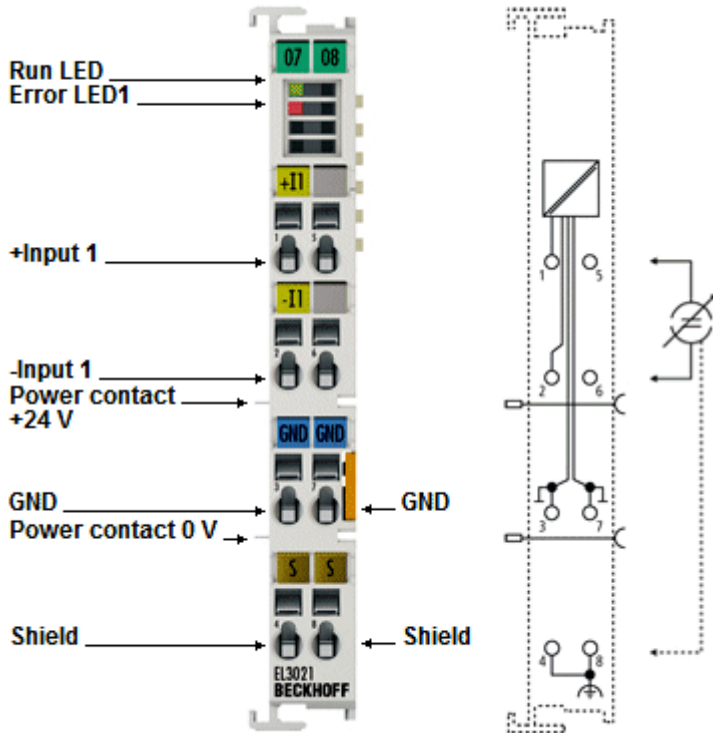
Fig. 18: EL3021
