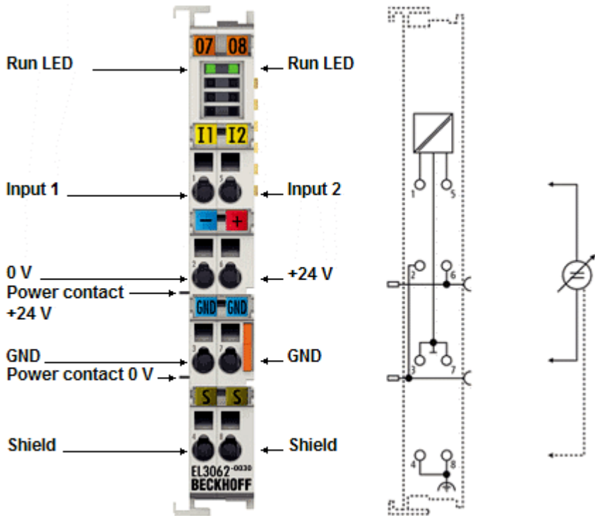
Fig. 44: EL3062-0030
