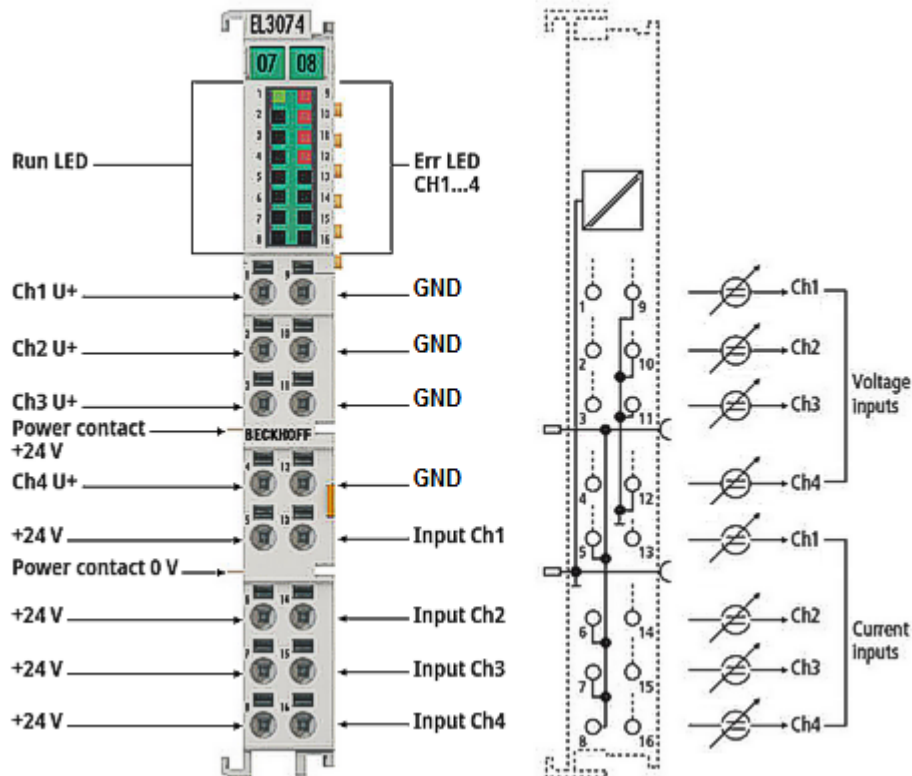
Fig. 52: EL3074
