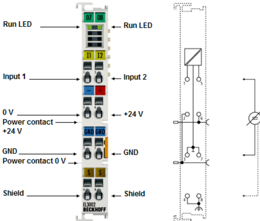
Fig. 6: EL3002
