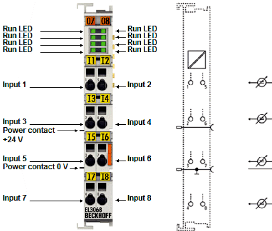
Fig. 48: EL3068
