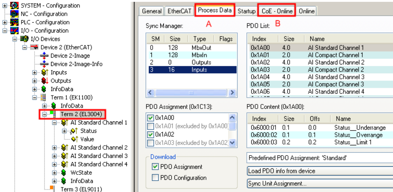
Fig. 182: EL30xx parameterization
