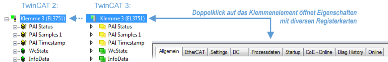
Abb. 131: „Baumzweig“ Element als Klemme EL3751
