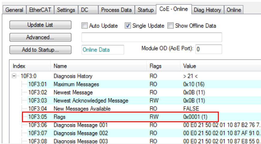
Abb. 179: Aktivierung/Deaktivierung Event-Absetzung
