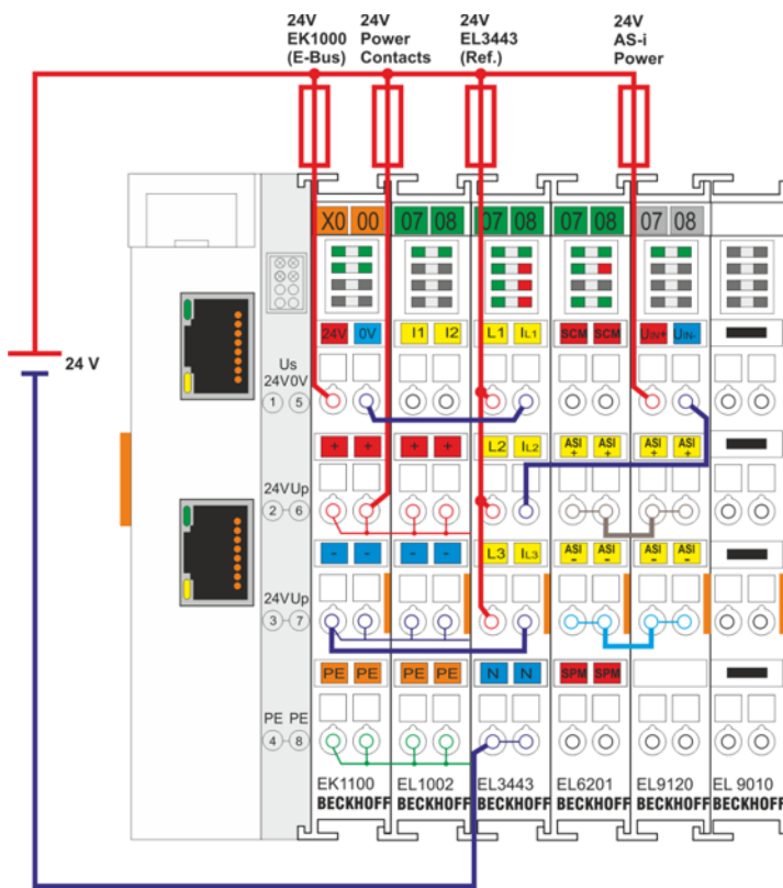
附图 159：应用示例 - 现场总线 I/O 站的电力测量
