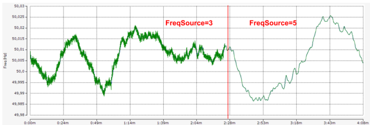
附图 153：设置 Index F800:13； [▶ 229] 左侧，无 PT2 滤波（FreqSource = 3）；右侧，有 PT2 滤波（FreqSource = 5）
