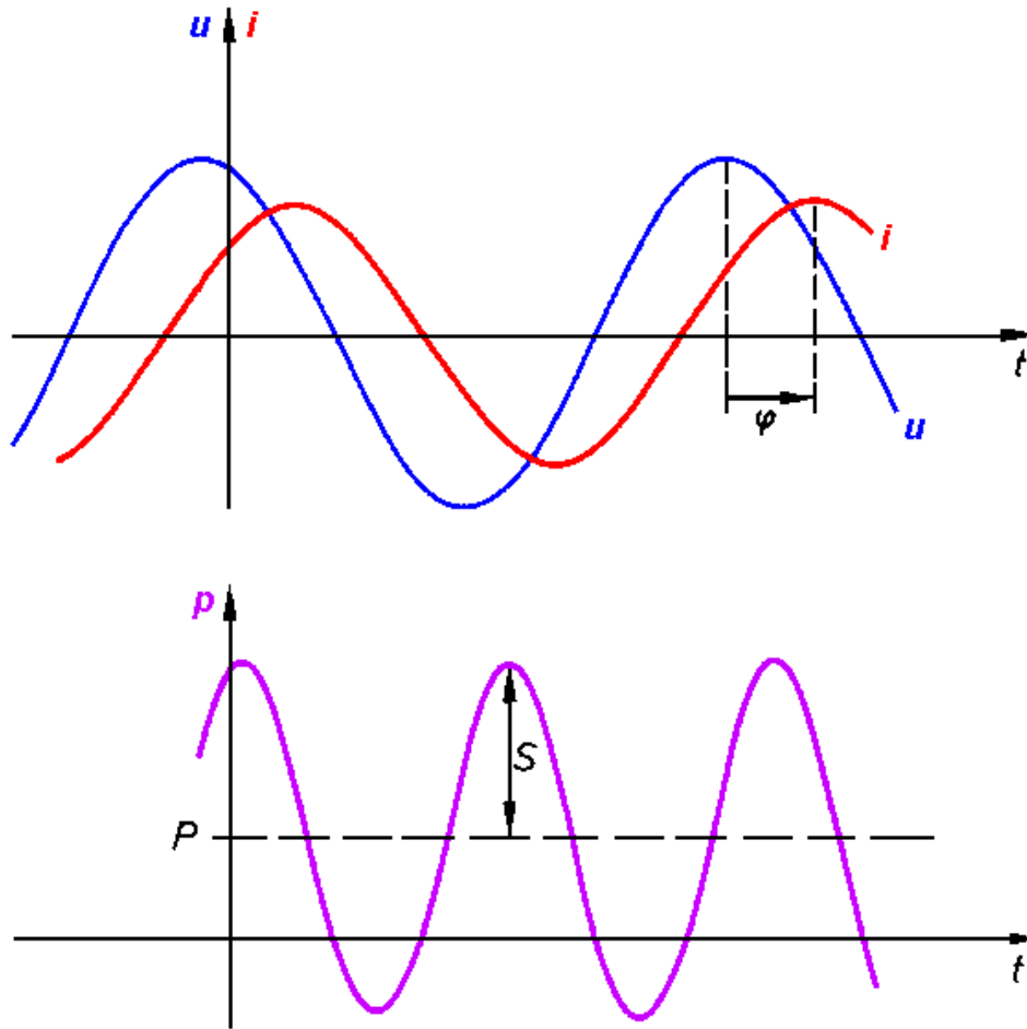
附图 16: 有相位角 \varphi 的 u 、 i 、 p 时间关系曲线
