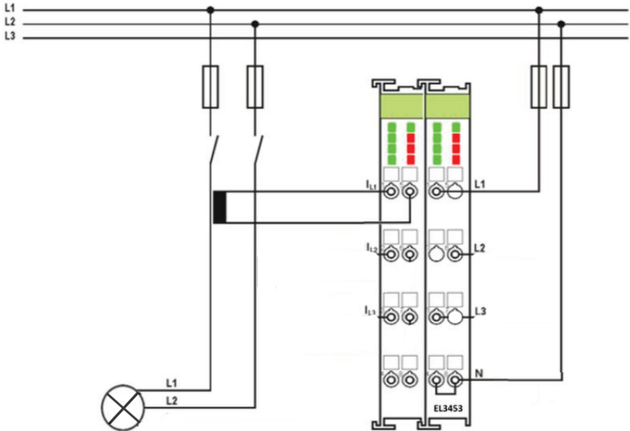
附图 162: EL3453 - 用于测量相间电压的接线
