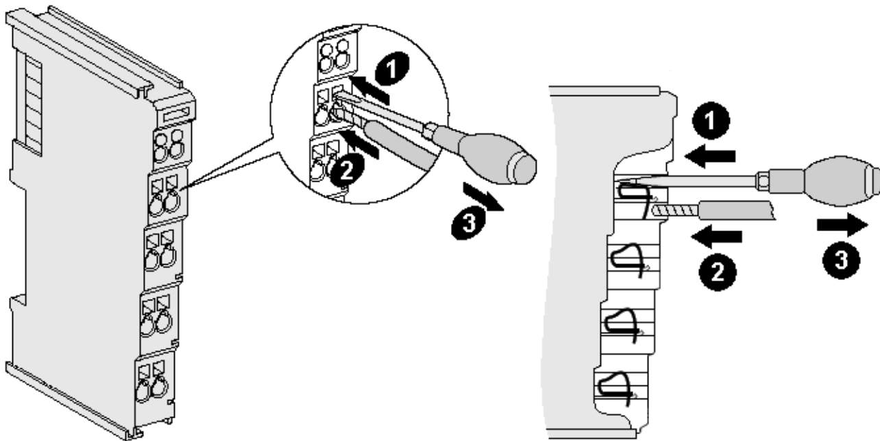
附图 58：在一个接线点上连接线缆
