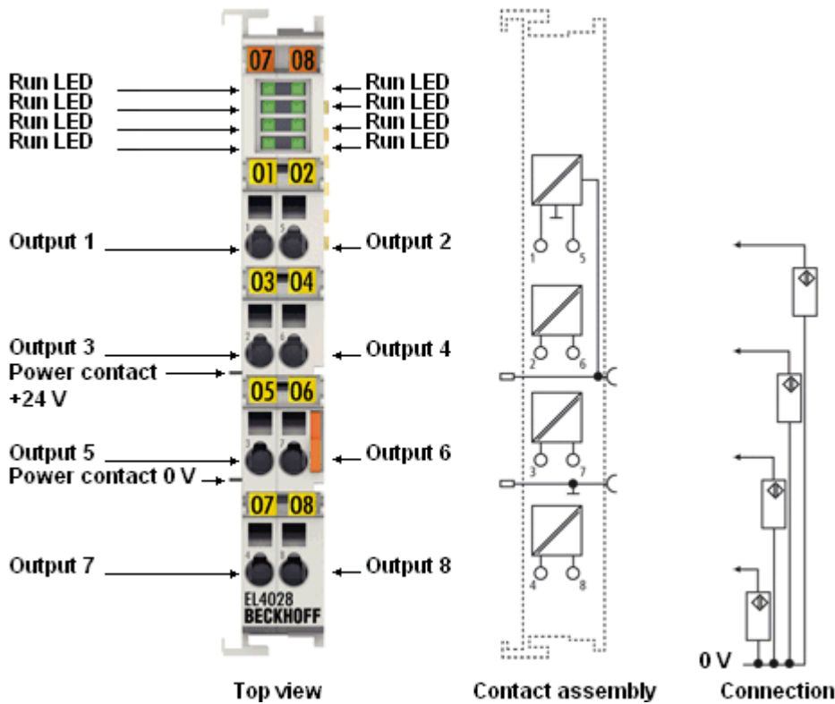
附图 33: EL4028, 连接和显示
