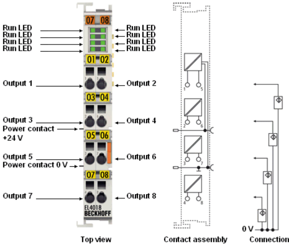
附图 23: EL4018, 连接和显示
