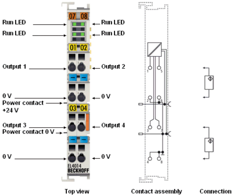
附图 22: EL4014, 连接和显示
