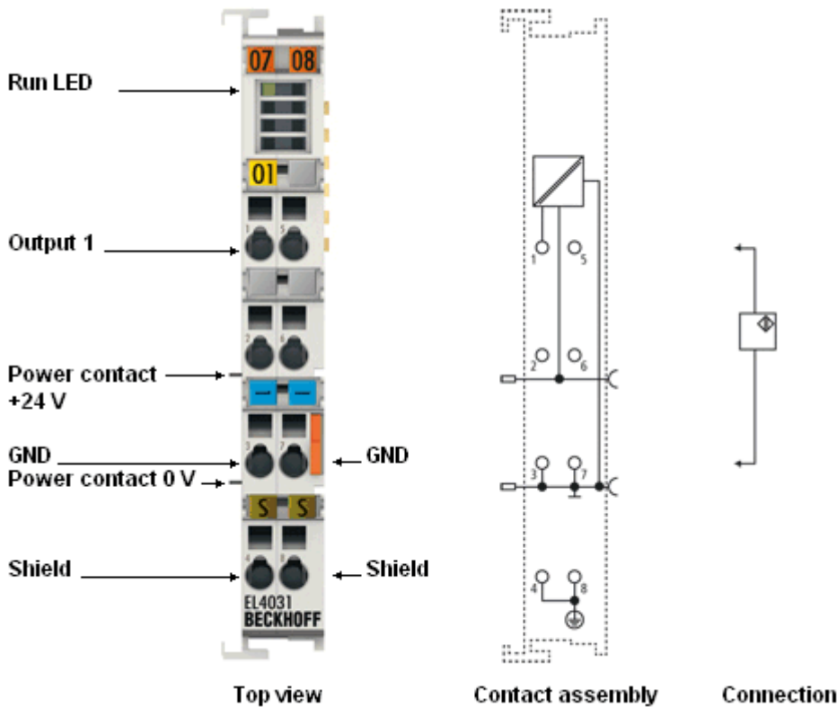
附图 38: EL4031, 连接和显示
