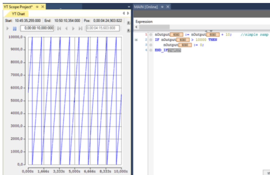
附图 175: 模拟值输出，以电压斜坡为例
