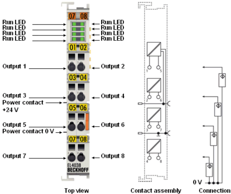
附图 43: EL4038, 连接和显示
