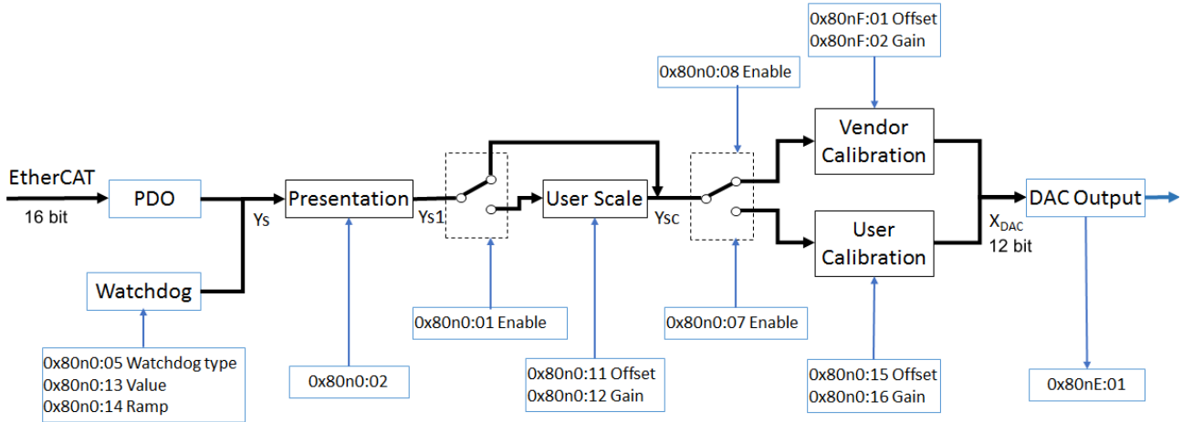
附图 179: 计算输出值的框图
