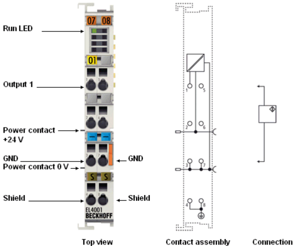
附图 8: EL4001, 连接和显示
