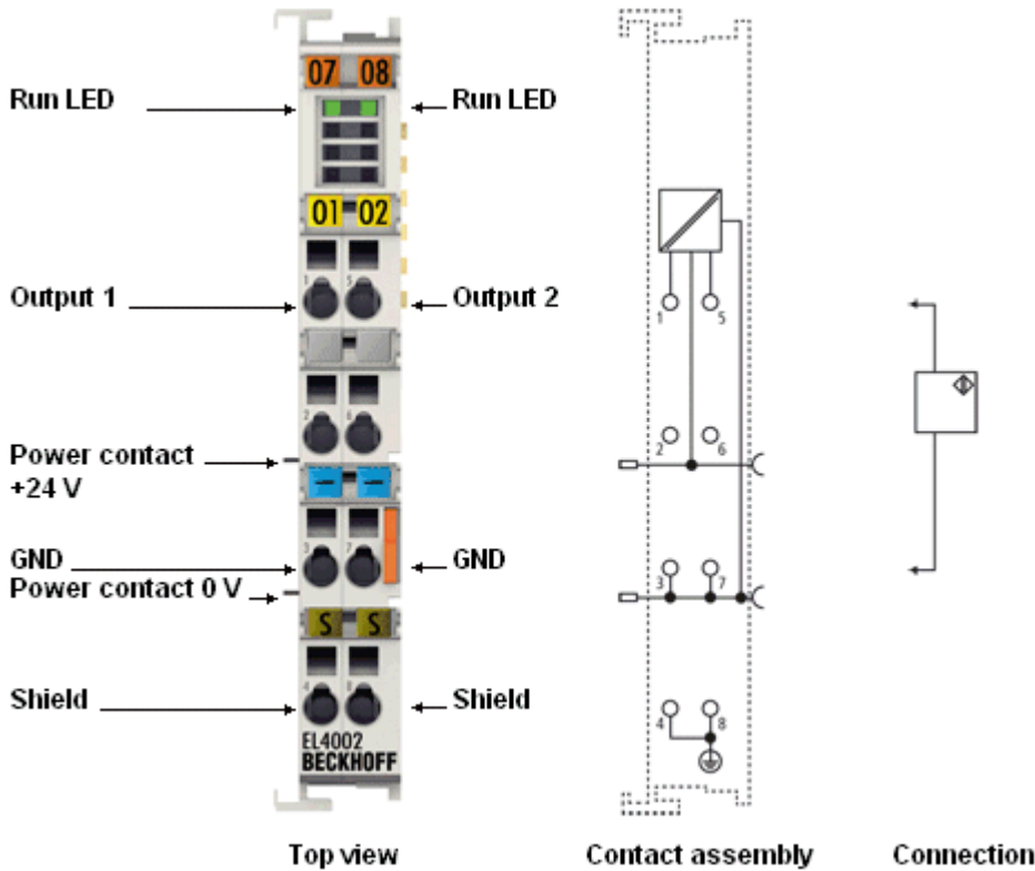
附图 10: EL4002, 连接和显示
