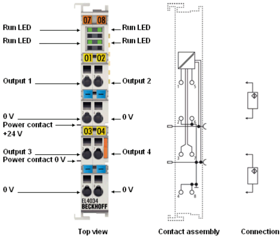
附图 42: EL4034, 连接和显示
