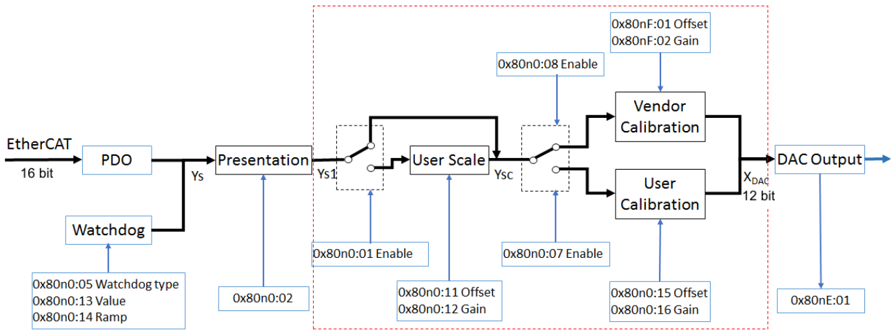
附图 181: 确定默认输出值的框图 (增益/偏移功能)
