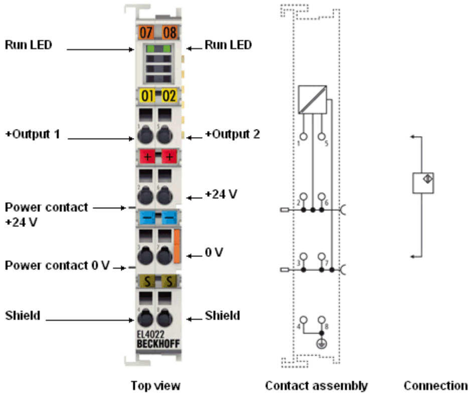
附图 30: EL4022, 连接和显示
