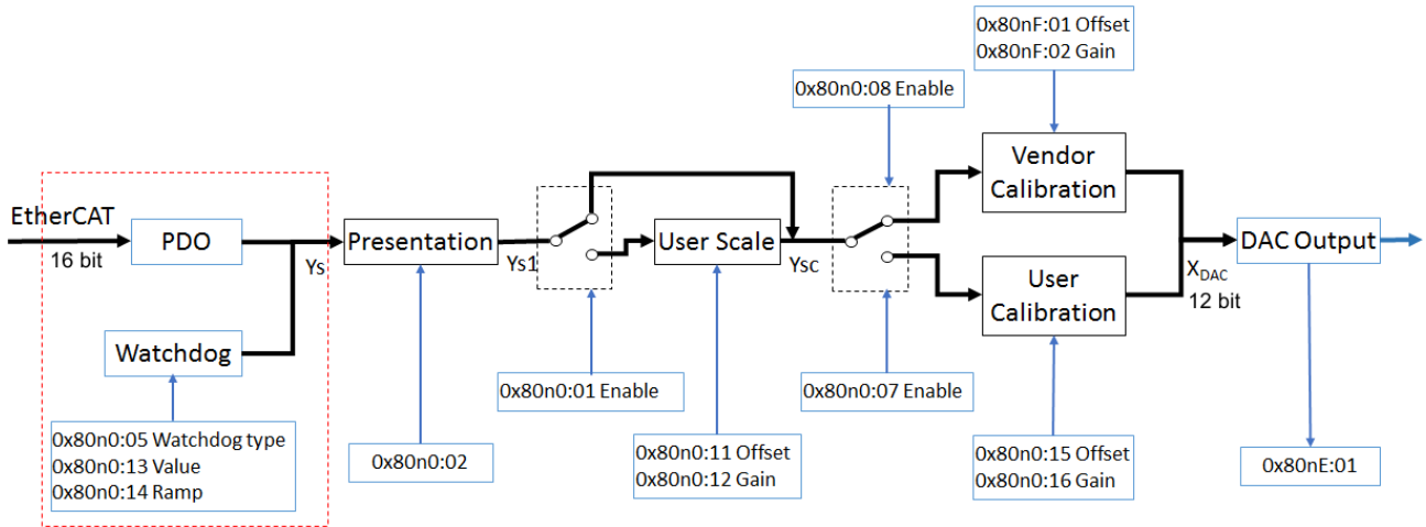
附图 182: 确定输出值的框图 (看门狗功能)
