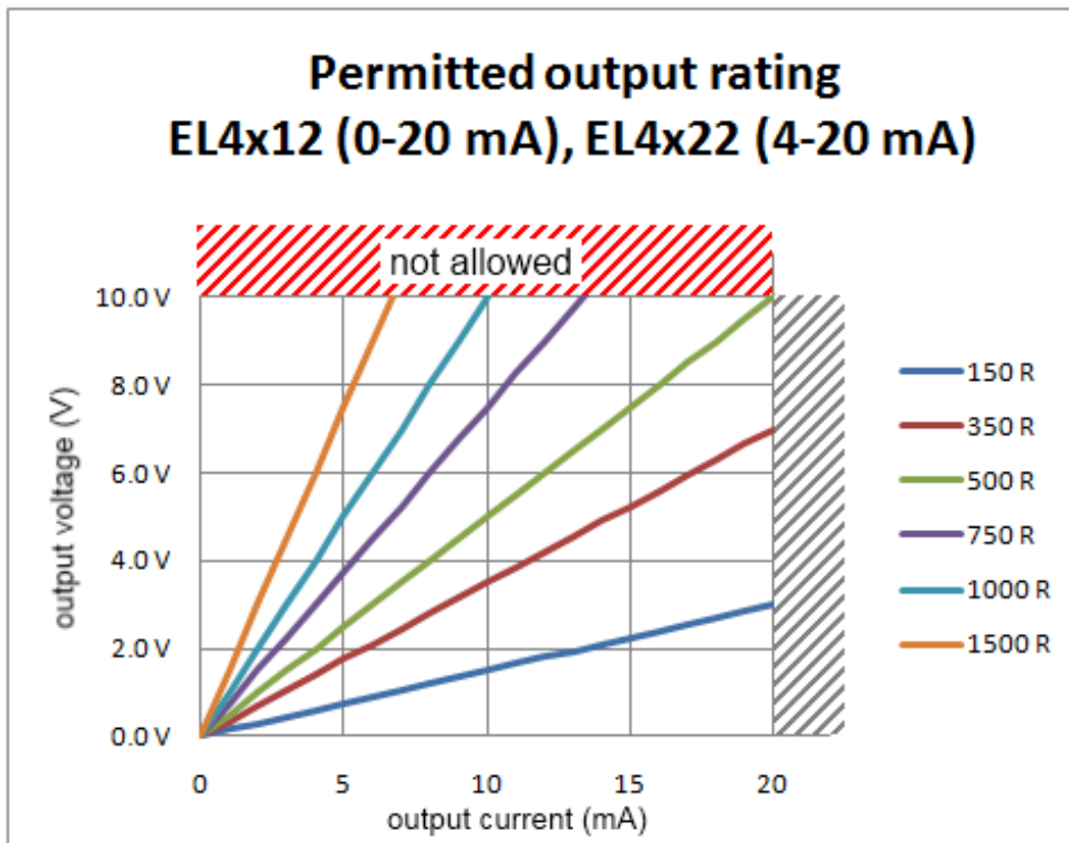
附图 184: EL4xx2 电流输出允许的操作范围
