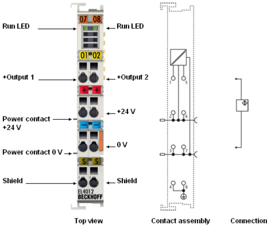
附图 20: EL4012, 连接和显示
