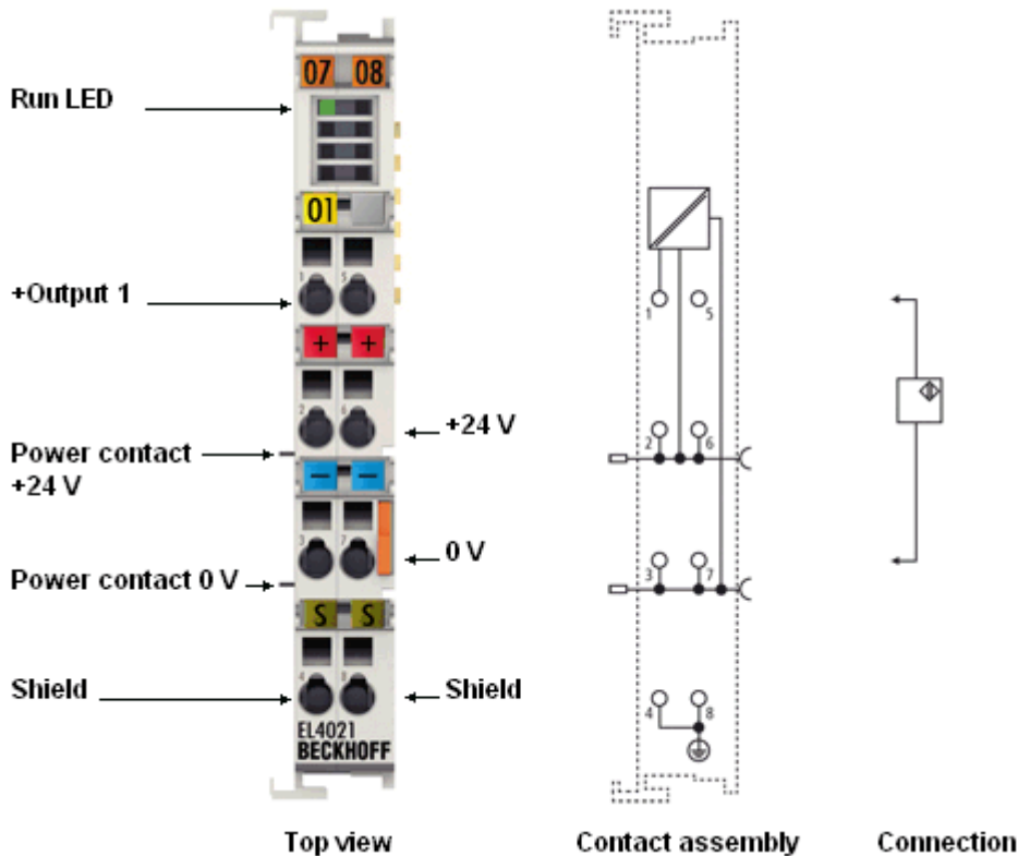
附图 28: EL4021, 连接和显示
