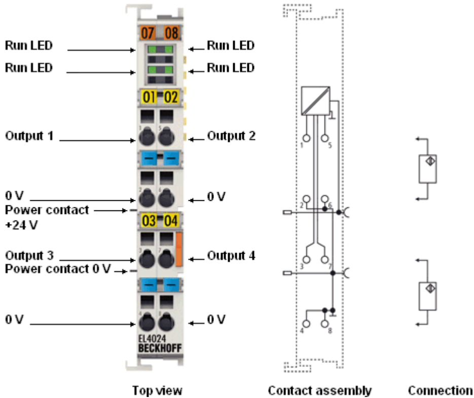
附图 32: EL4024, 连接和显示
