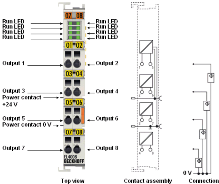
附图 13: EL4008, 连接和显示
