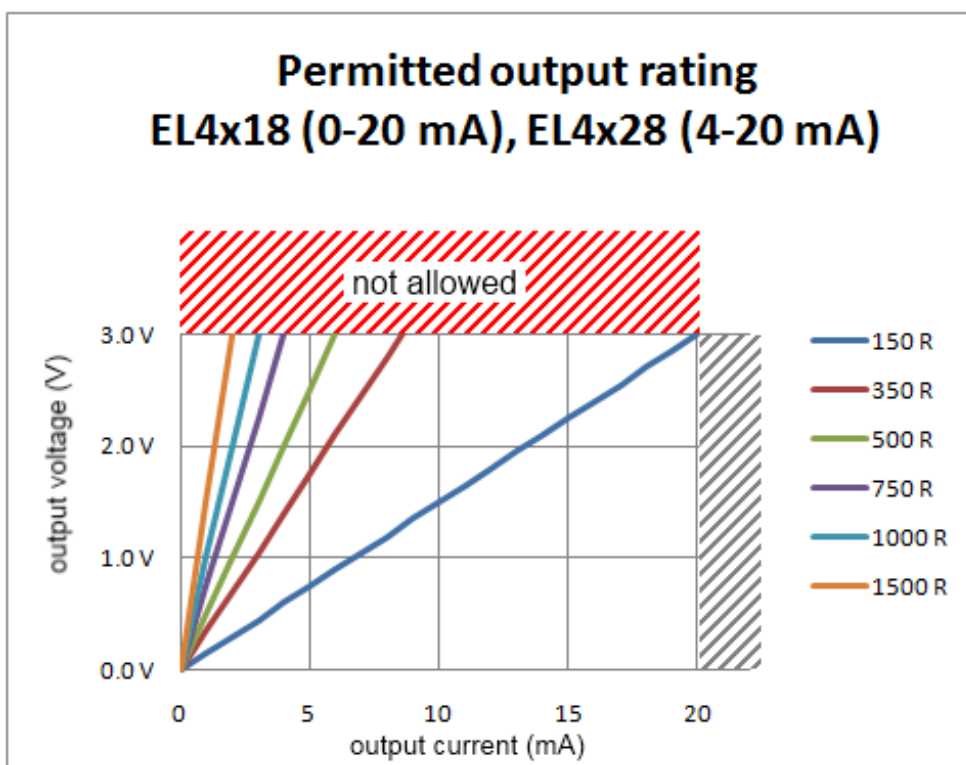
附图 186: EL4xx8 电流输出允许的操作范围
