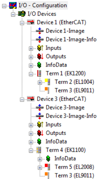
附图 70: TwinCAT 2 System Manager 中的配置映射
