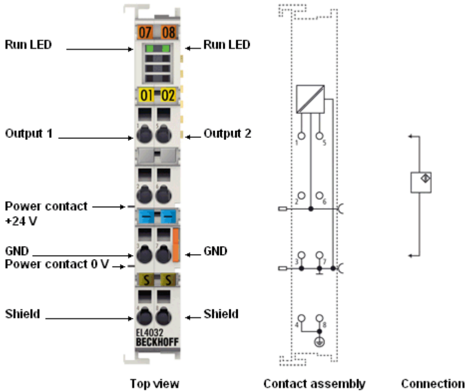
附图 40: EL4032, 连接和显示
