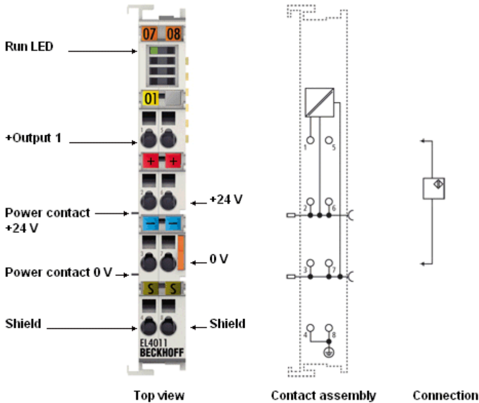
附图 18: EL4011, 连接和显示
