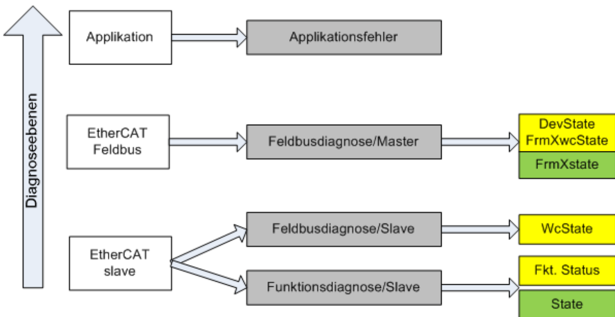
Abb. 95: Auswahl an Diagnoseinformationen eines EtherCAT Slave
