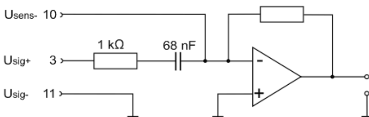
Abb. 35: Prinzipschaltbild Eingangsimpedanz Mahr® (Kanal 1)
