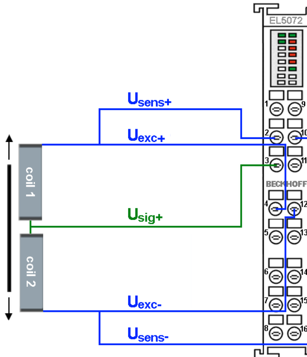
Abb. 32: Anschlussbelegung 5-Leiter induktive Halbrücke
