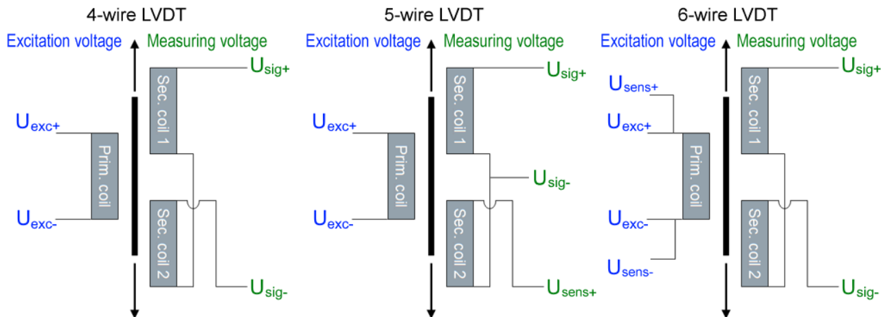
Abb. 6: LVDT - Funktionsprinzip
