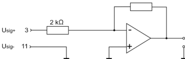
Abb. 34: Prinzipschaltbild Eingangsimpedanz Tesa® (Kanal 1)
