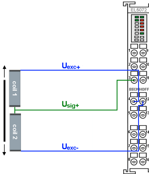
Abb. 31: Anschlussbelegung 3-Leiter induktive Halbrücke
