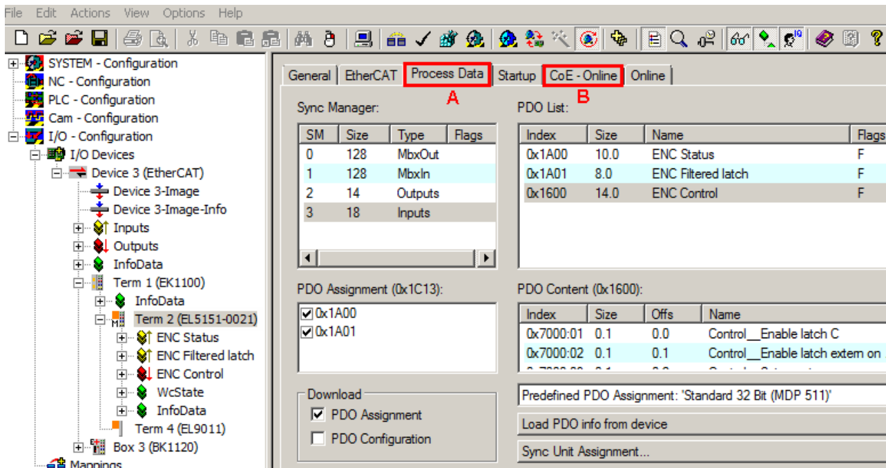
Abb. 151: Parametrierung EL5151-0021
