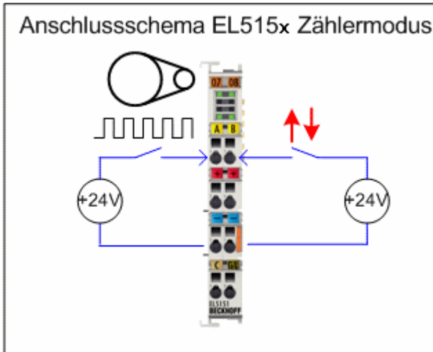
Abb. 154: Prinzip Zähleranschluss
