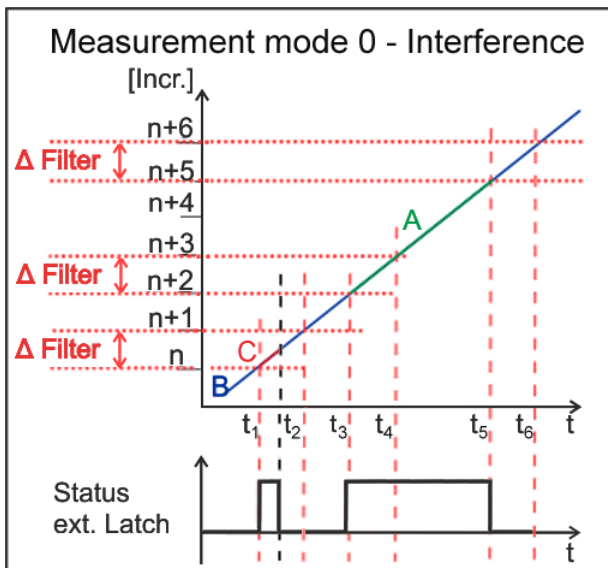
Abb. 156: Graphische Darstellung Messung in Modus 0 - Signalstörung
