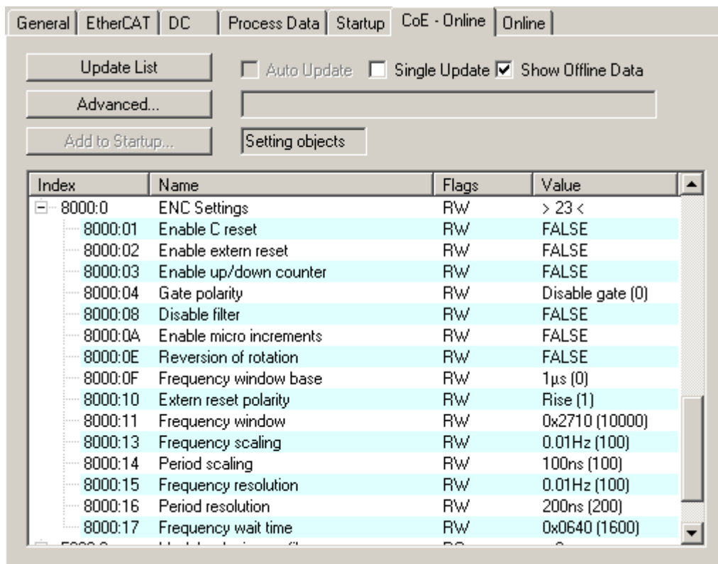
Abb. 145: Reiter „CoE - Online“, EL5151
