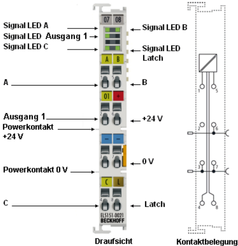
Abb. 30: EL5151-0021 - LEDs und Anschlussbelegung
