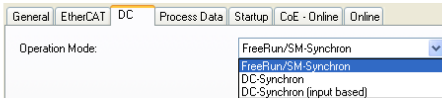
Abb. 142: Reiter DC
