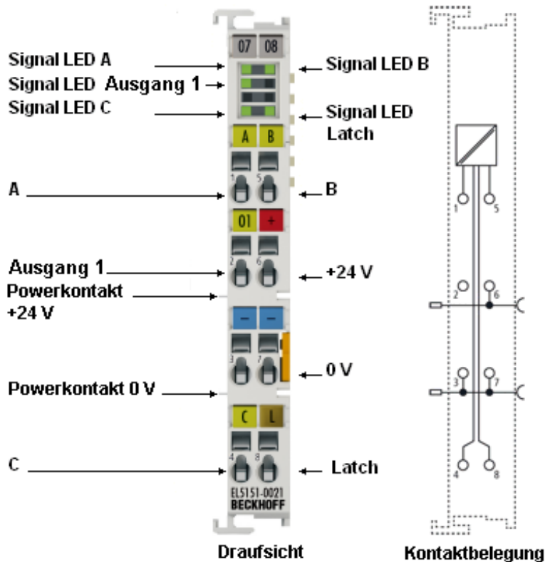
Abb. 5: EL5151-0021
