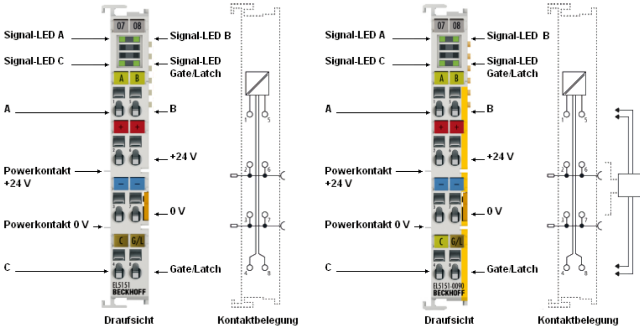
Abb. 29: EL5151, EL5151-0090 - LEDs und Anschlussbelegung
