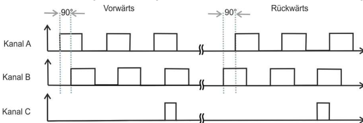
Abb. 8: Quadraturdecoder
