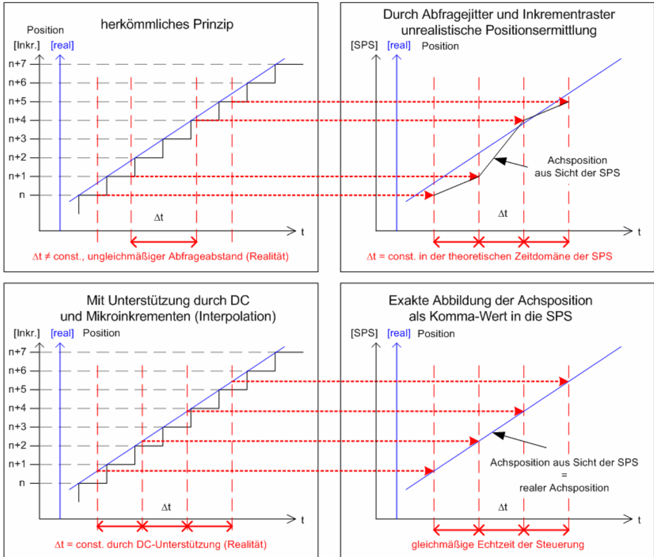
Abb. 150: Prinzip Frequenzmessung
