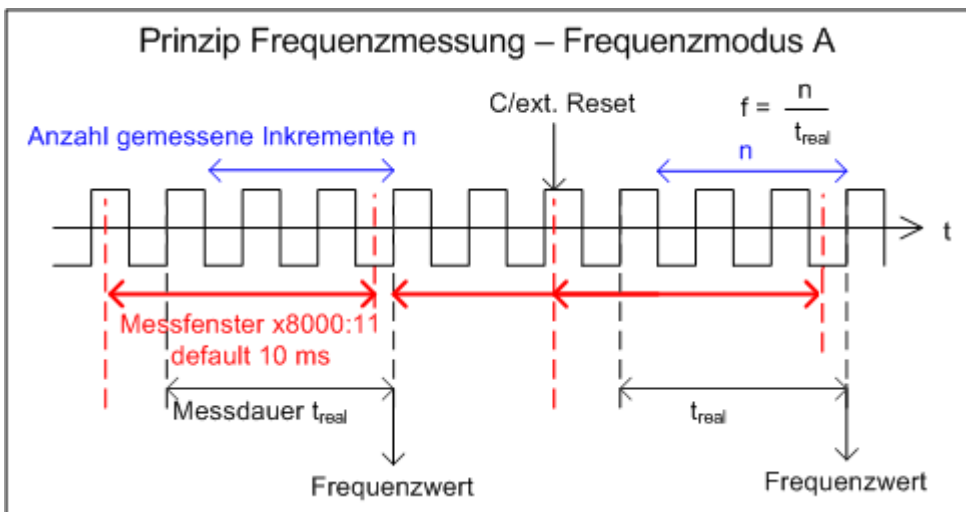
Abb. 147: Prinzip Frequenzmessung - Frequenzmodus A
