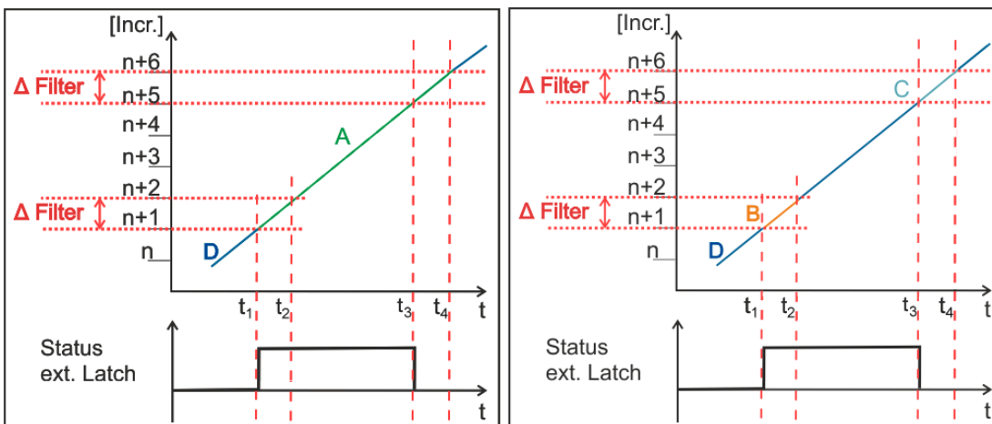
Abb. 155: Graphische Darstellung der Messung
