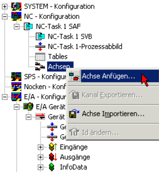
Abb. 169: Achse einfügen
