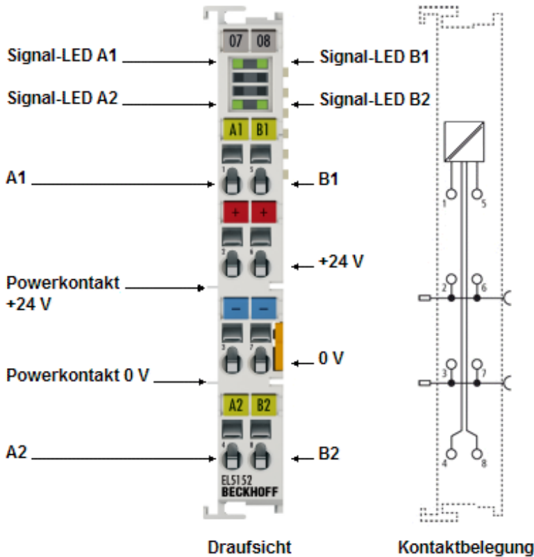
Abb. 31: EL5152 - LEDs und Anschlussbelegung
