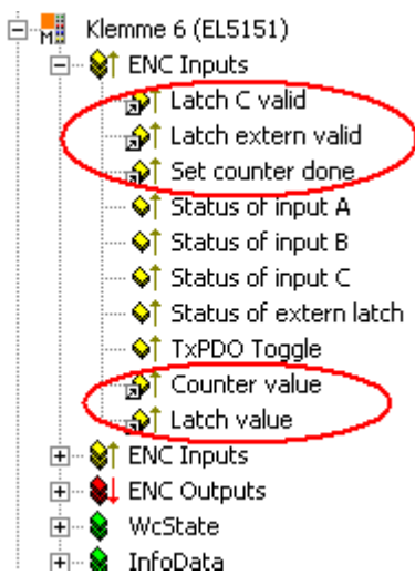
Abb. 173: Verknüpfte Eingänge der EL5151 mit der NC-Task
