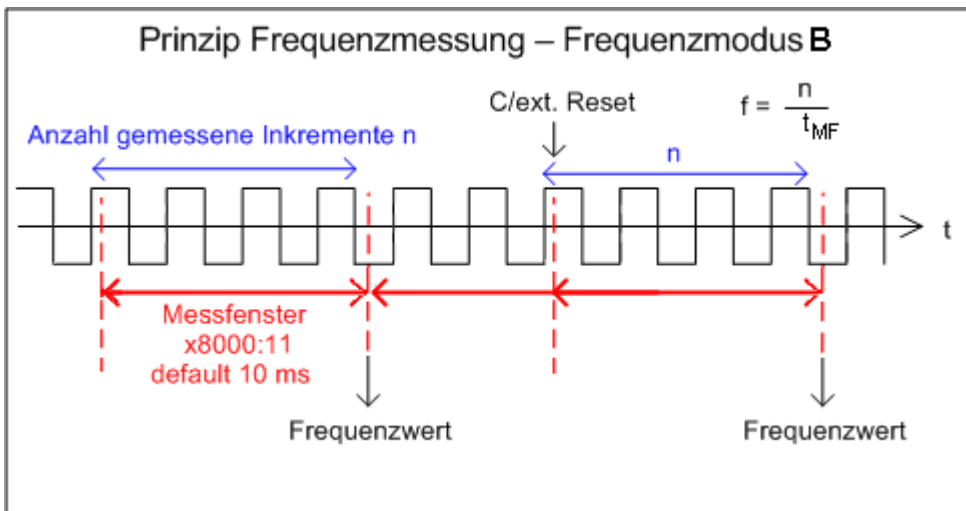
Abb. 148: Prinzip Frequenzmessung - Frequenzmodus B
