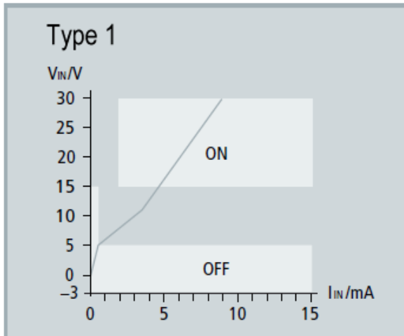
Abb. 9: Kennlinie Eingang 24 V DC Typ 1
