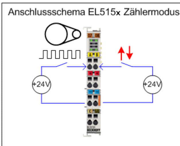
Abb. 149: Prinzip Zähleranschluss
