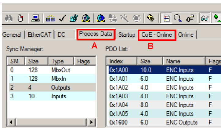
Abb. 143: Parametrierung am Beispiel EL5151
