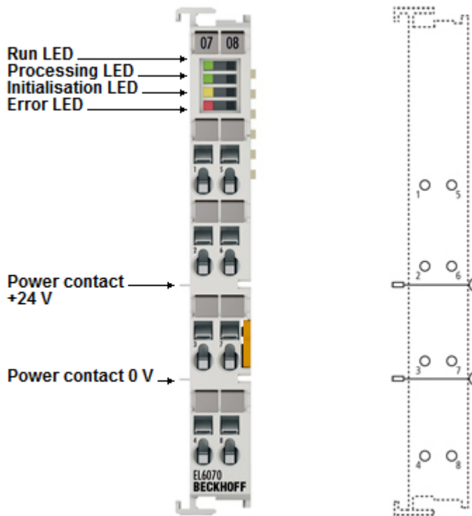
Abb. 21: LEDs and Anschlussbelegung
