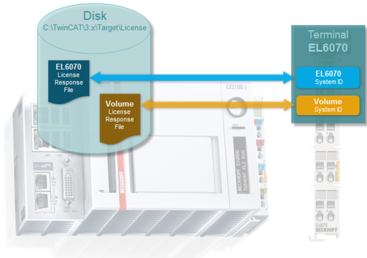
Abb. 23: TwinCAT Dongle Architektur
