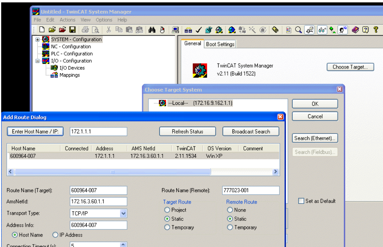
Abb. 177: Eingabe Zielsystem 172.1.1.1
