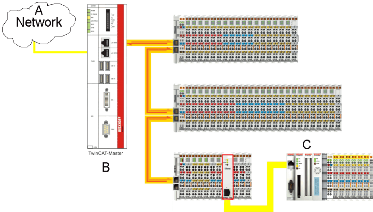
Abb. 166: Einrichten eines EtherCAT-Master-PC als Netzwerk Bridge
