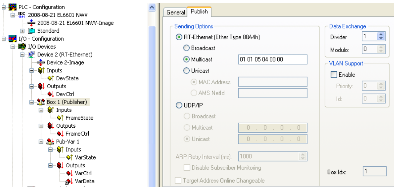
Abb. 126: Einstellungen Publisher - RT Ethernet
