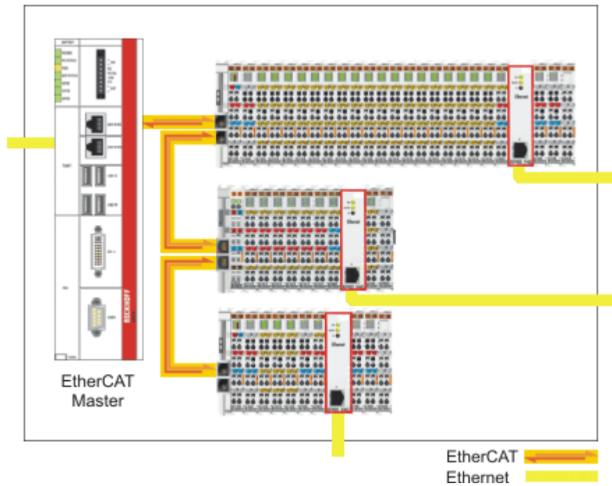
Abb. 5: EL6601 als im Feld verteilter, virtueller Switch
