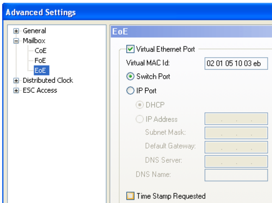
Abb. 10: Standard-einstellung der EL66xx als Switch-Port ohne IP-Adressenvergabe
