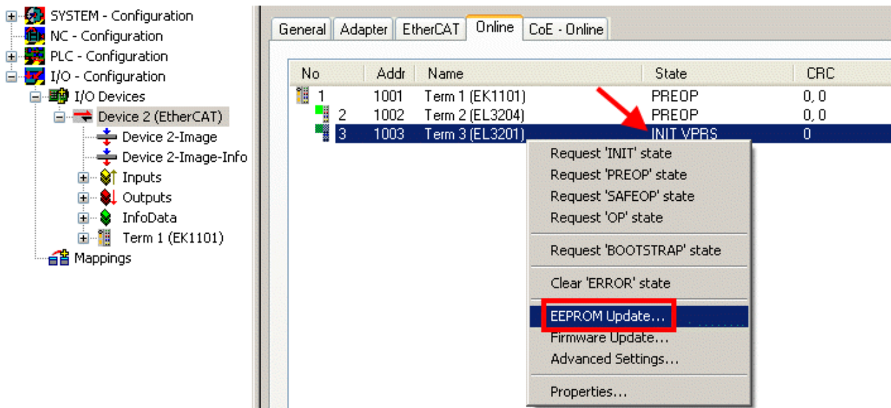
Abb. 185: EEPROM Update
