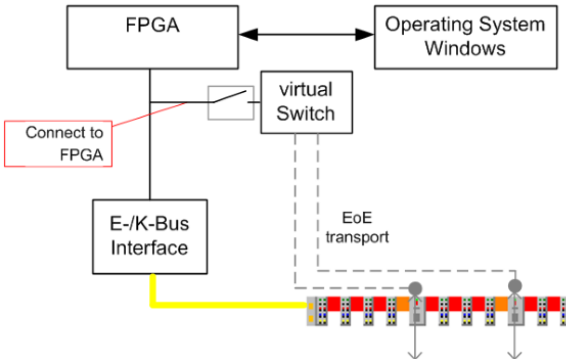
Abb. 29: Virtueller TwinCAT Switch im CX20x0 & CX50x0 System
