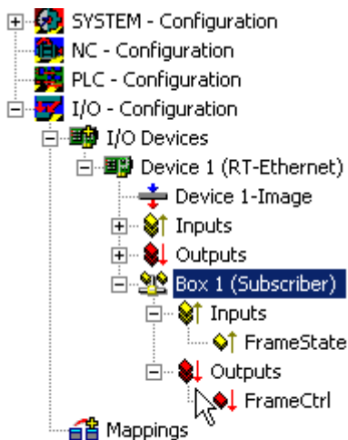
Abb. 116: Anlegen einer Subscriber Box ("Box 1")
