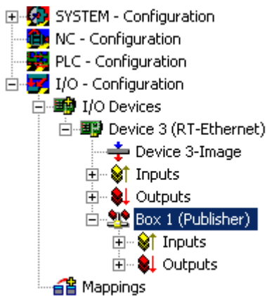
Abb. 111: Einfügen einer Publisher Box in die TwinCAT Konfiguration
