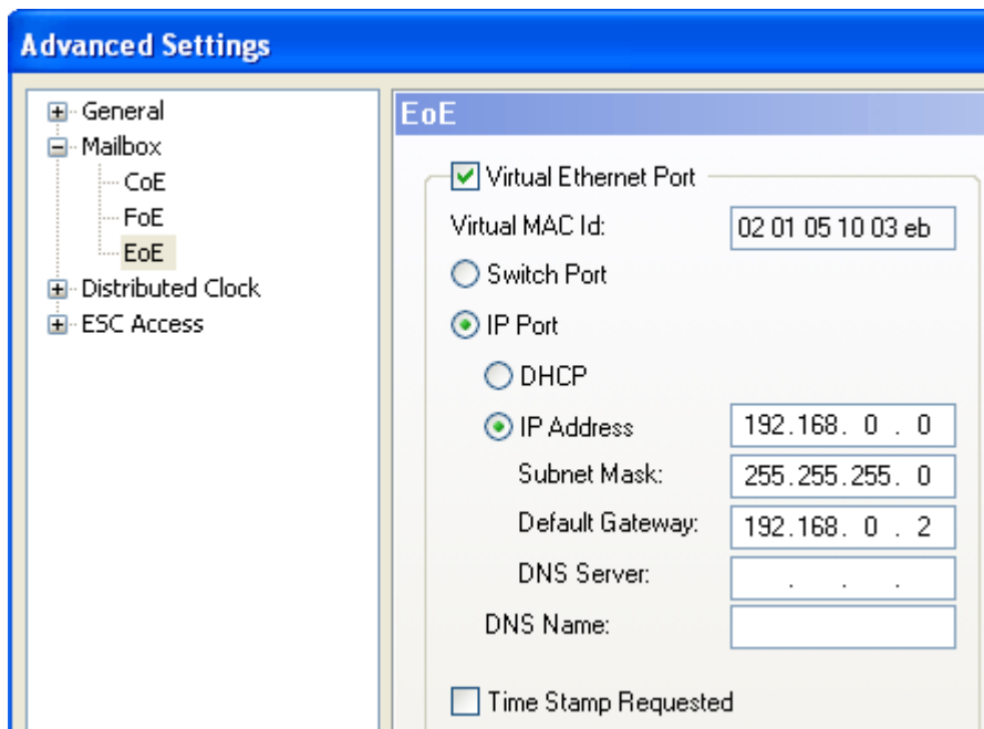
Abb. 11: Ab FW03: Einstellungen für dynamisch vergebene IP-Adresse
