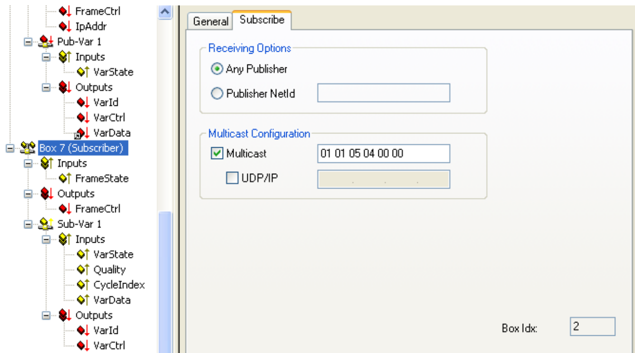
Abb. 129: Einstellungen Subscriber
