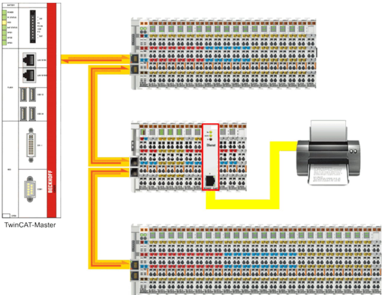
Abb. 131: Anbindung eines Netzwerkdruckers
