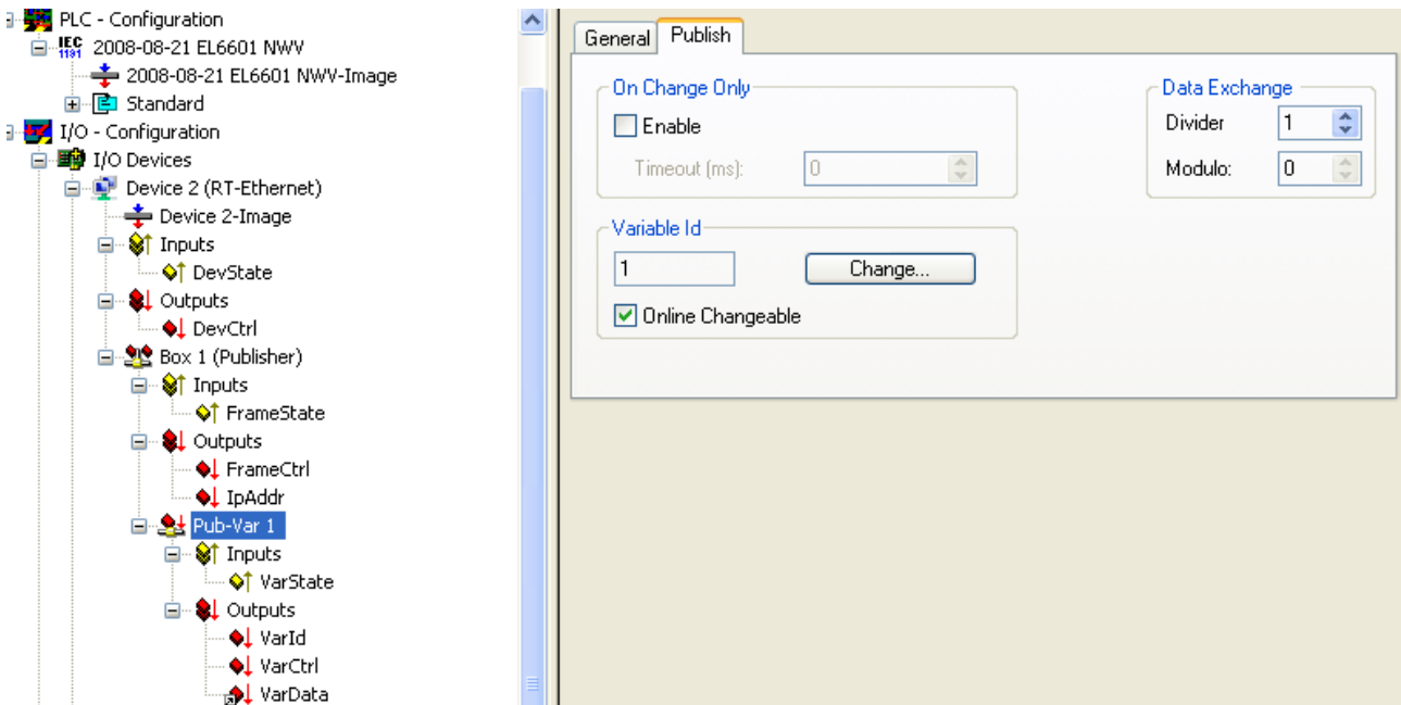
Abb. 128: Einstellungen Publisher - Variable
