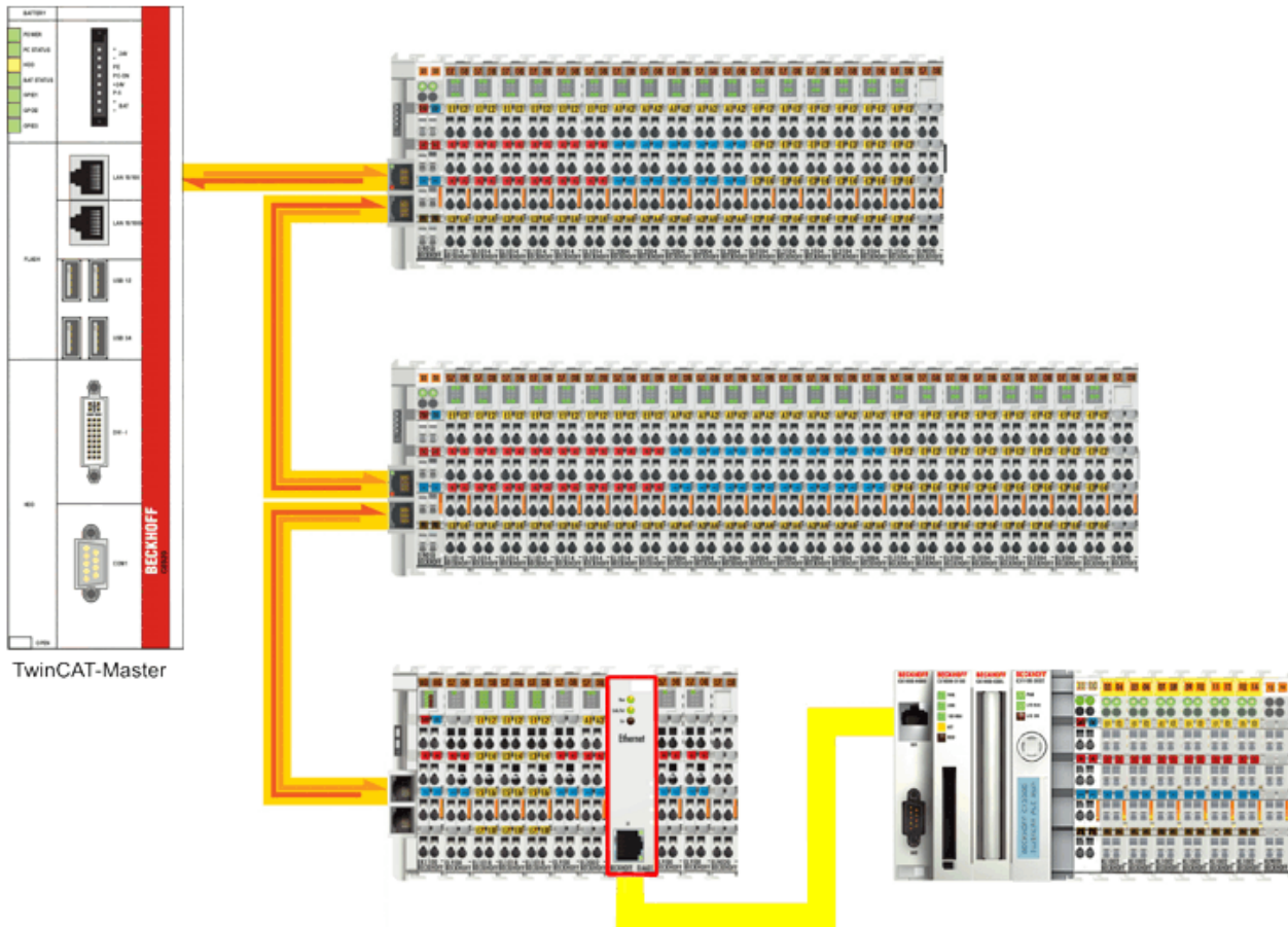
Abb. 157: Einbindung einer unterlagerten Steuerung
