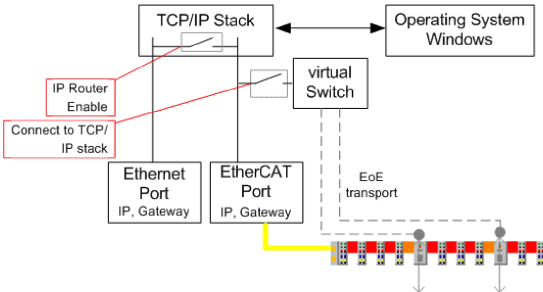
Abb. 14: TwinCAT 2.11, virtueller TwinCAT Switch
