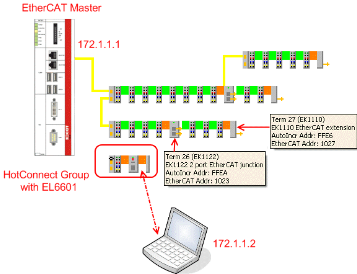
Abb. 173: Aufbau HotConnect-Gruppe
