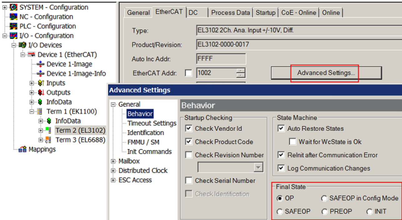
Abb. 106: Default Zielzustand im Slave
