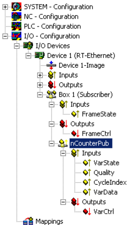
Abb. 120: Angelegte Ein-/Ausgänge der eingefügten Variablen
