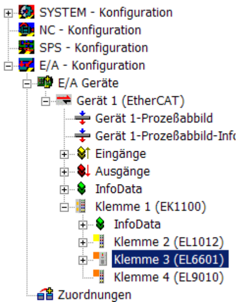
Abb. 142: EL6601 in der Konfiguration
