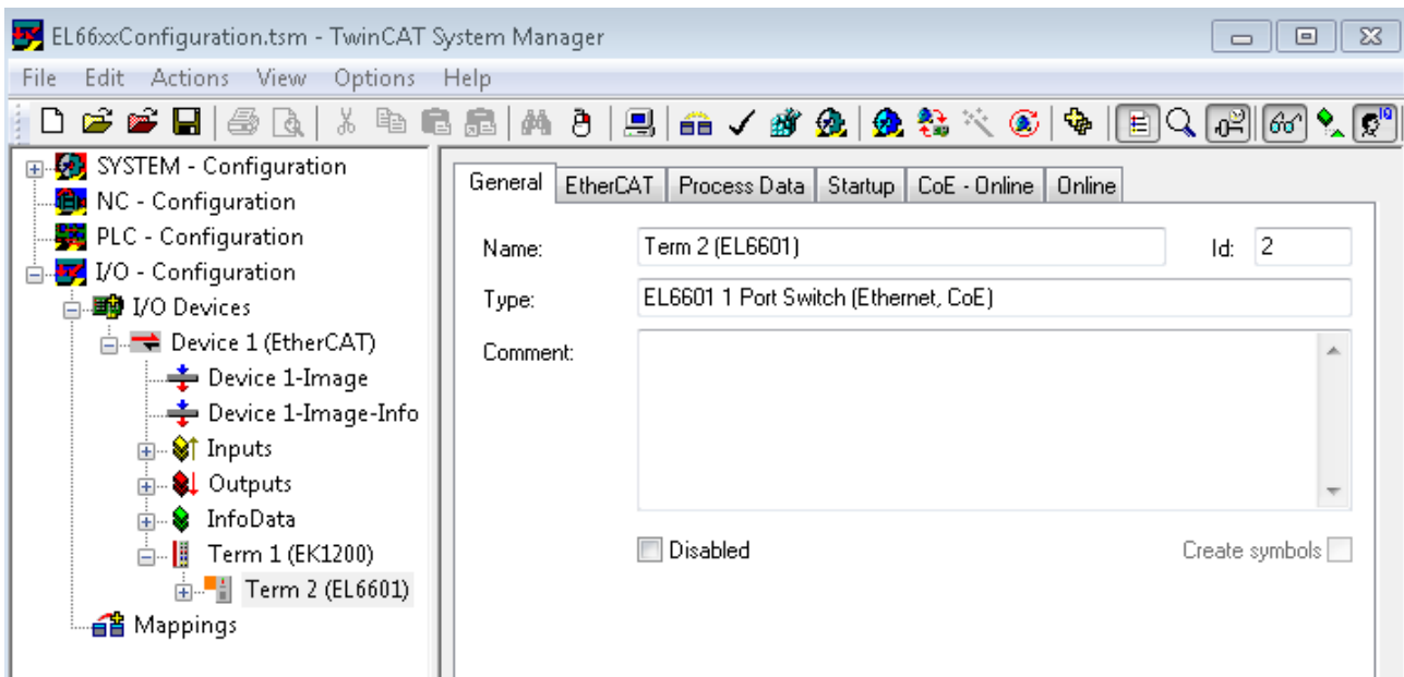
Abb. 31: Einfügen der EL66xx in die Konfiguration
