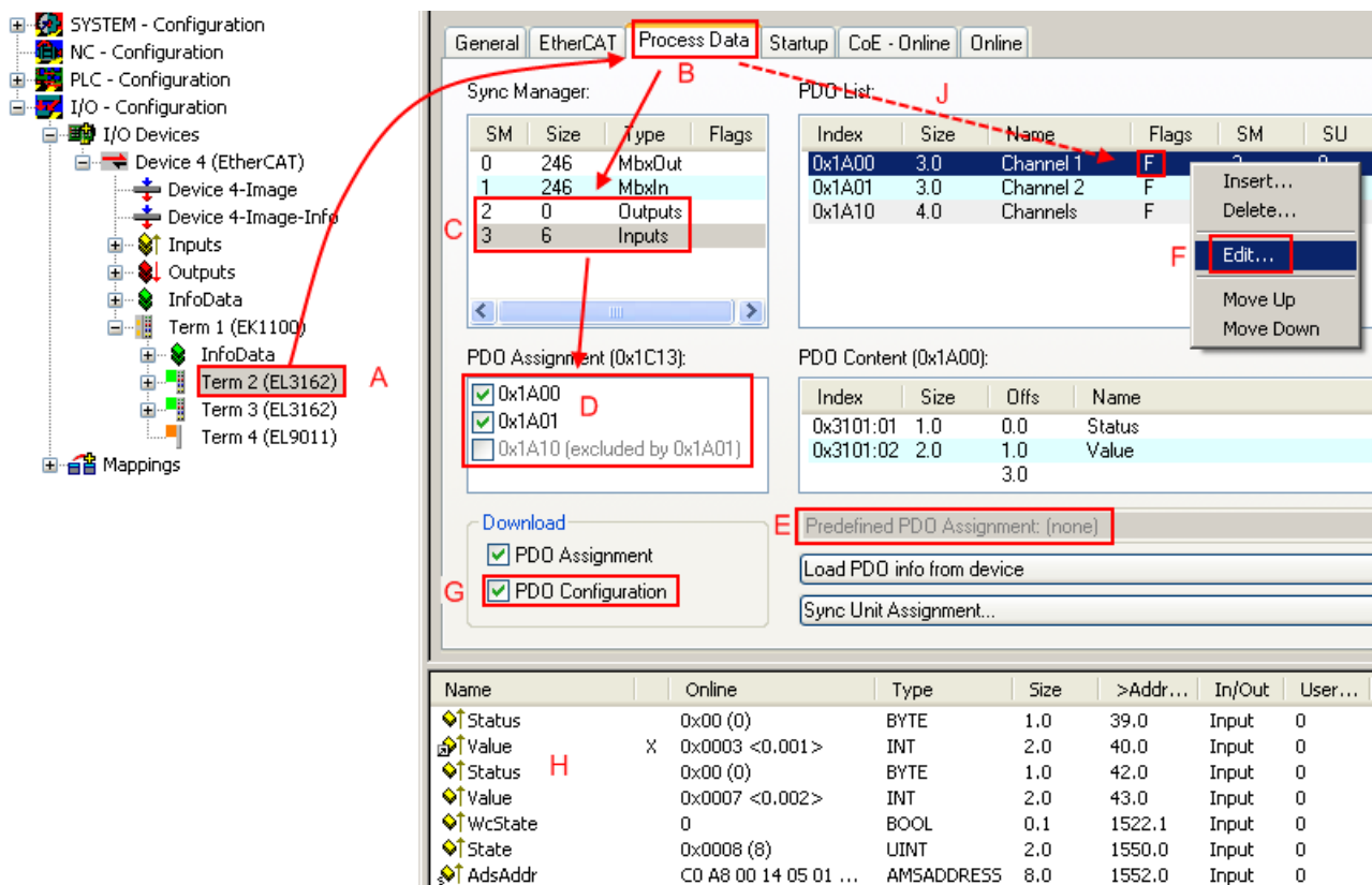
Abb. 95: Konfigurieren der Prozessdaten
