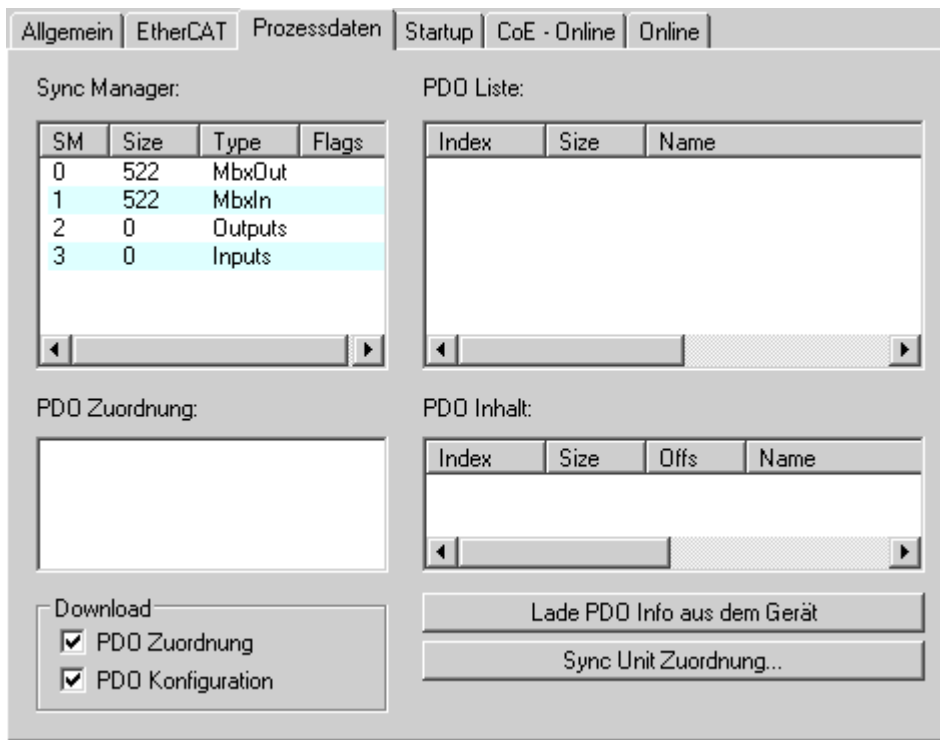
Abb. 12: Default Einstellungen der Mailbox
