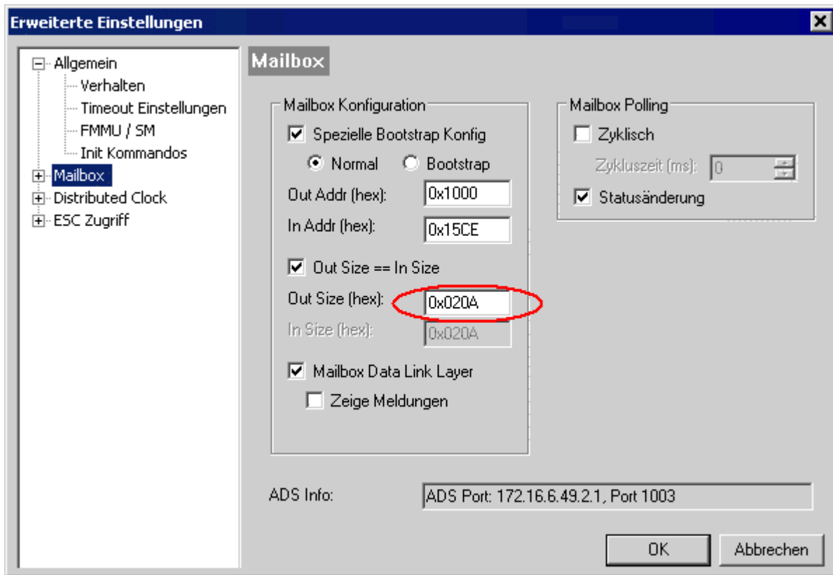
Abb. 13: Vergrößerung der Mailbox
