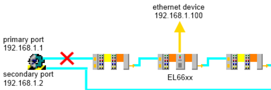
Abb. 8: Verbindungsausfall zwischen primären EtherCAT-Port und 1. Slave (X)
