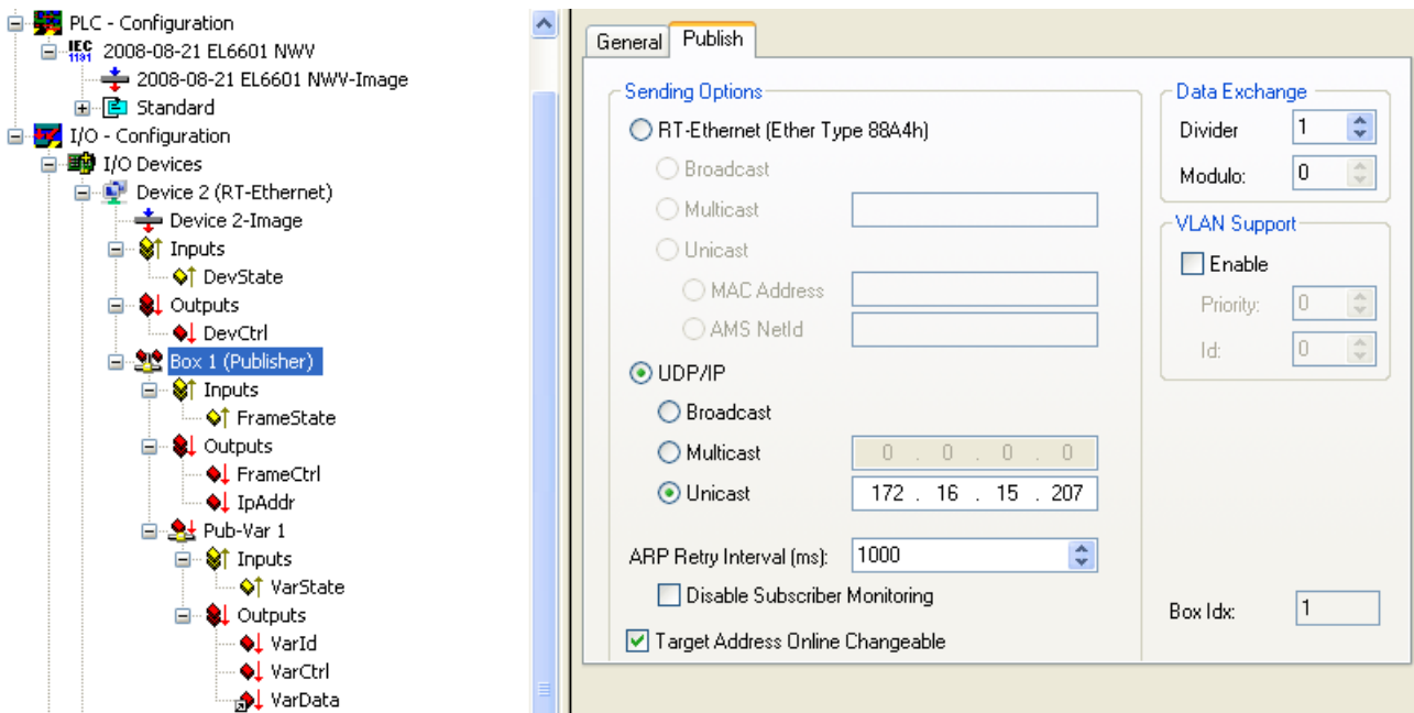
Abb. 127: Einstellungen Publisher - UDP/IP
