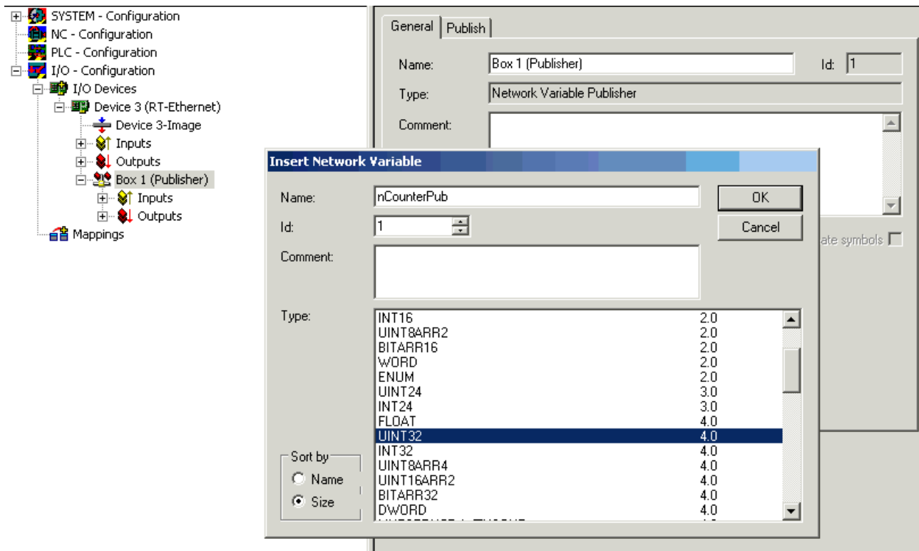
Abb. 112: Einfügen einer Netzwerk Variablen
