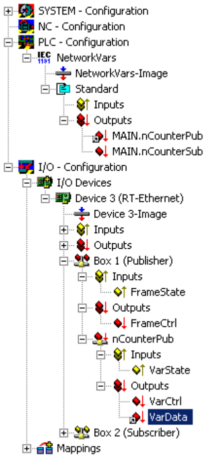
Abb. 114: Verknüpfung der Netzwerkvariablen mit der Ausgangsvariablen einer SPS
