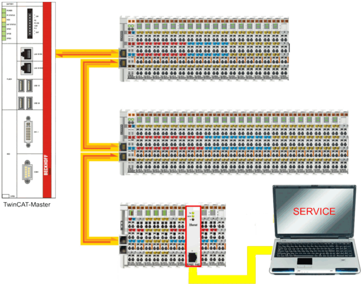
Abb. 141: Einbindung einer Service Schnittstelle mit Remotedesktop-PC
