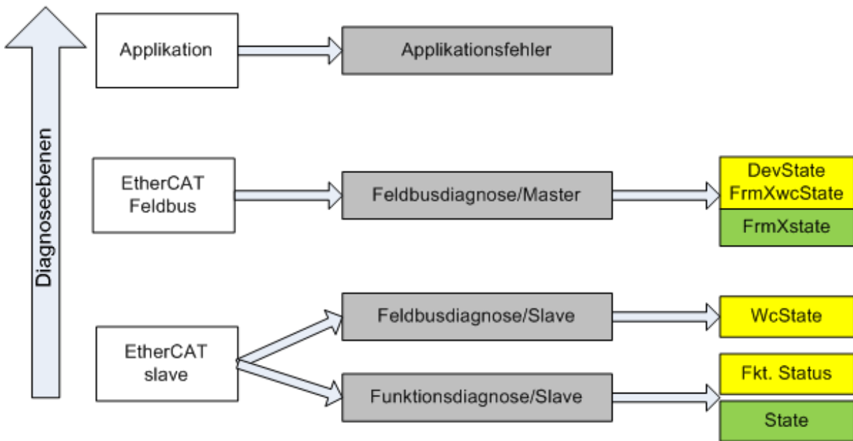
Abb. 101: Auswahl an Diagnoseinformationen eines EtherCAT Slave
