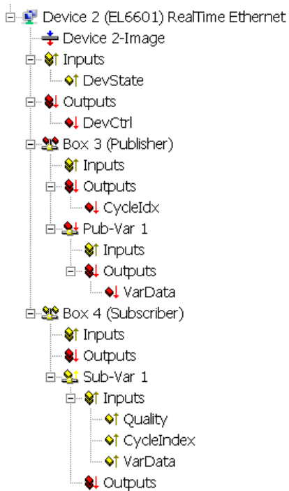
Abb. 17: Beispielkonfiguration Netzwerkvariablen auf EL6601
