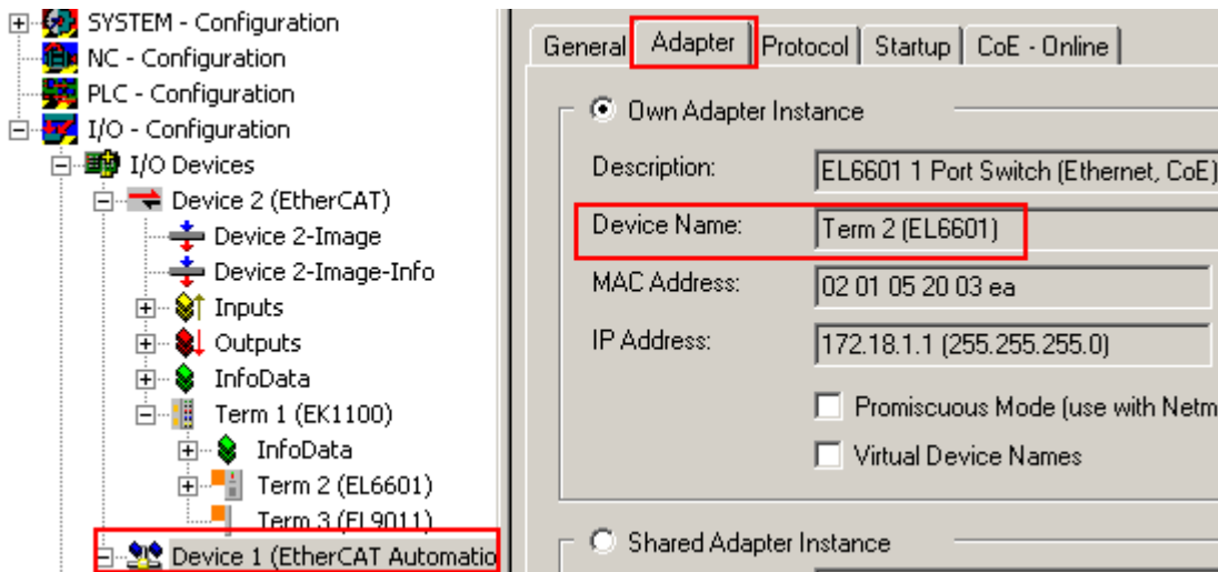
Abb. 25: Gerätezuordnung zur EL66xx
