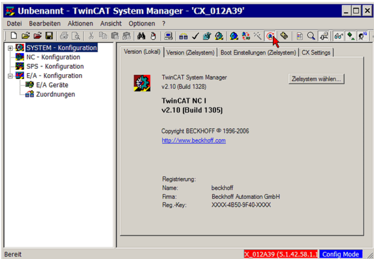
Abb. 165: FreeRun aktivieren
