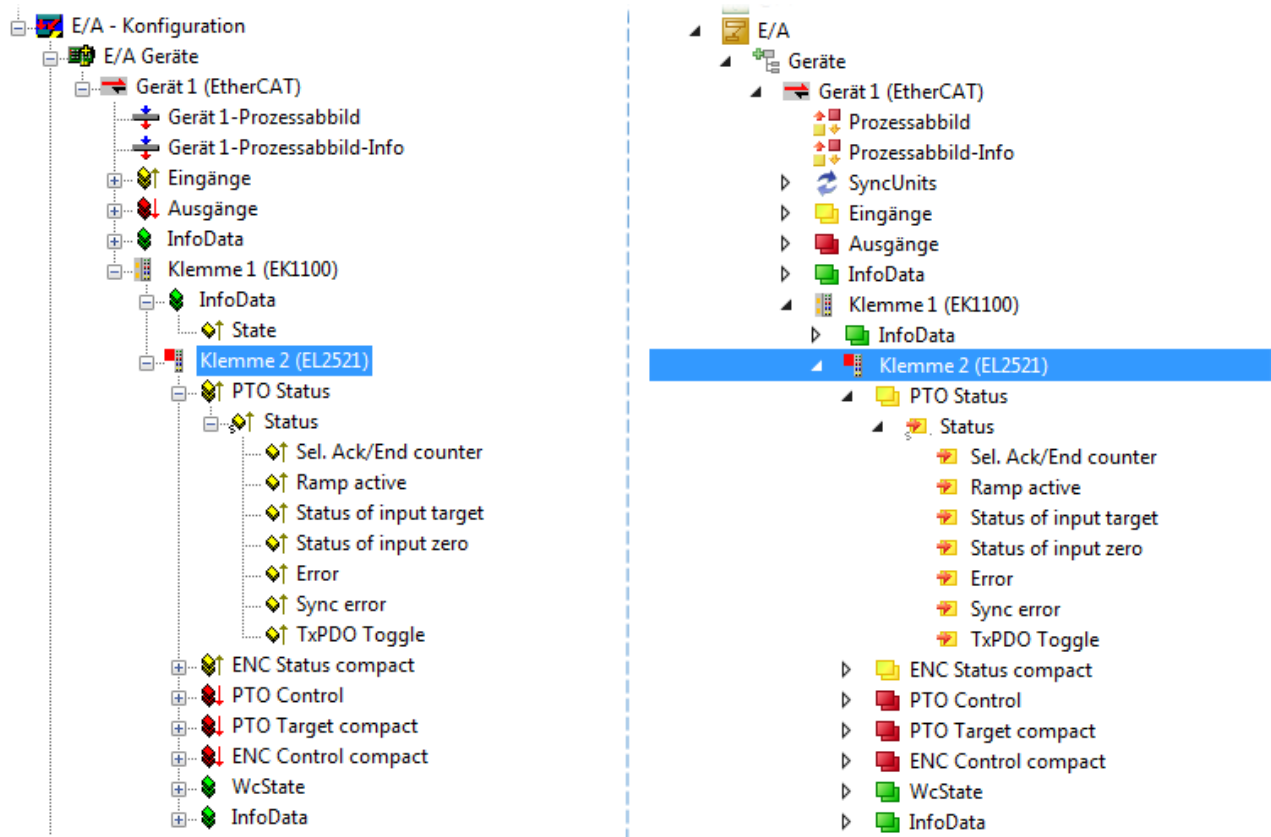
Abb. 69: EtherCAT Klemme im TwinCAT-Baum (links: TwinCAT 2; rechts: TwinCAT 3)
