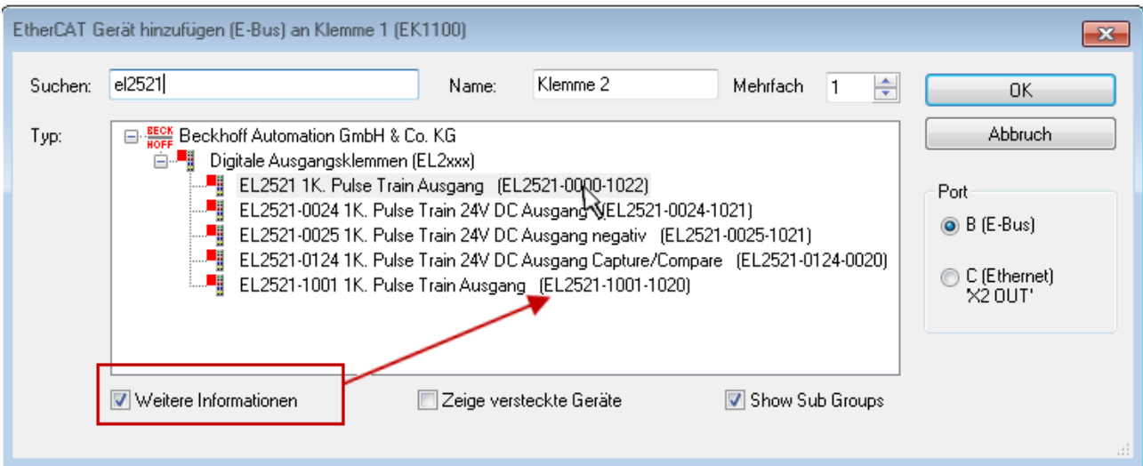
Abb. 66: Anzeige Geräte-Revision
