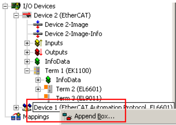
Abb. 26: Box anfügen
