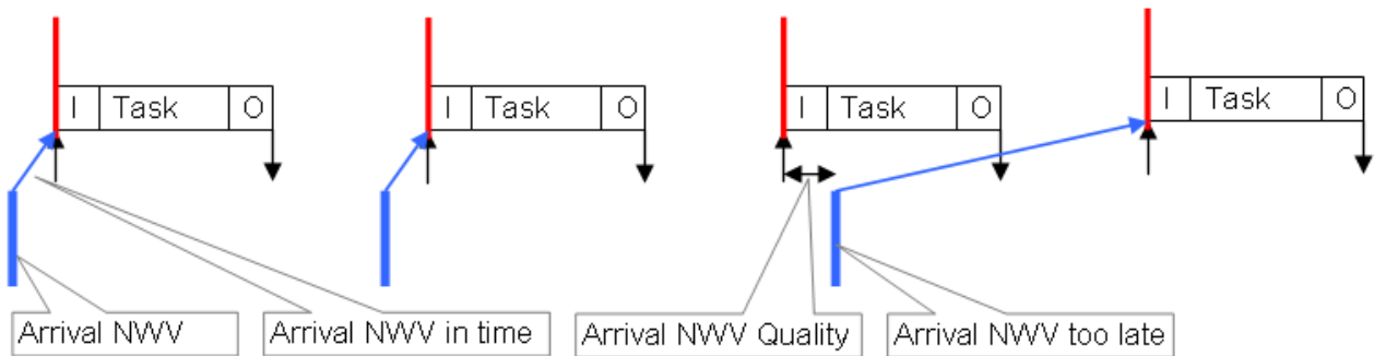
Abb. 123: Zusammenhang Quality und verspätet angekommenen Netzwerkvariable
