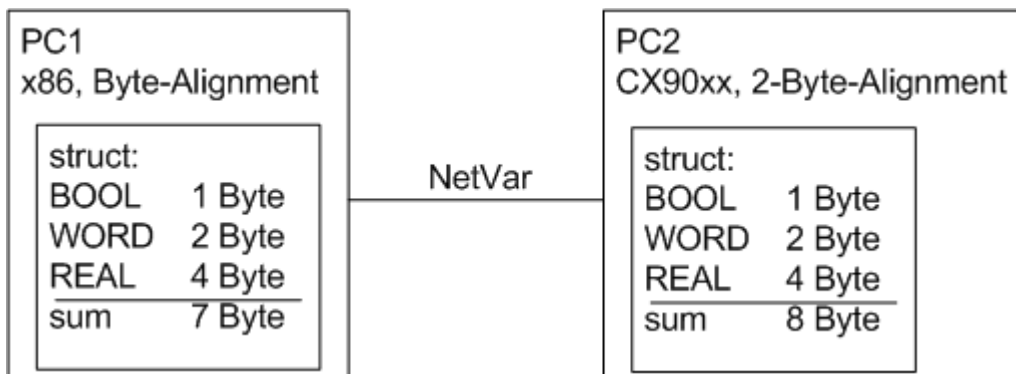
Abb. 125: Datendarstellung z.B. x86 Systeme vs. ARM Systeme
