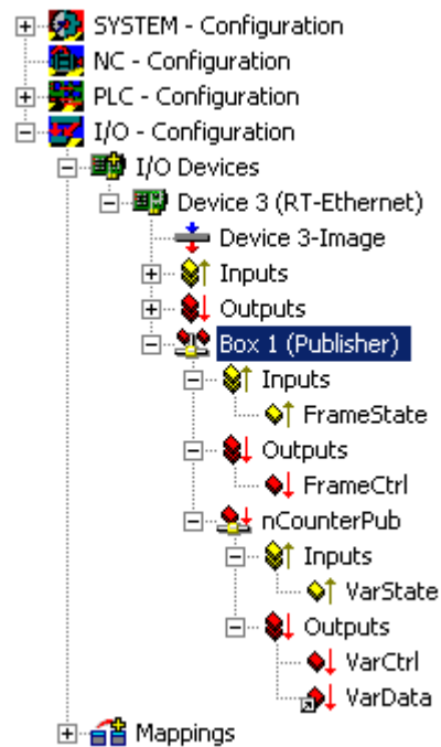
Abb. 113: Inputs/Outputs der eingefügten Variablen
