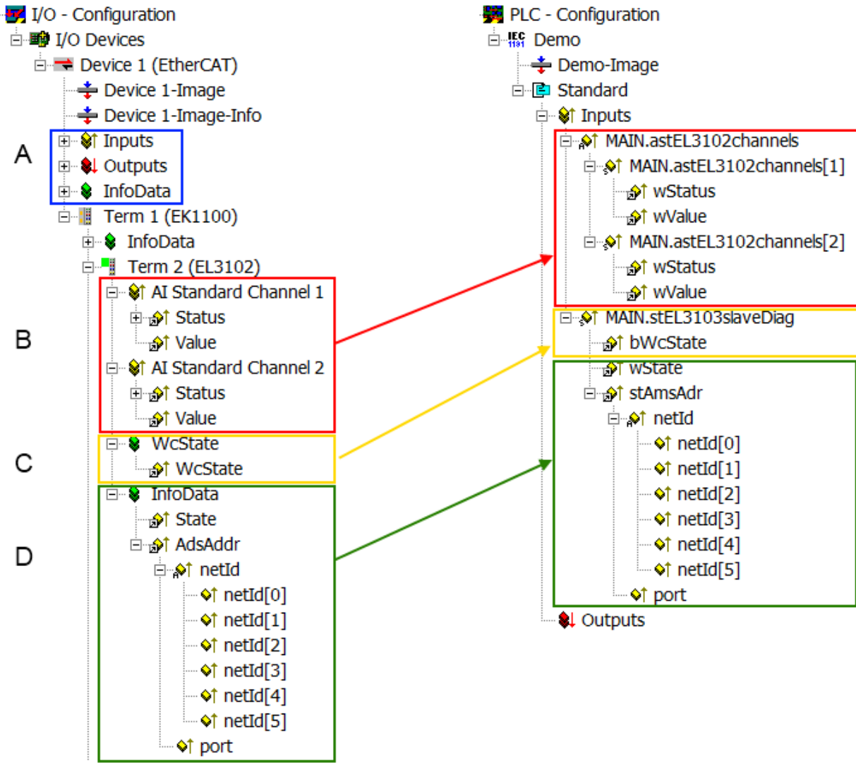
Abb. 102: Grundlegende EtherCAT Slave Diagnose in der PLC
