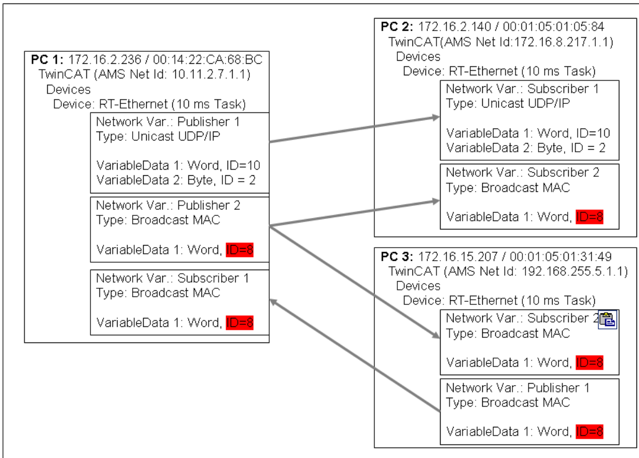
Abb. 124: Beispielhafte Kommunikation über Netzwerkvariablen
