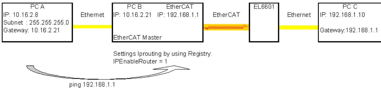
Abb. 167: Konfiguration der Netzwerk PC
