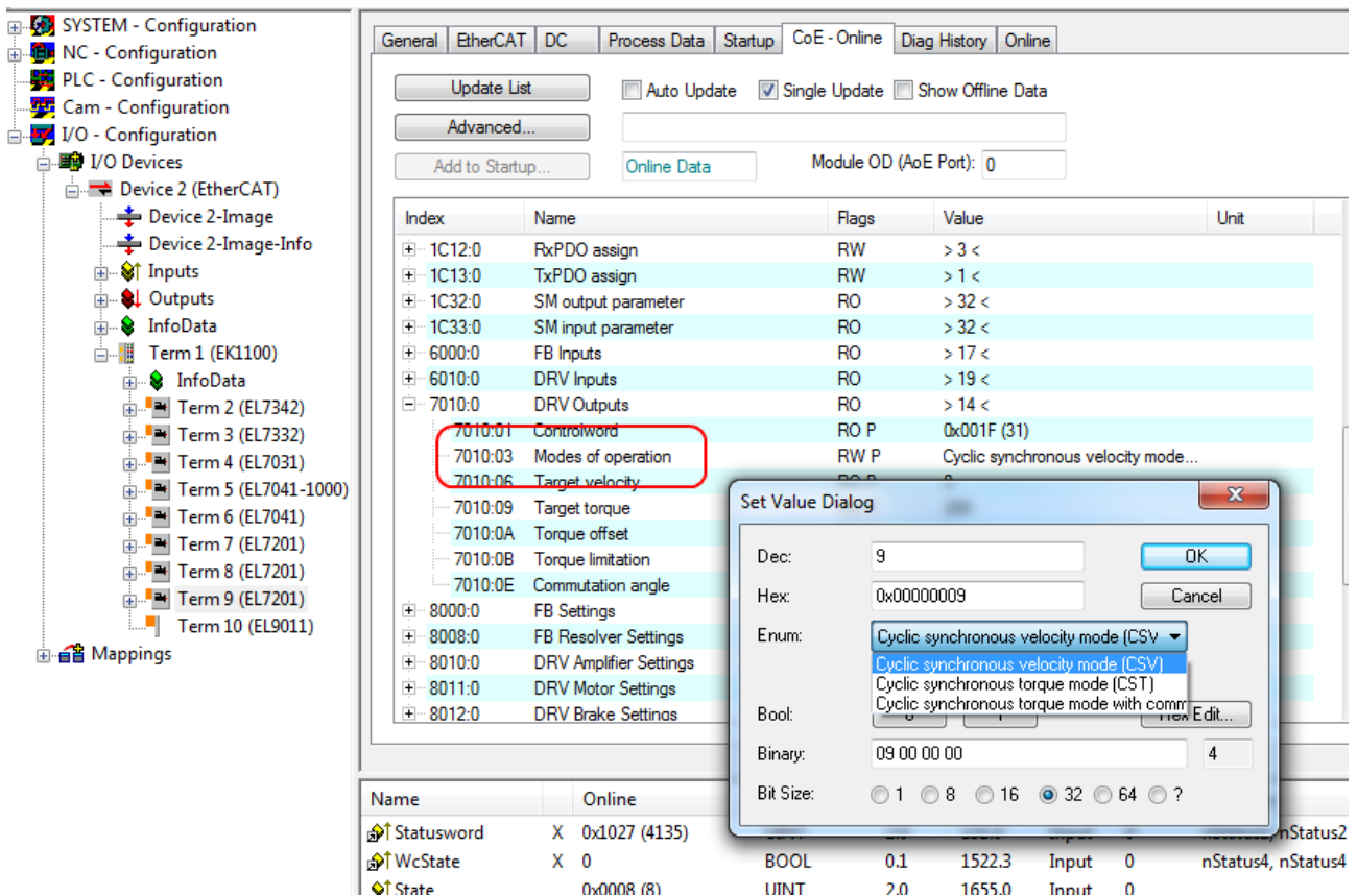
Abb. 185: Auswahl Betriebsart
