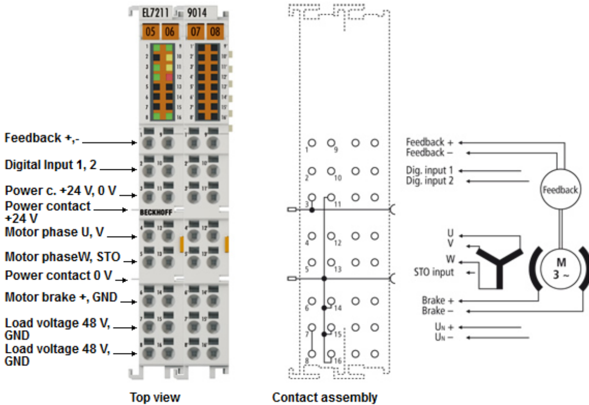
Abb. 37: EL7211-901x, EL7221-901x - Anschlussbelegung
