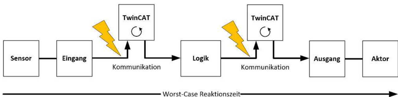
Abb. 212: Worst-Case-Reaktionszeit
