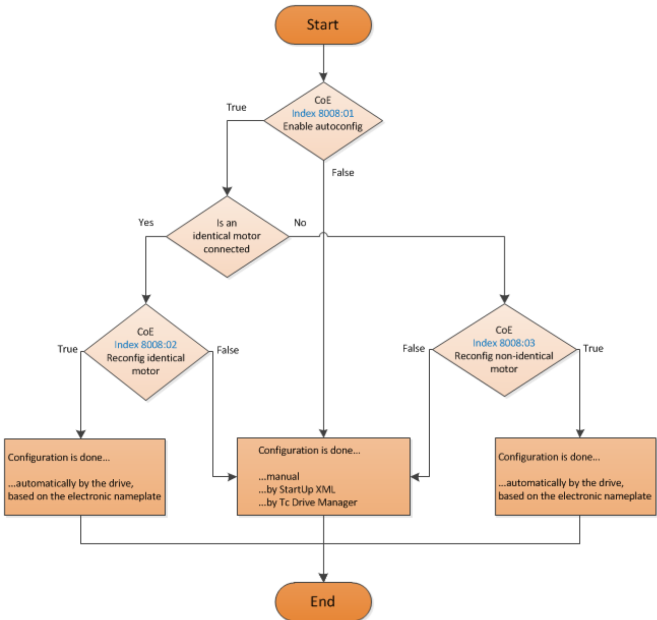
Abb. 176: Flussdiagramm der automatischen Konfiguration
