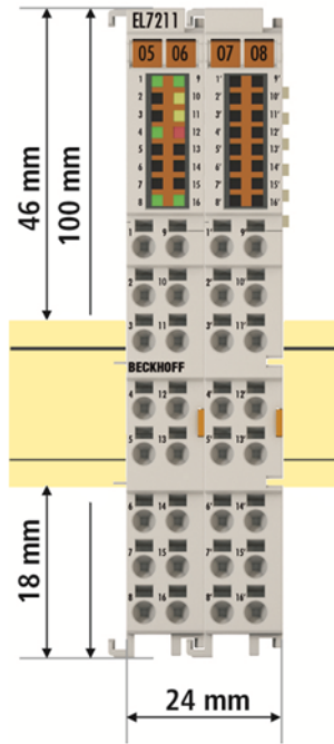
Abb. 210: Abmessung der EL7211-xxxx, EL7221-xxxx
