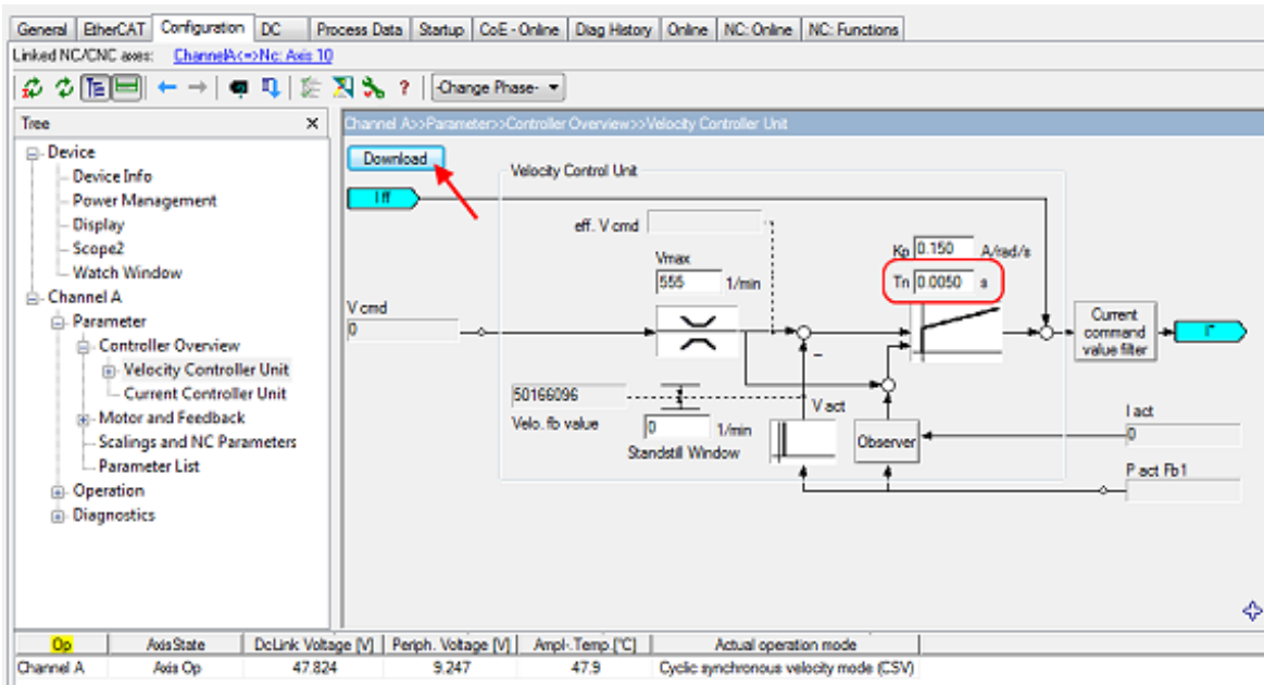
Abb. 152: Anpassung Tn
