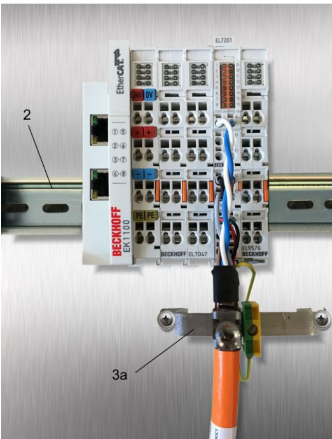
Abb. 31: Schirmschienen-Bügel
