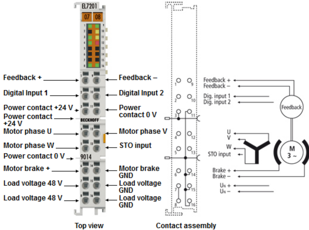
Abb. 35: EL7201-901x Anschlussbelegung
