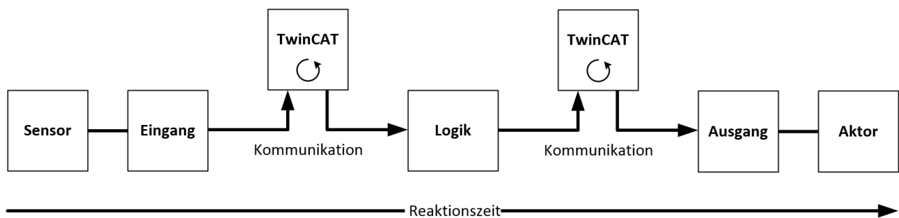
Abb. 211: Typische Reaktionszeit
