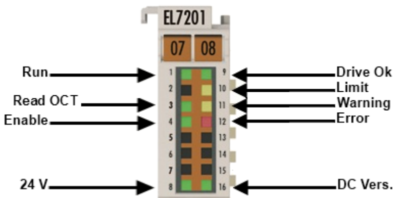
Abb. 34: EL7201-901x - LEDs
