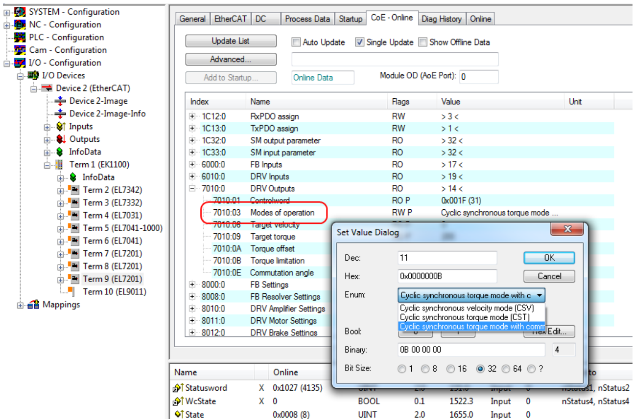
Abb. 193: Auswahl Betriebsart
