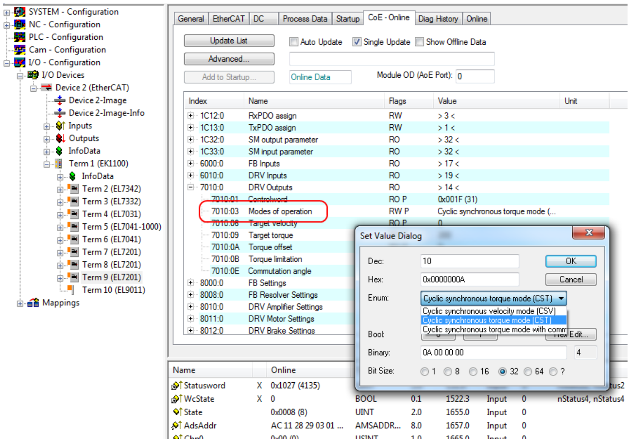
Abb. 189: Auswahl Betriebsart
