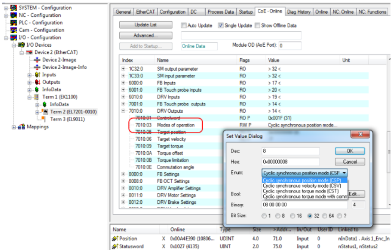
Abb. 197: Auswahl Betriebsart
