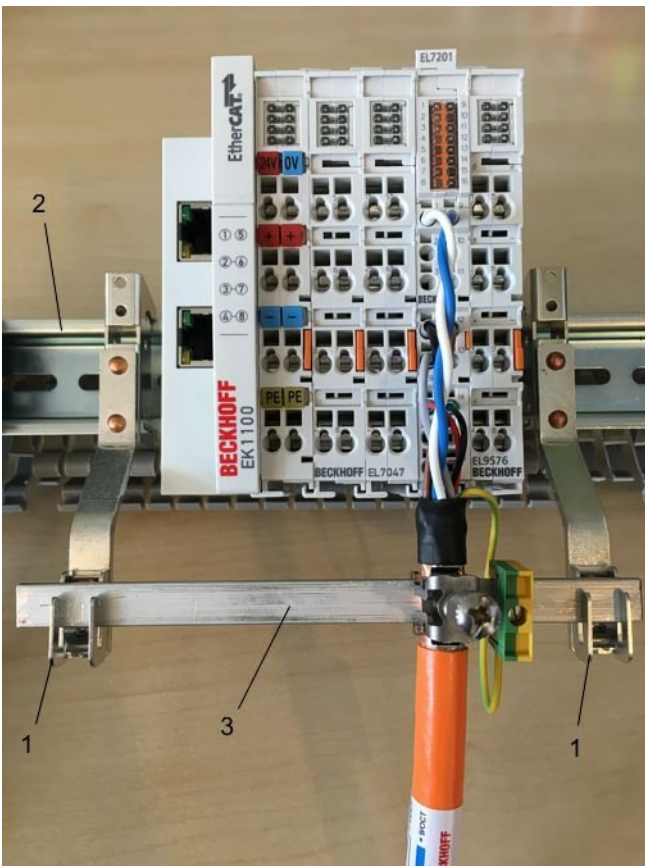
Abb. 30: Schirmschiene
