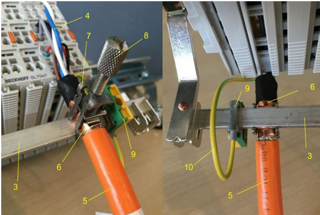
Abb. 32: Schirmanbindung
