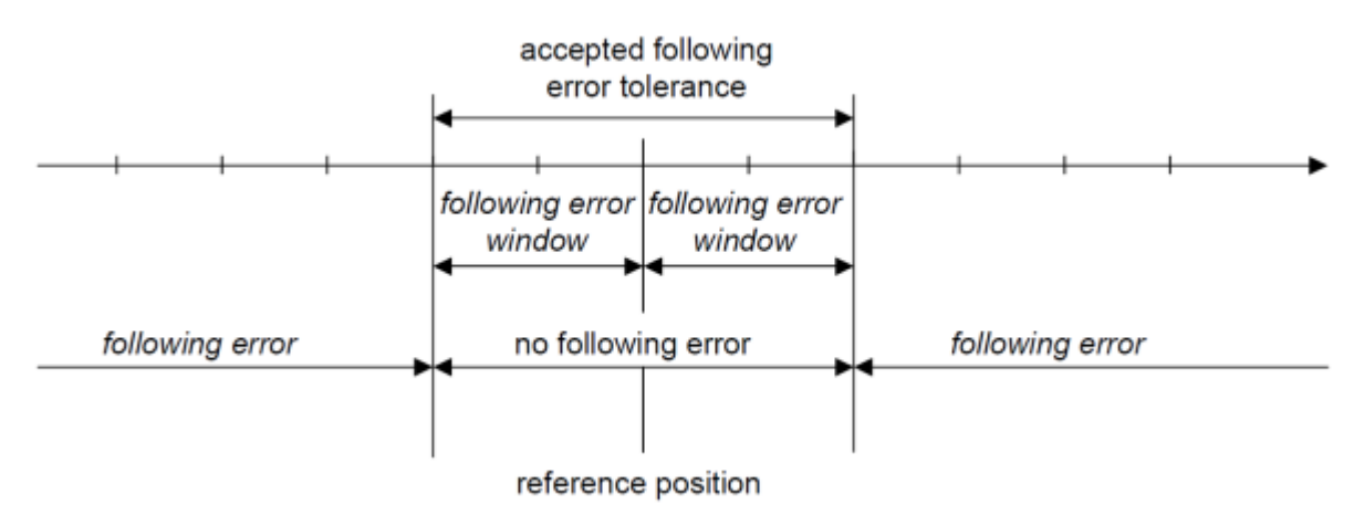
Abb. 201: Schleppfehlerfenster
