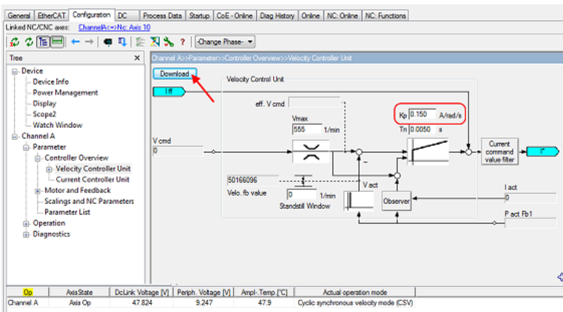
Abb. 153: Anpassung Kp
