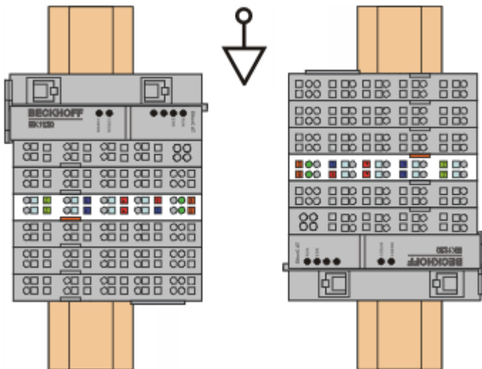
Abb. 21: Weitere Einbautagen, Beispiel 1
