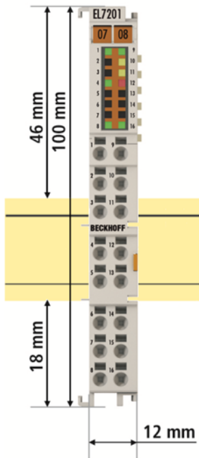
Abb. 209: Abmessung der EL7201-xxxx
