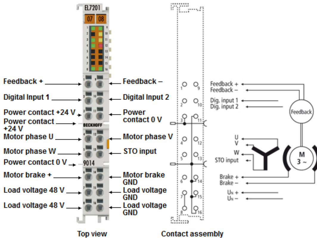
Abb. 4: EL7201-901x
