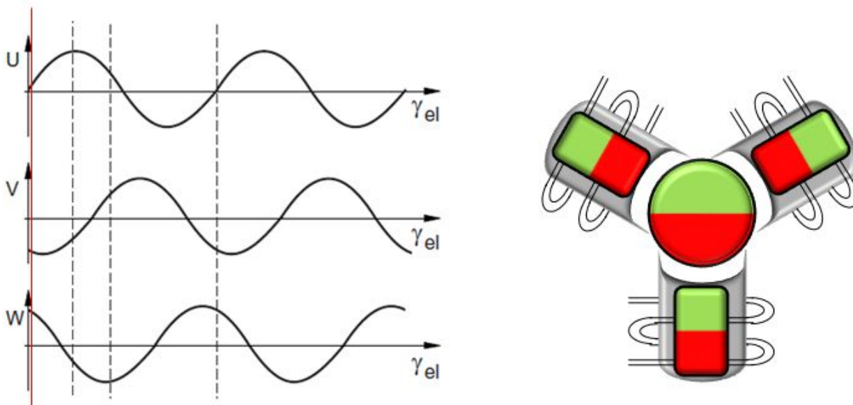
Abb. 6: Drei um 120° verschobenen Spulen eines Synchronmotors
