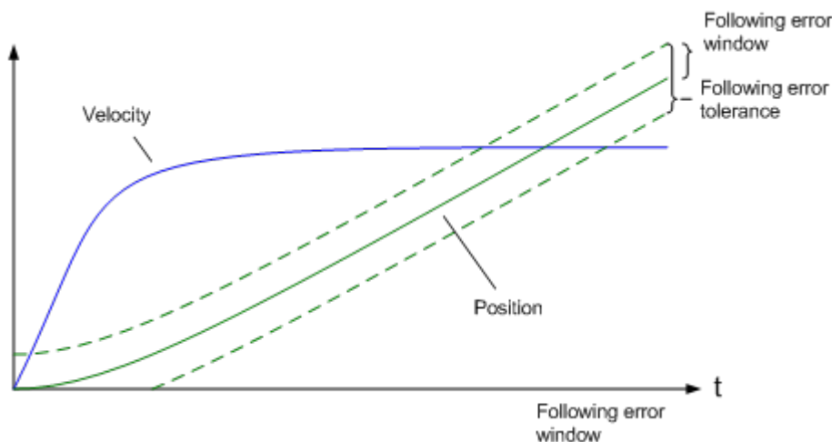
Abb. 156: Schleppfehler über die Zeit
