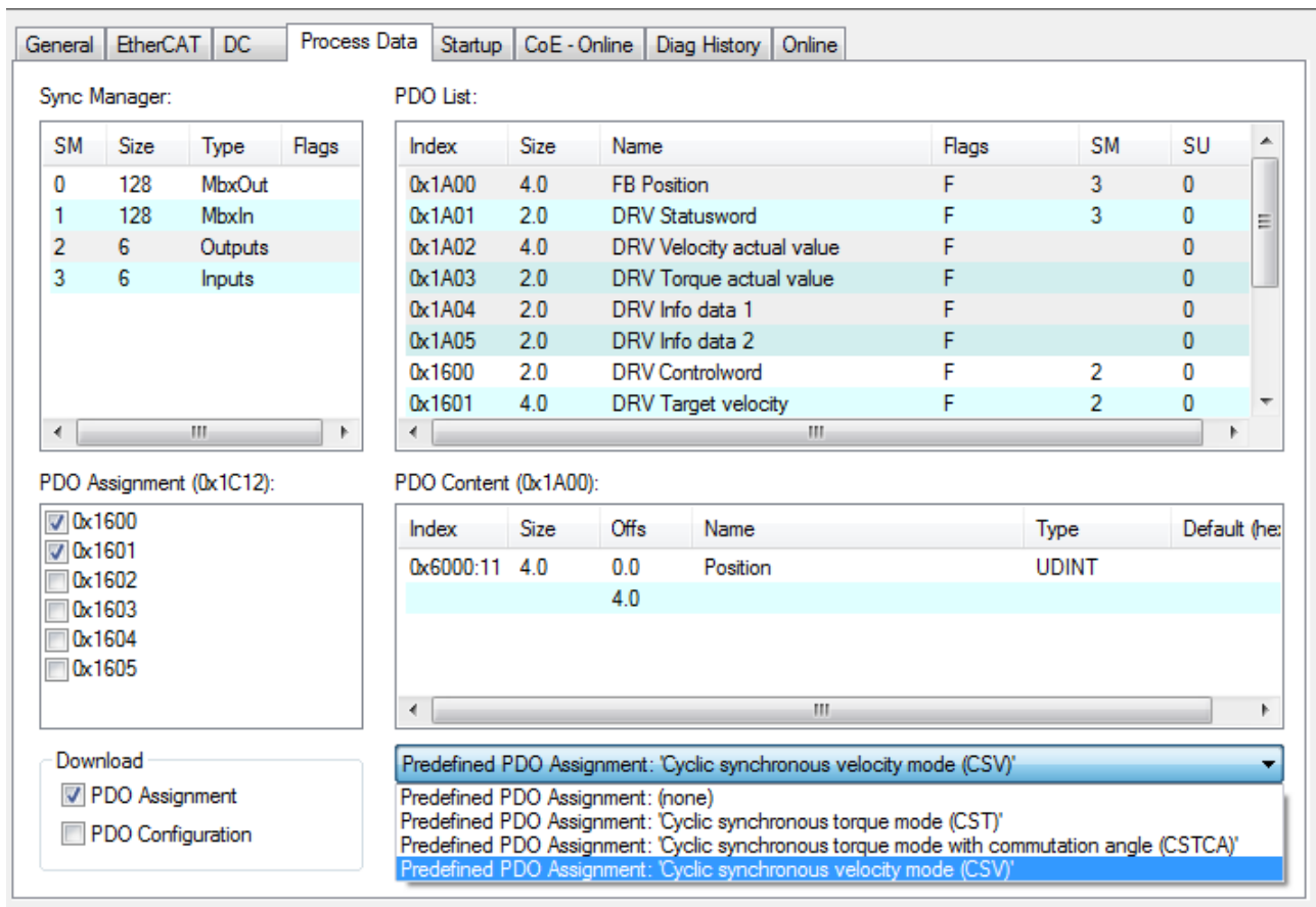
Abb. 140: Predefined PDO Assignment wählen
