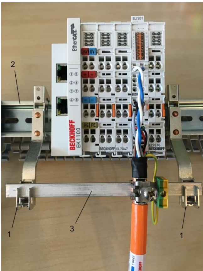
Abb. 29: Schirmschiene
