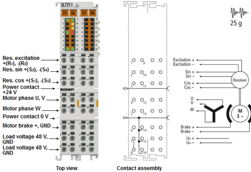
Abb. 36: EL7211, EL7211-001 Anschlussbelegung
