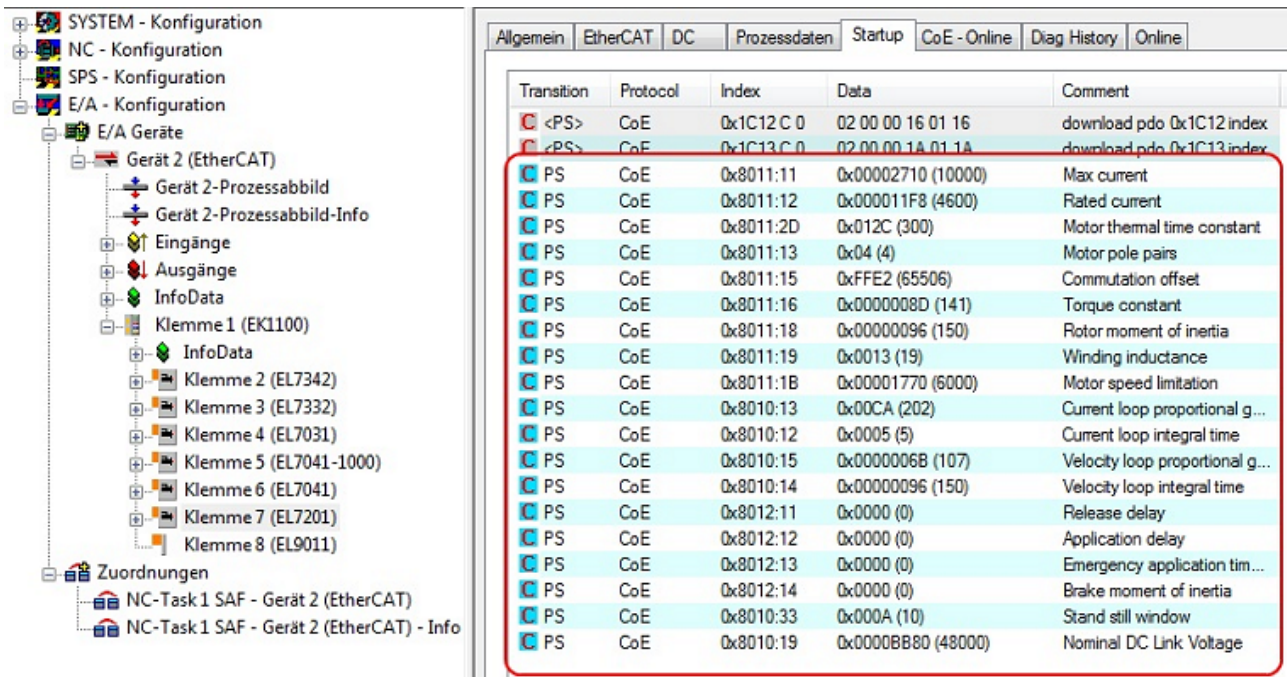
Abb. 113: CoE Parameter der Motor XML Datei
