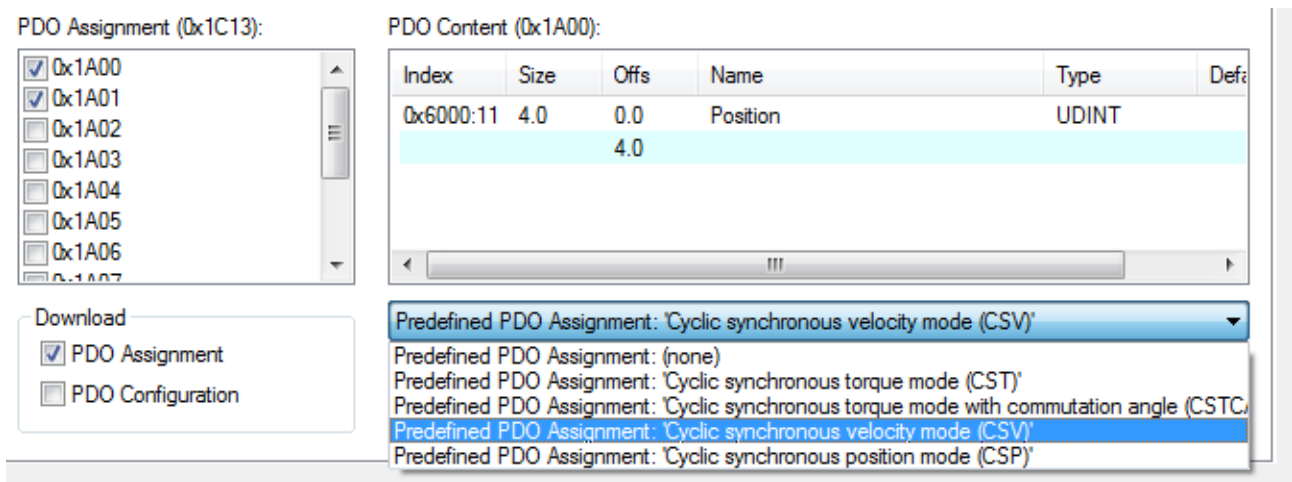
Abb. 162: Karteireiter Prozessdaten Predefined PDO Assignment, EL72x1
