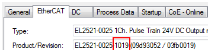
Abb. 71: Erkennen EtherCAT-Klemme mit Revision -1019
