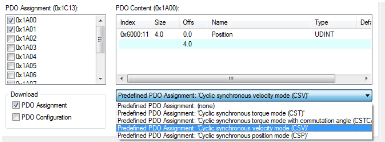
Abb. 159: Karteireiter Prozessdaten Predefined PDO Assignment, EL72x1
