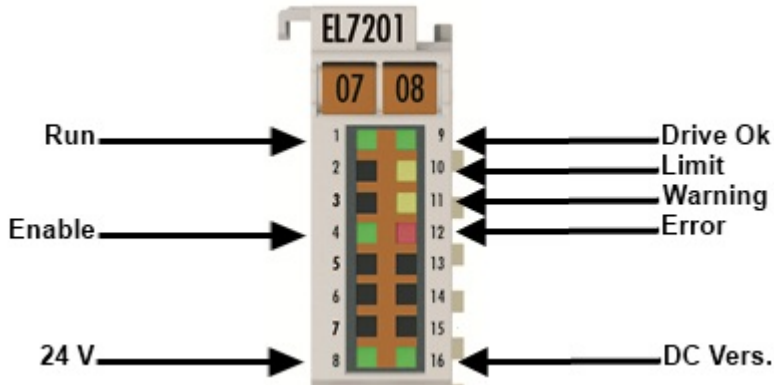
Abb. 33: EL7201, EL7201-0001 - LEDs
