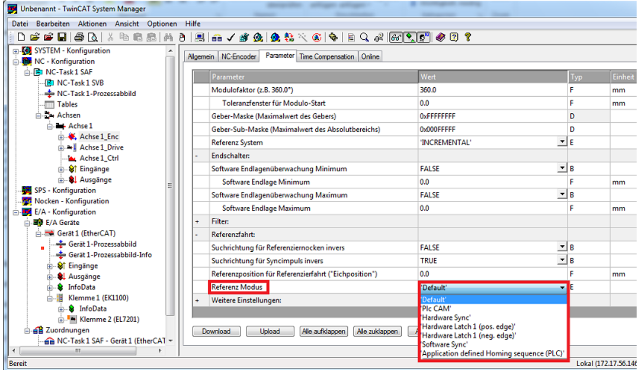
Abb. 128: Auswahl der Referenz Modi in der NC
