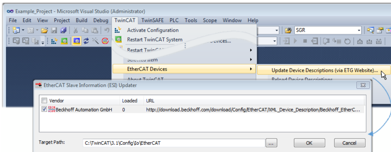
Abb. 54: Anwendung des ESI Updater (TwinCAT 3)
