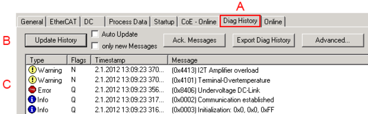
Abb. 164: Implementierung DiagMessage-System im TwinCAT System Manager
