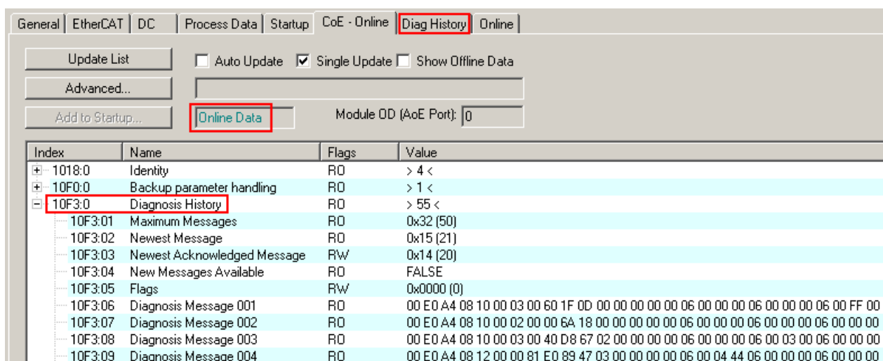
Abb. 163: DiagMessages im CoE
