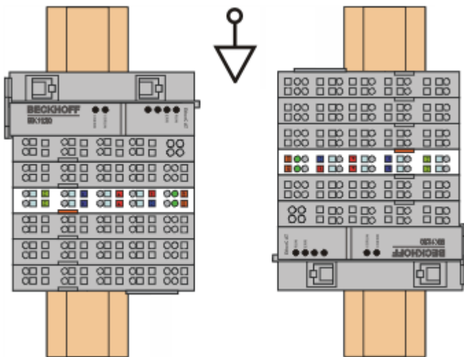
Abb. 27: Weitere Einbaulagen, Beispiel 1
