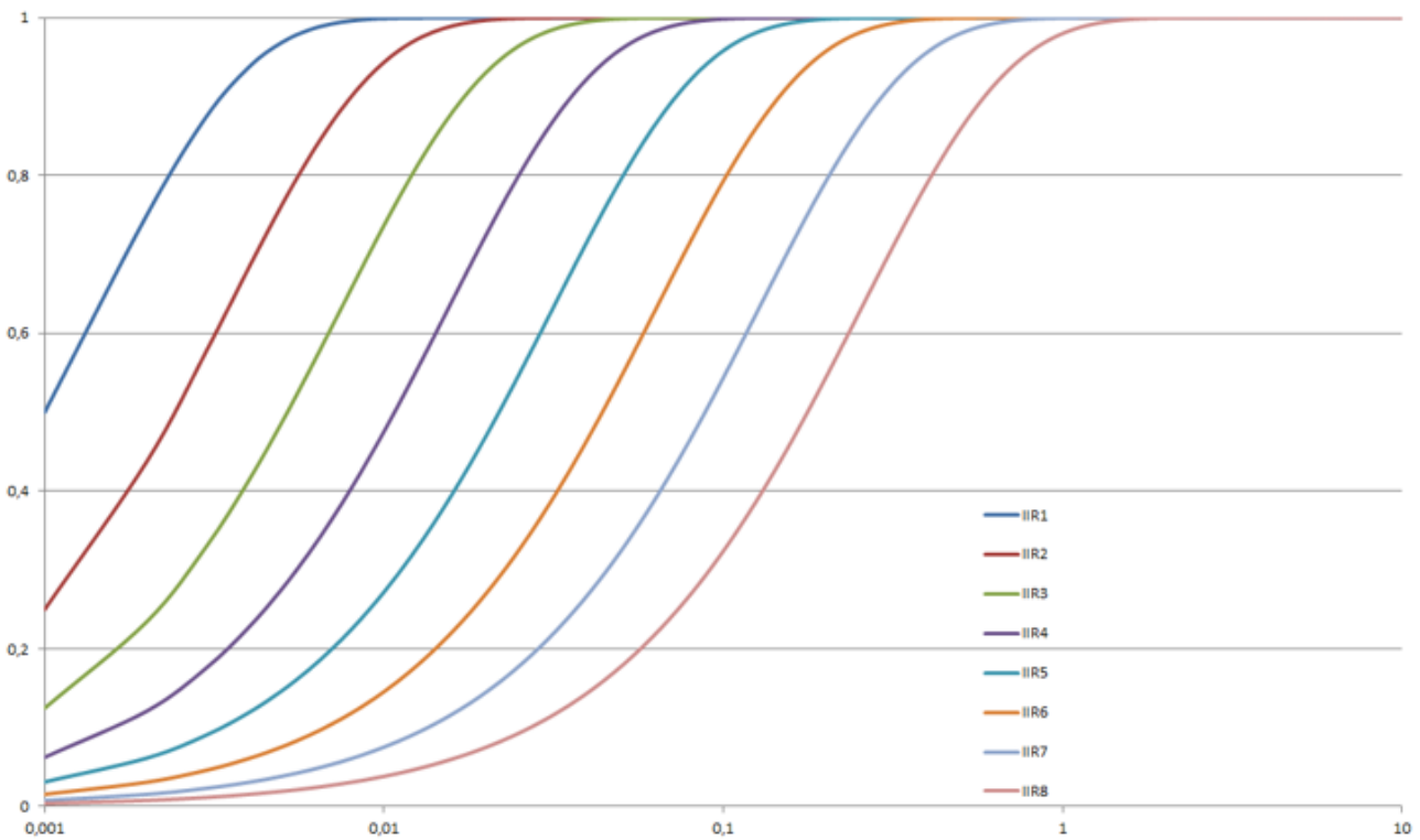
Abb. 95: EL9576 Sprungantwort der IIR Filter
