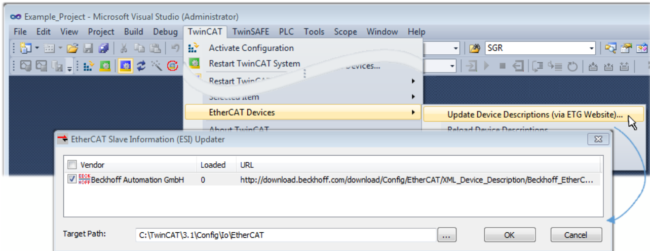
Abb. 41: Anwendung des ESI Updater (TwinCAT 3)
