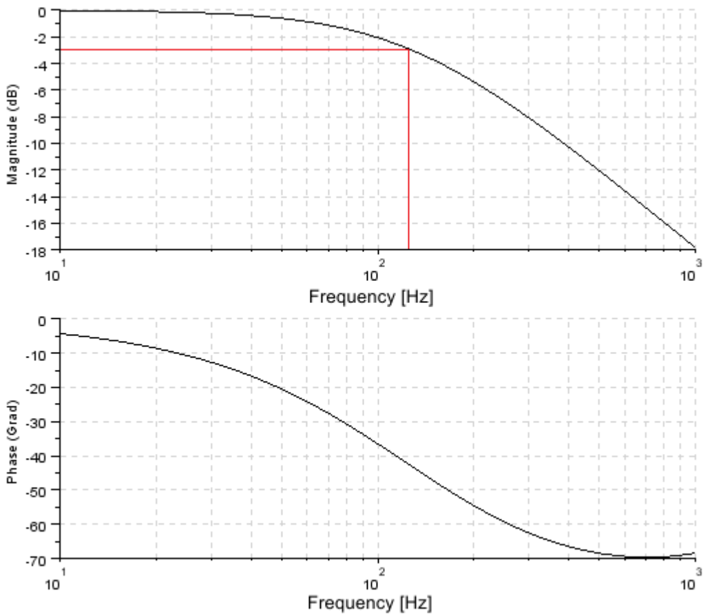
Abb. 96: Bodediagramm der IIR-Filter
