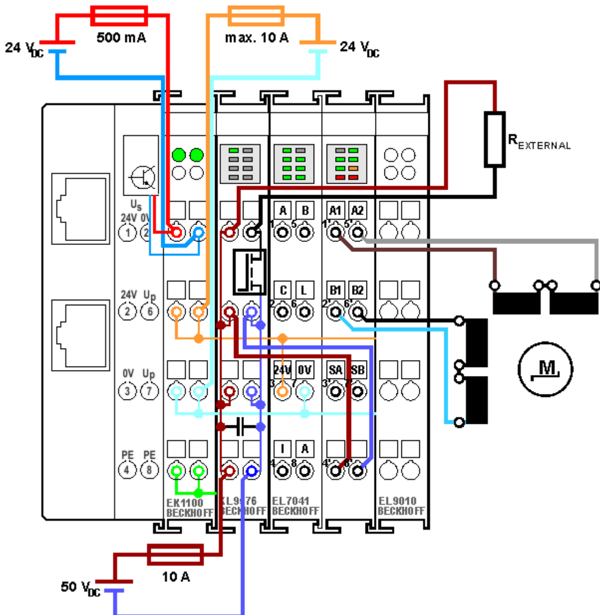
Abb. 99: Anschlussbeispiel
