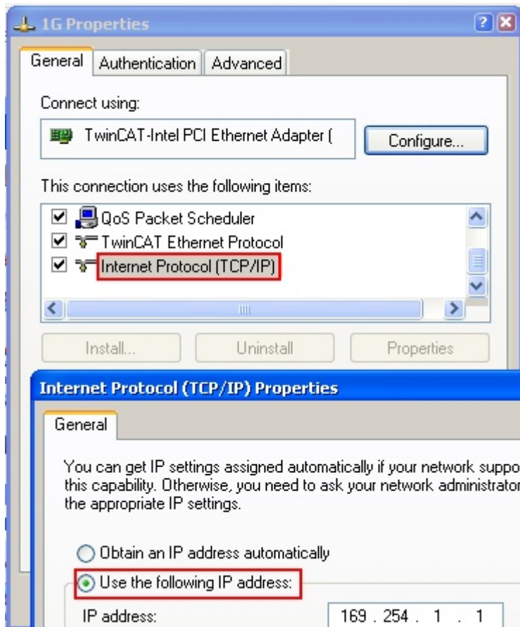
Abb. 33: TCP/IP-Einstellung des Ethernet Ports
