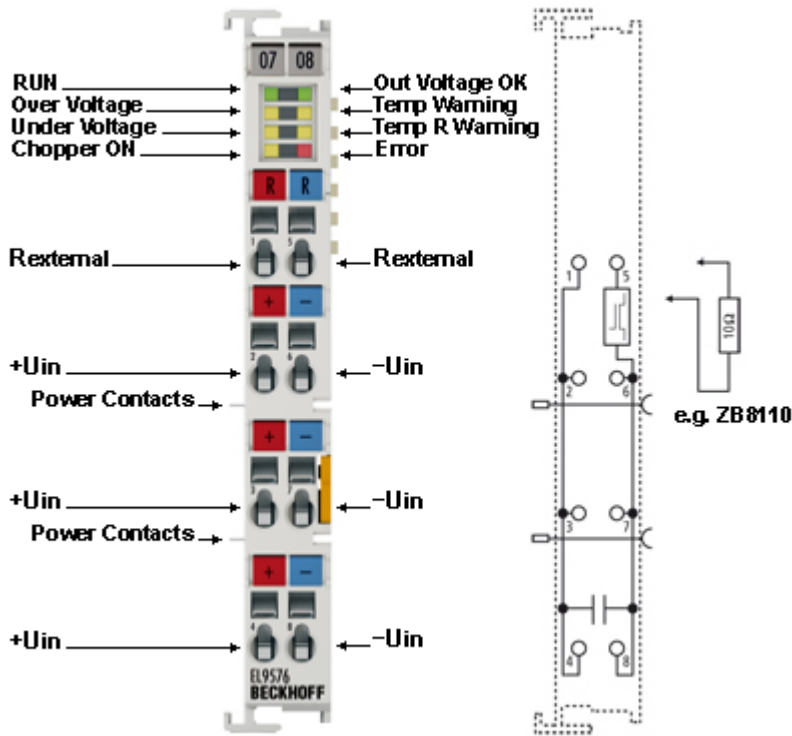
Abb. 24: LEDs und Anschlussbelegung EL9576
