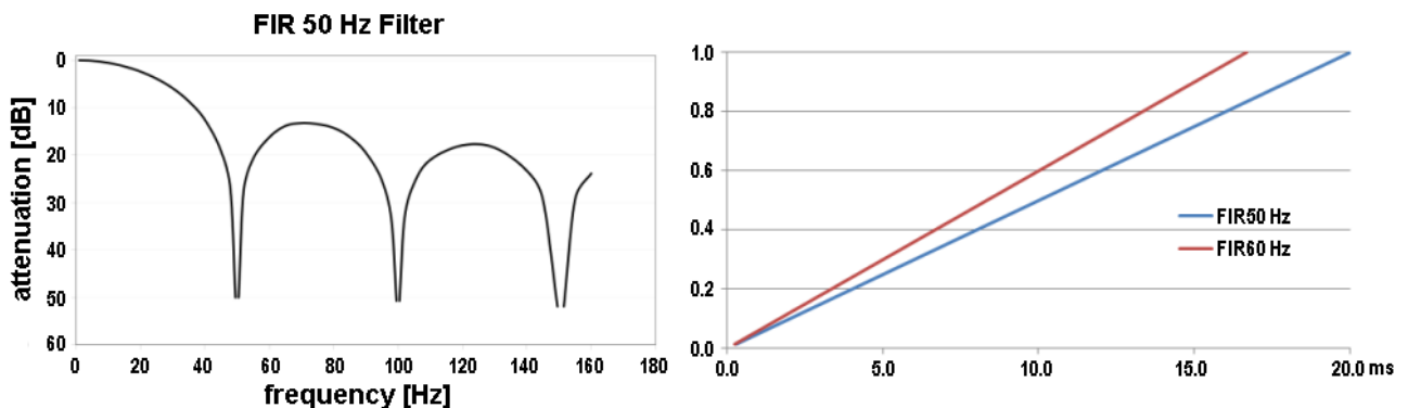
Abb. 94: Notch-Kennlinie/Amplitudengang und Sprungantwort der FIR-Filter
