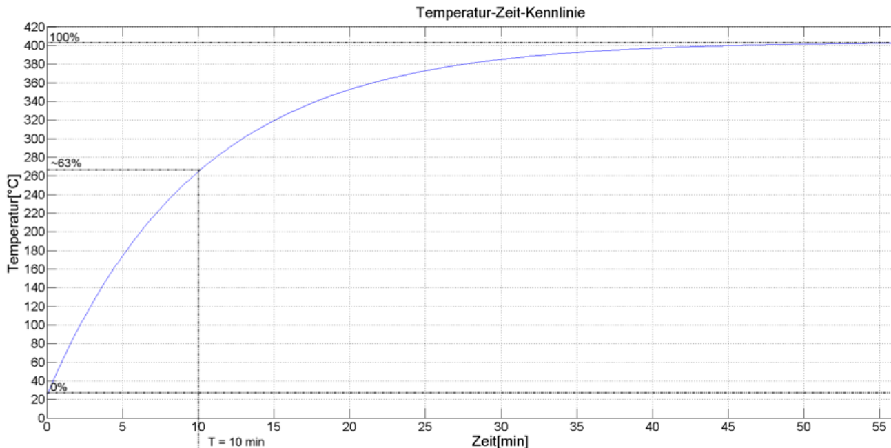
Abb. 97: Temperaturanstieg bei Nennlast
