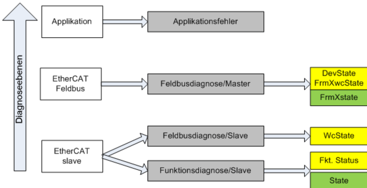
Abb. 84: Auswahl an Diagnoseinformationen eines EtherCAT Slave
