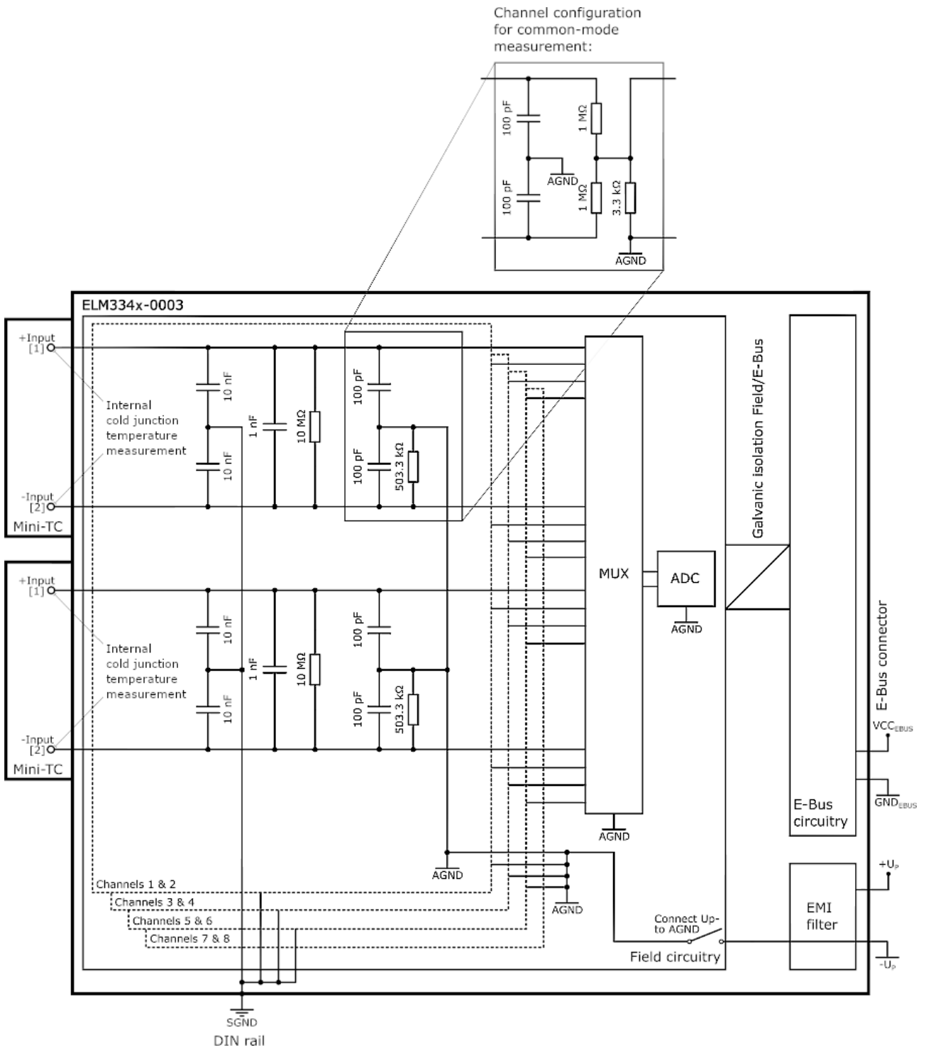
Fig. 354: Potentials schematics ELM334x-0003
