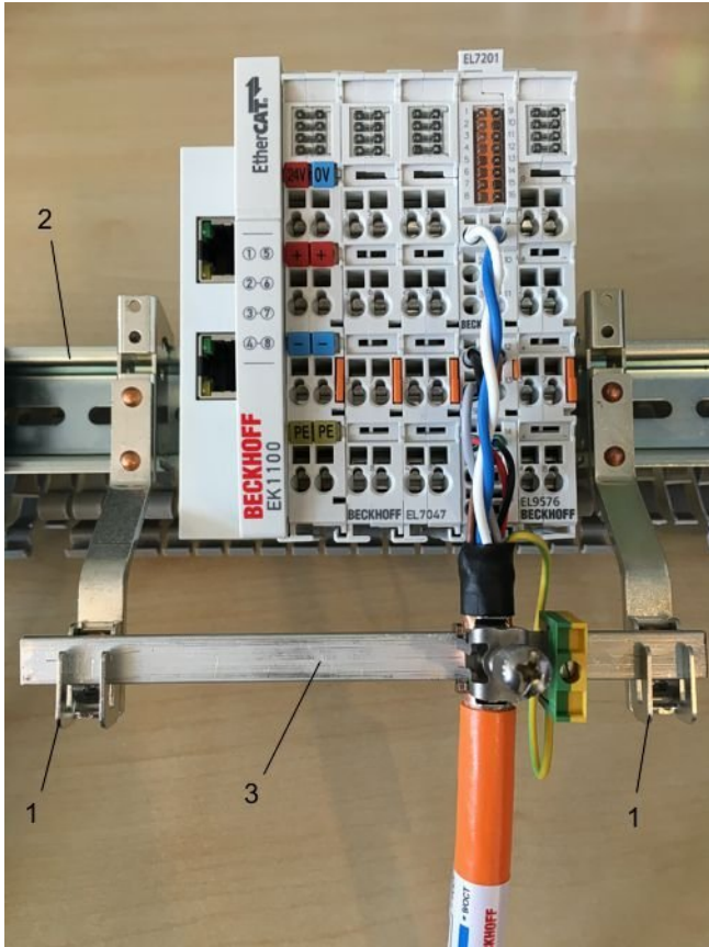
Fig. 343: Shield busbar
