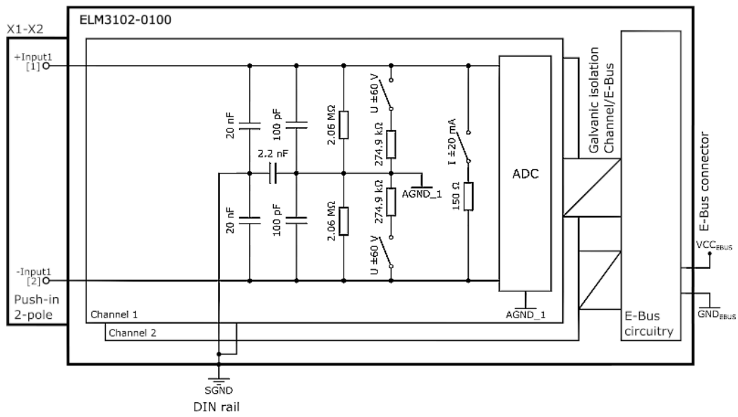
Fig. 349: Potentials schematics ELM3102-0100
