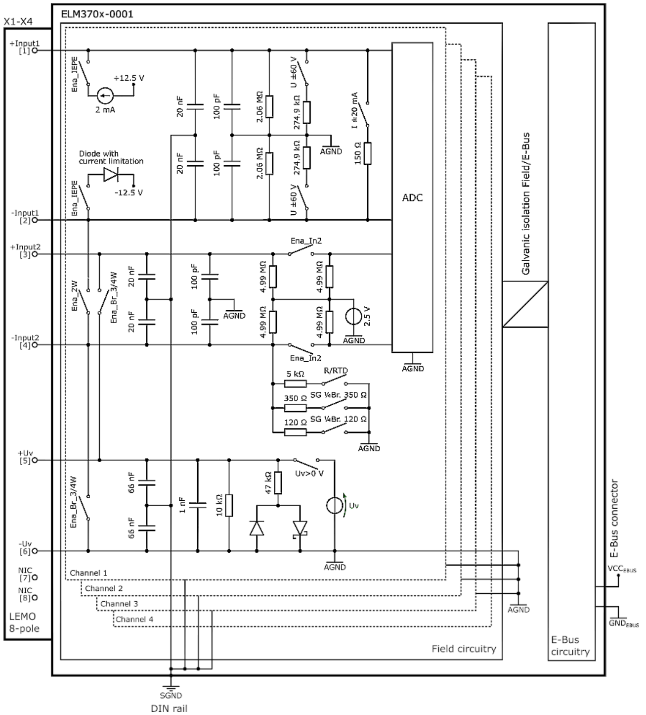
Fig. 359: Potentials schematics ELM370x-0001
