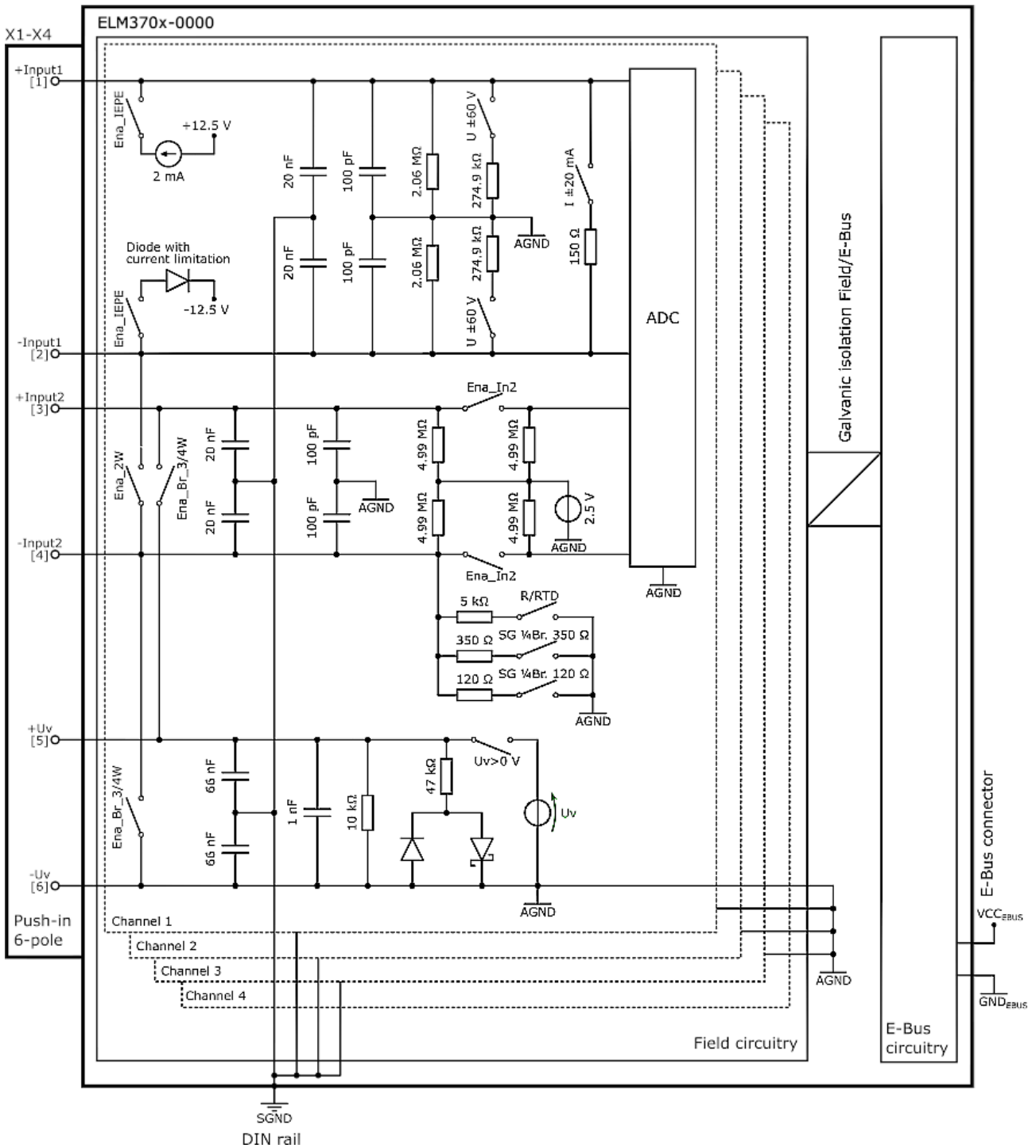
Fig. 358: Potentials schematics ELM370x-0000
