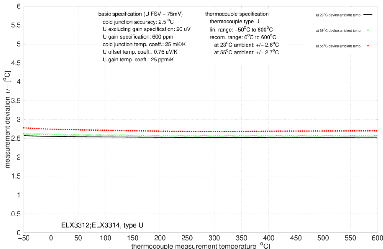
Abb. 41: Messunsicherheit für Thermoelement Typ U
