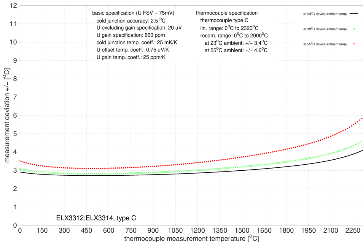
Abb. 32: Messunsicherheit für Thermoelement Typ C
