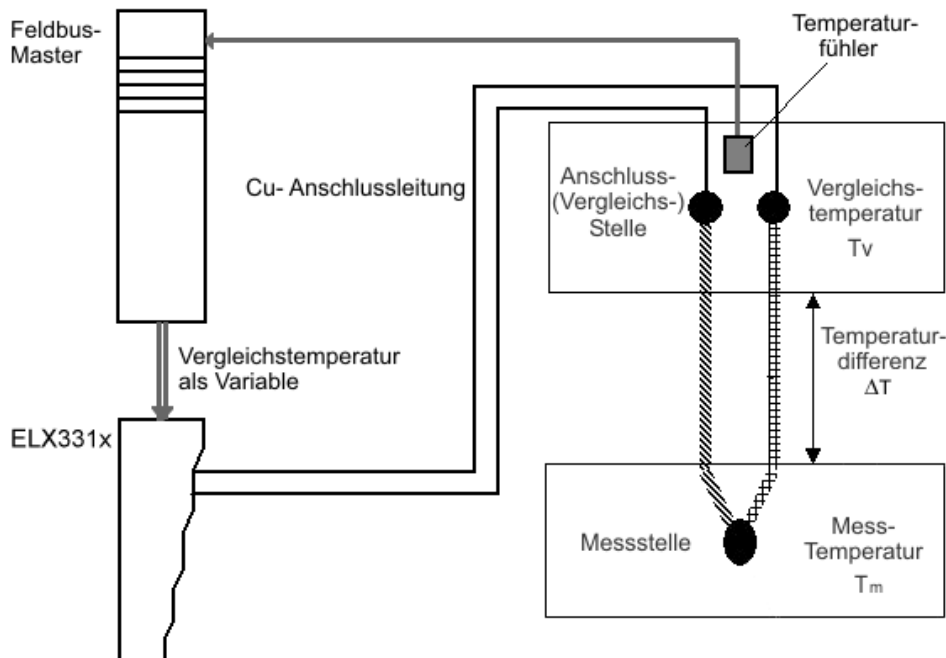
Abb. 44: Externe Vergleichsstelle
