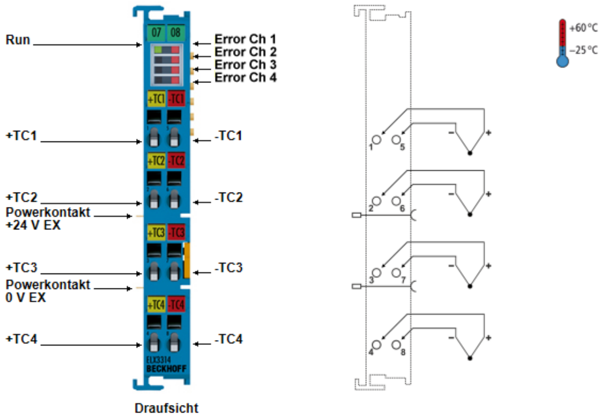
Abb. 21: ELX3314 - Anschlussbelegung
