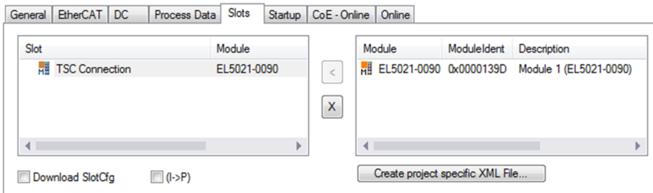
Abb. 51: Hinzufügen der TwinSAFE-SC-Prozessdaten unterhalb der Komponente z.B. EL5021-0090
