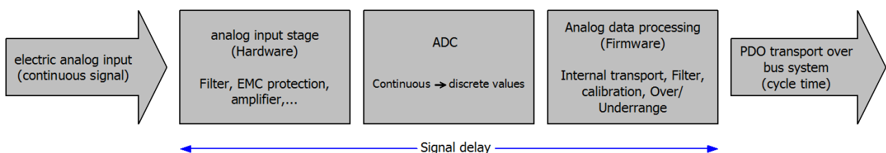
Abb. 27: Signalverarbeitung Analogeingang
