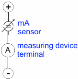
Abb. 24: 2-Leiter-Anschluss
