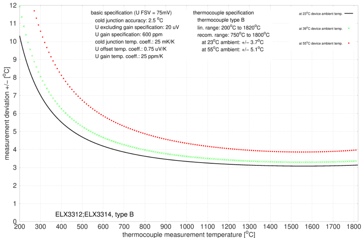
Abb. 31: Messunsicherheit für Thermoelement Typ B
