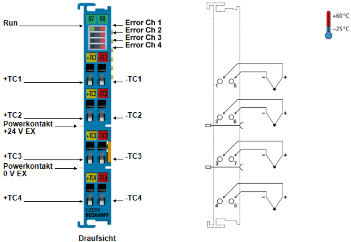
Abb. 5: ELX3314 - Vierkanalige Analog-Eingangsklemme für Thermoelemente, 16 Bit, Ex i
