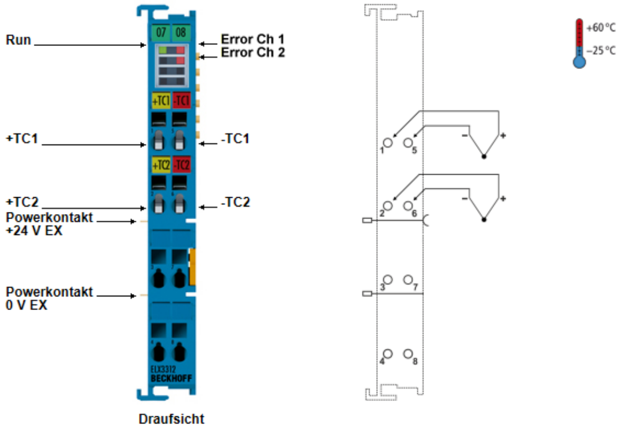
Abb. 4: ELX3312 - Zweikanalige Analog-Eingangsklemme für Thermoelemente, 16 Bit, Ex i
