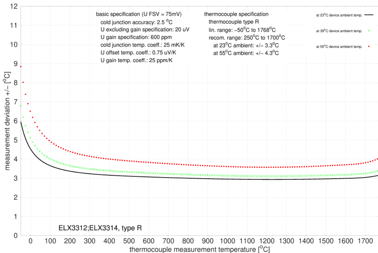
Abb. 38: Messunsicherheit für Thermoelement Typ R
