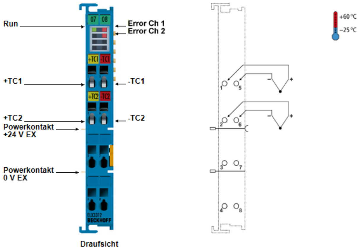
Abb. 20: ELX3312 - Anschlussbelegung
