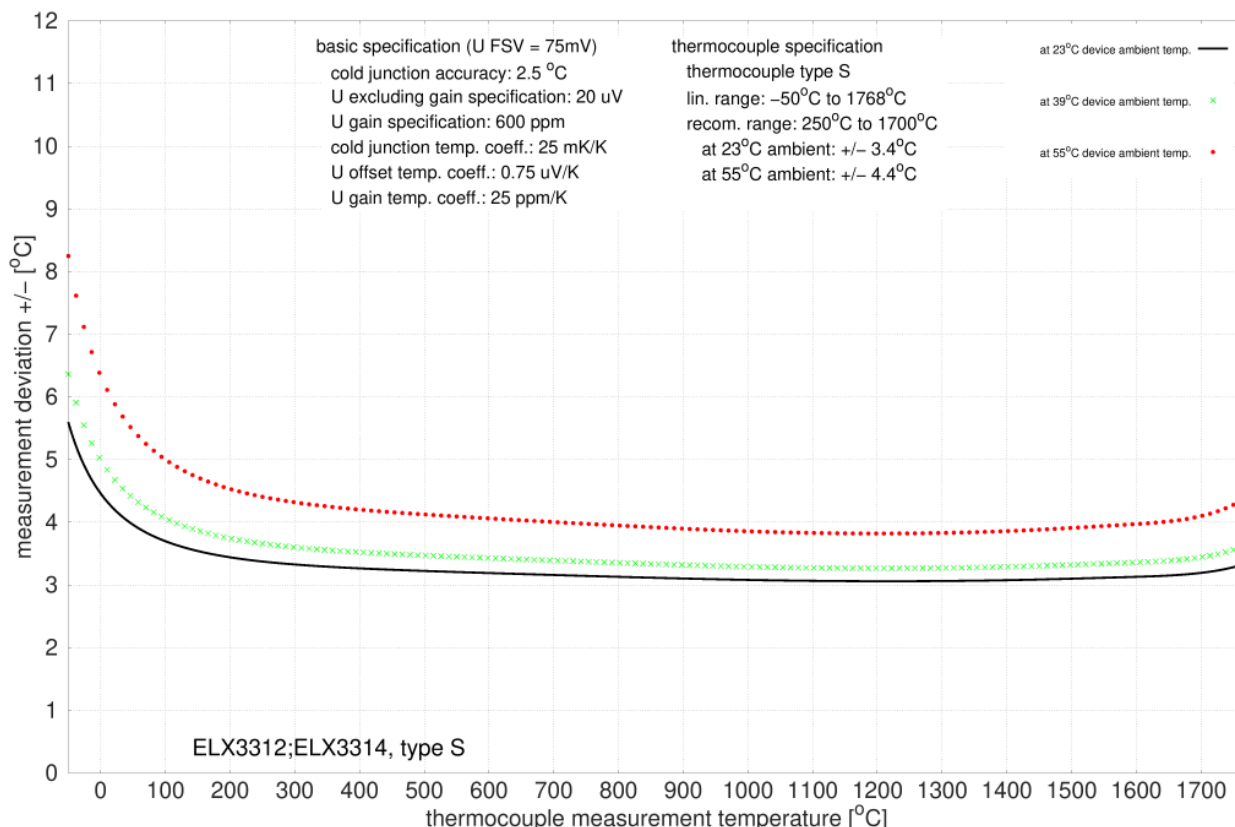
Abb. 39: Messunsicherheit für Thermoelement Typ S
