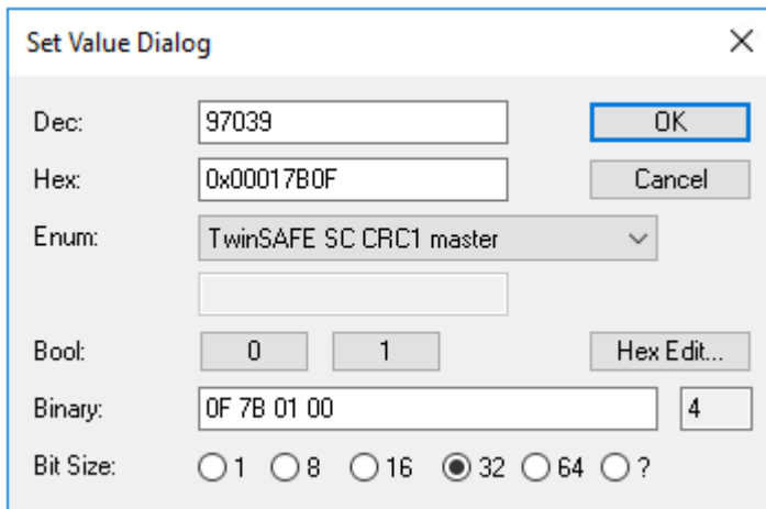
Abb. 59: Eintragen der Safety-Adresse und der CRC
