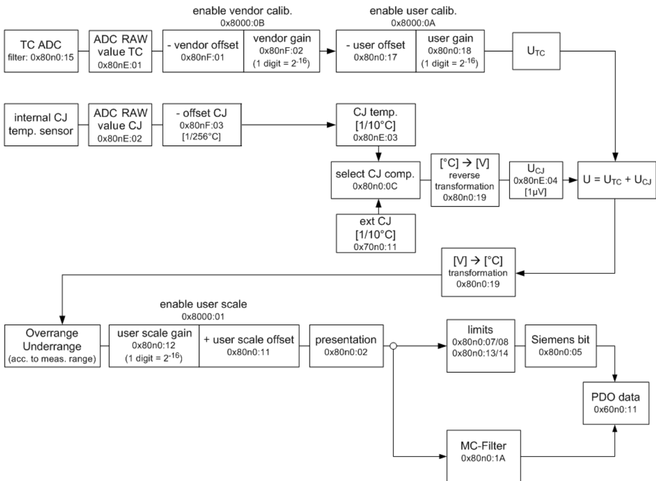
Abb. 42: ELX331x - Datenfluss
