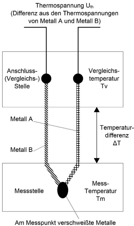
Abb. 30: Prinzip des Thermoelementes
