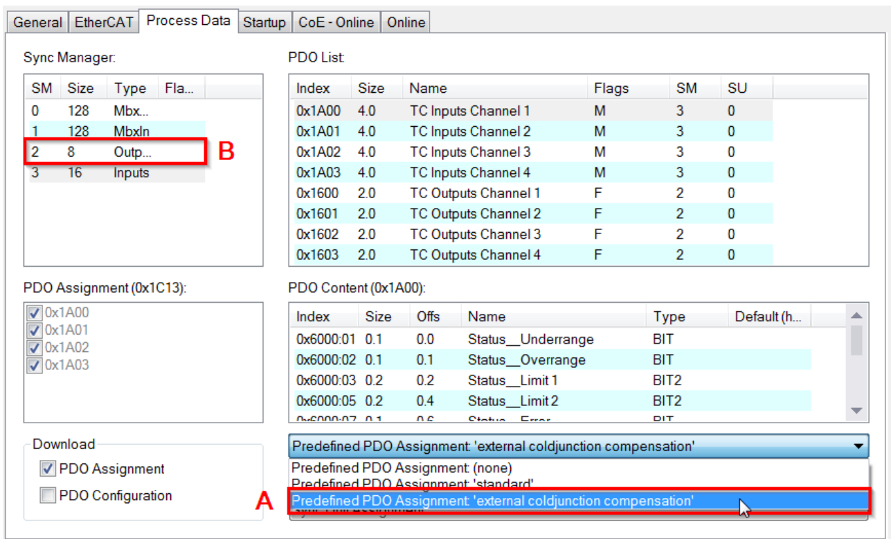
Abb. 50: TwinCAT Systemmanager mit der vordefinierten PDO-Auswahl External Compensation
