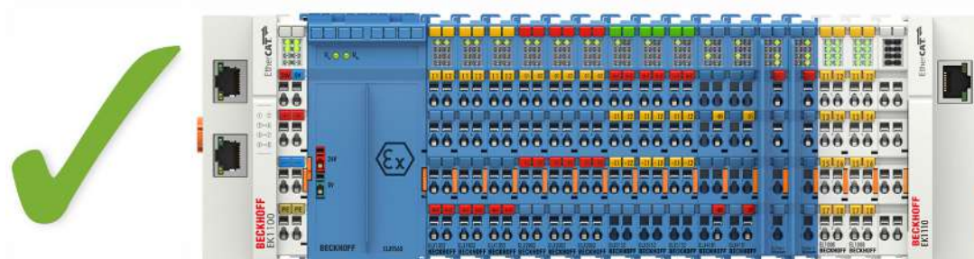
Abb. 7: Zulässige Anordnung - vor und nach dem ELX-Klemmenstrang sind Klemmen gesetzt, die nicht zur ELX-Serie gehören. Die Trennung erfolgt durch die ELX9560 zu Beginn des ELX-Klemmenstranges und zwei ELX9410 zum Ende des ELX-Klemmenstranges.
