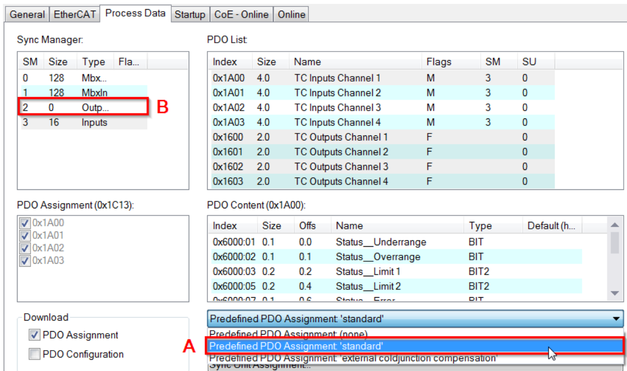
Abb. 49: TwinCAT Systemmanager mit der vordefinierten PDO-Auswahl Standard
