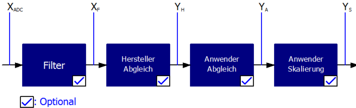
Abb. 43: Berechnung der Prozessdaten
