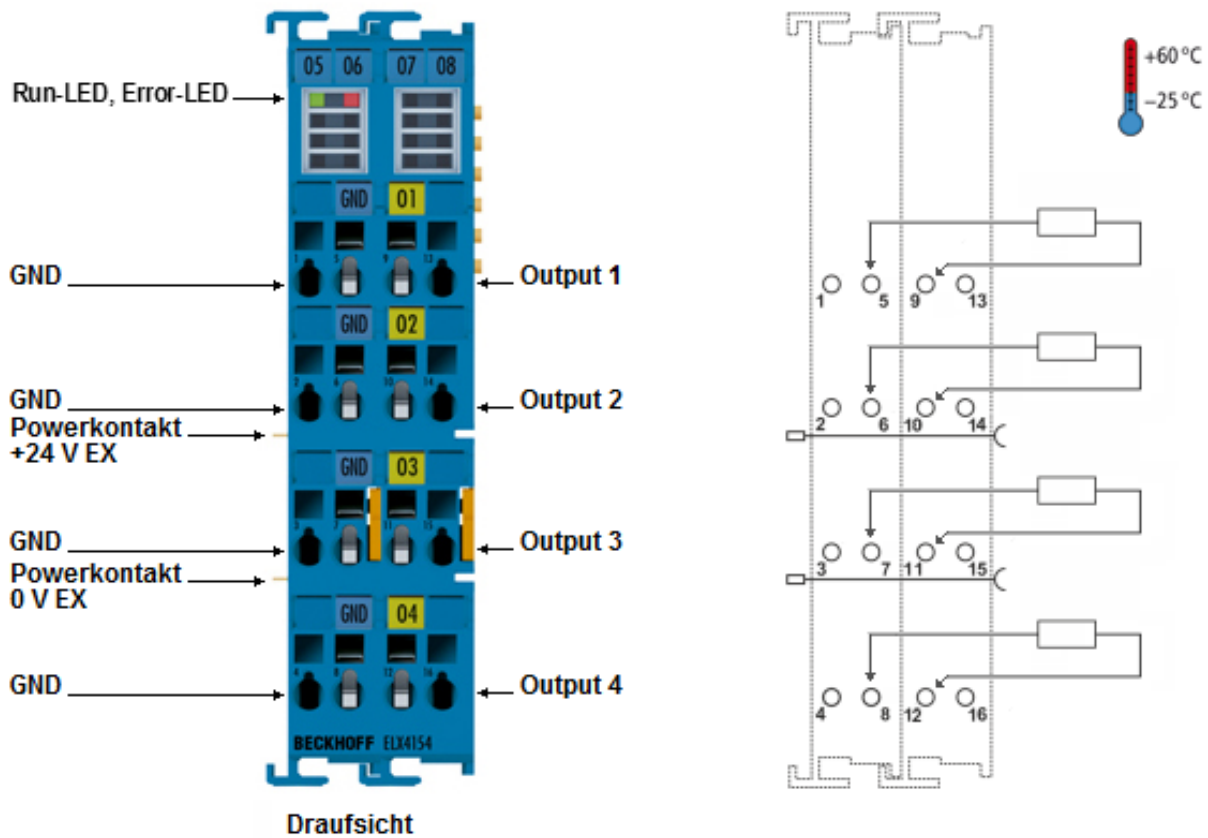
Abb. 19: ELX4154 - Anschlussbelegung
