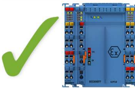
Abb. 8: Zulässige Anordnung - ELX9410 vor einer Einspeiseklemme ELX9560.
