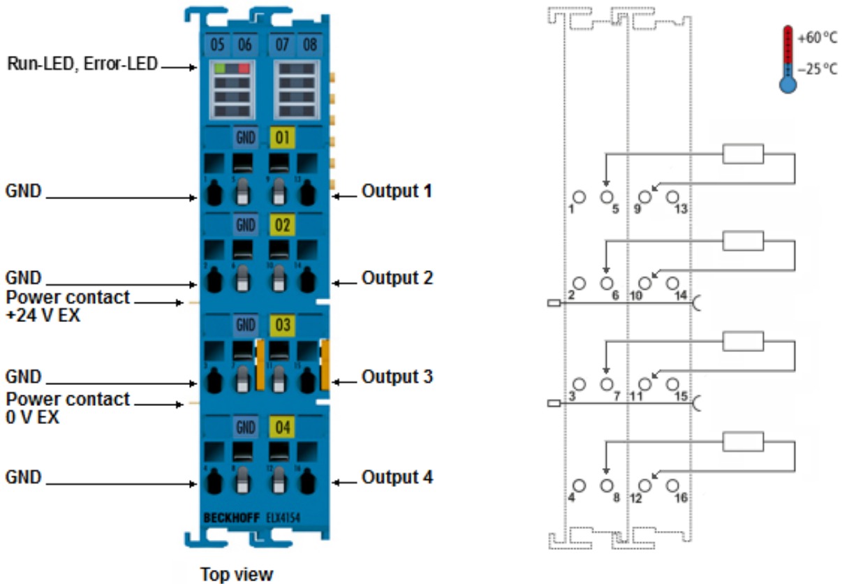
附图 19: ELX4154 - 触点分配
