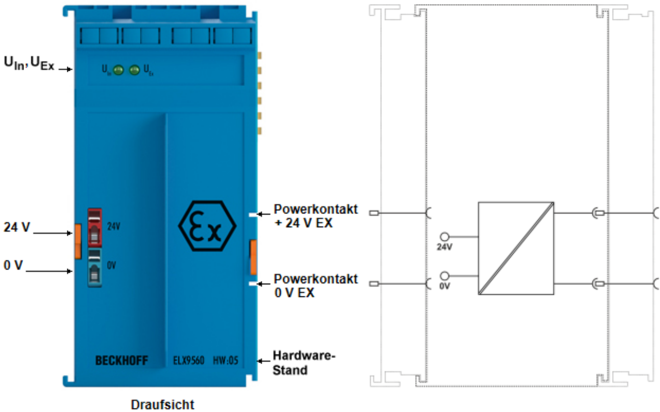
Abb. 21: ELX9560 - Anschlussbelegung
