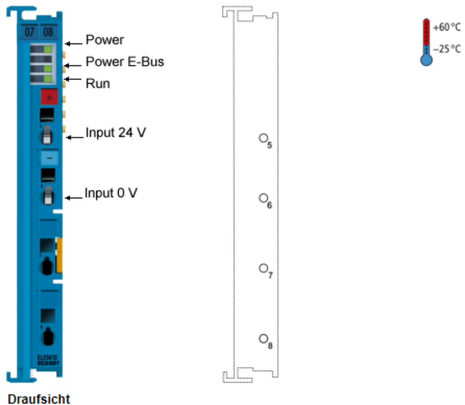
Abb. 5: ELX9410 - Einspeiseklemme zur E-Bus-Auffrischung
