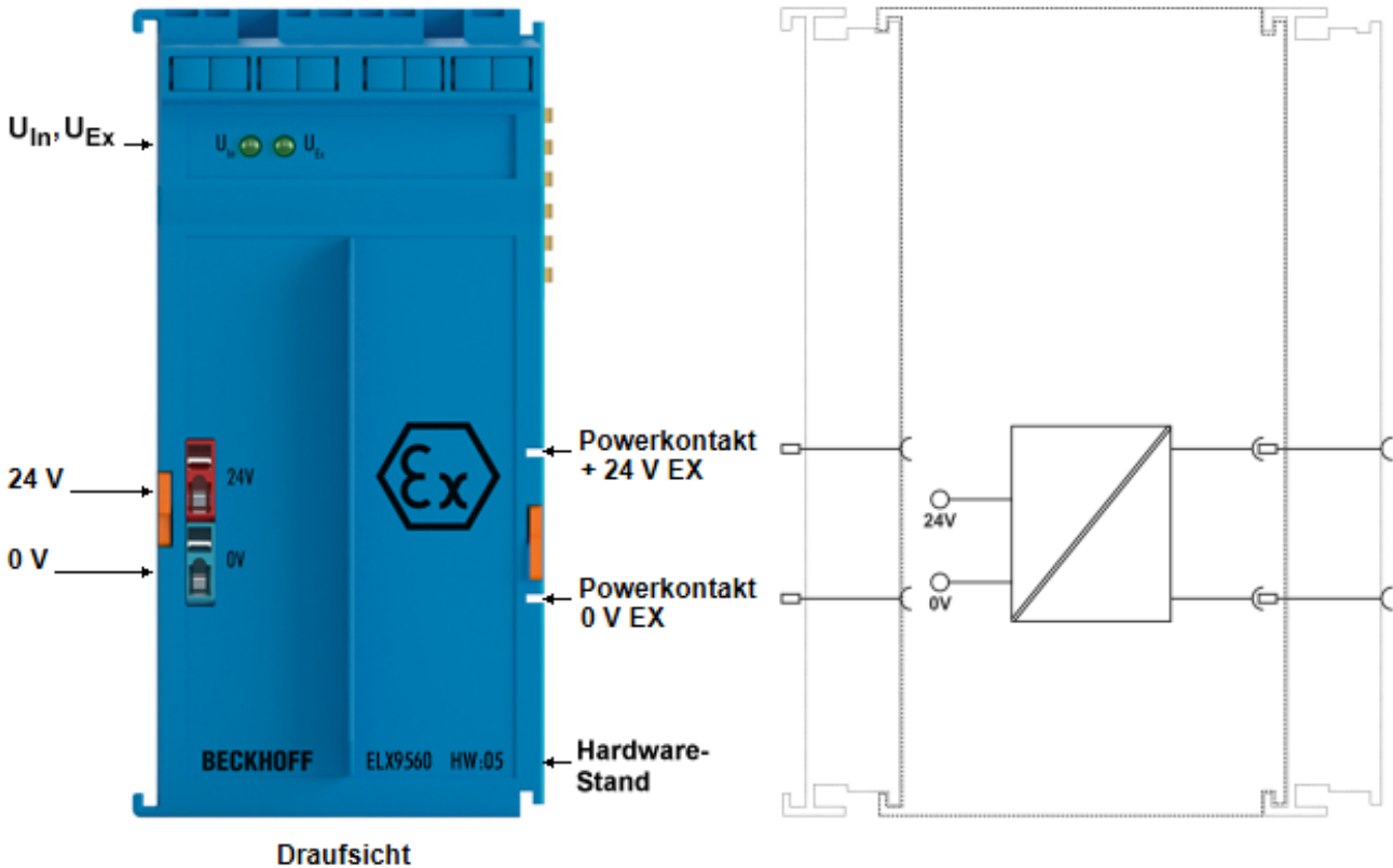
Abb. 4: ELX9560 - Einspeiseklemme, 24 V DC , potentialgetrennt
