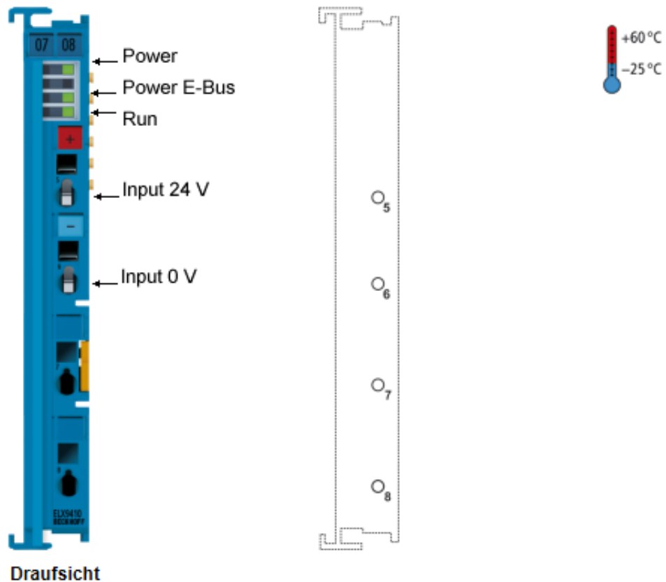
Abb. 22: ELX9410 - Anschlussbelegung
