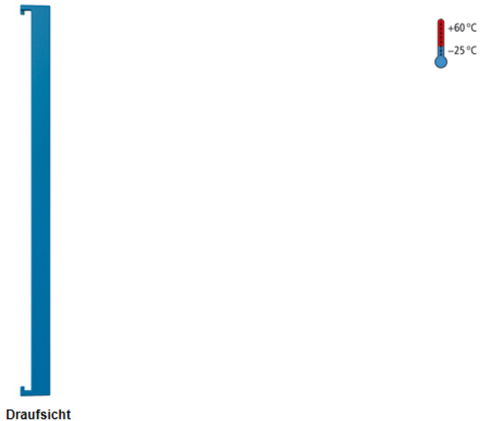
Abb. 6: ELX9012 - Busendkappe für ELXxxxx, Abdeckung der Power- und E-Bus-Kontakte, blau
