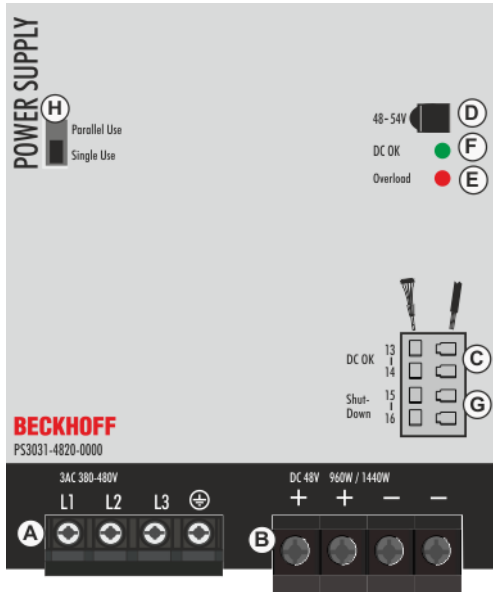
Fig. 17: PS3031-4820-0000, front
