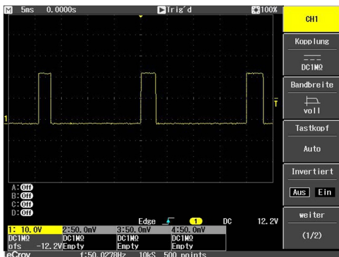
Abb. 38: Verkürzter Puls eines digitalen Ausgangs mit Last.
