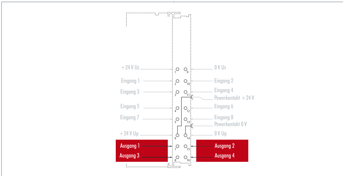
Abb. 19: Konfigurierbare digitale Ausgänge.
