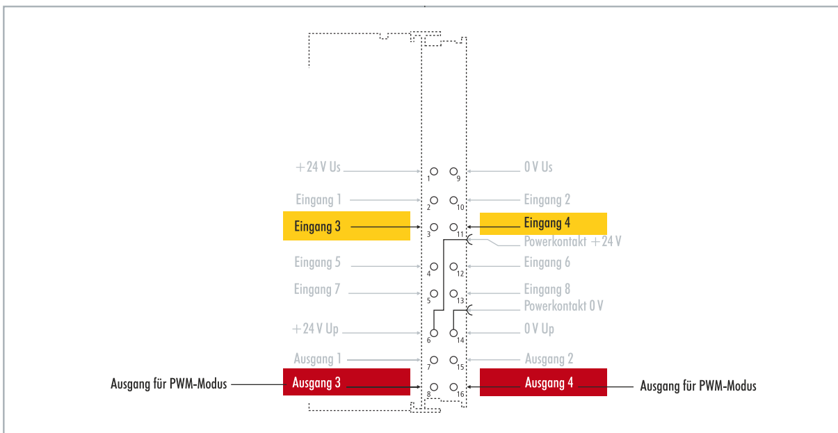
Abb. 23: Konfigurierbare Ein- und Ausgänge im PWM-Signal-Modus
