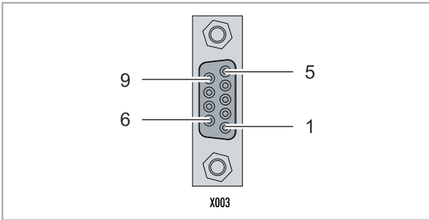
Abb. 4: PROFIBUS-Schnittstelle X003.
