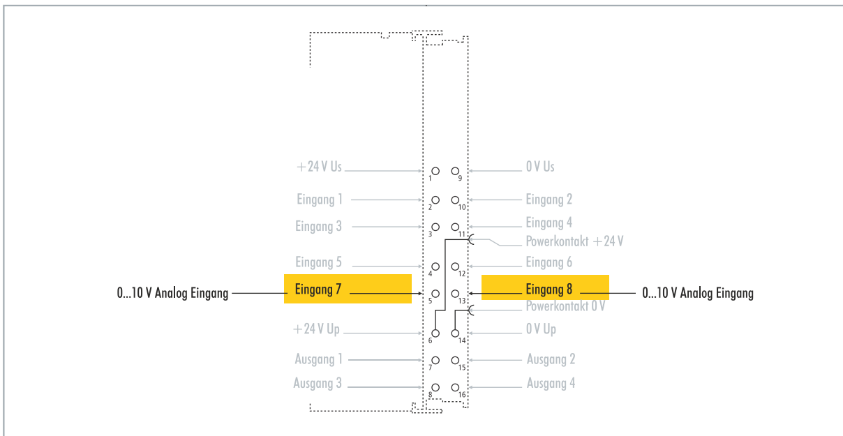
Abb. 22: Konfigurierbare analoge Eingänge.
