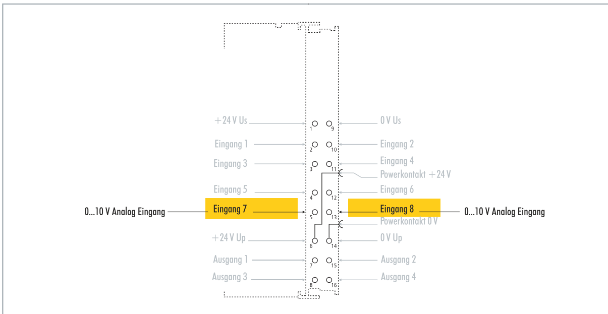
Abb. 21: Konfigurierbare analoge Eingänge.
