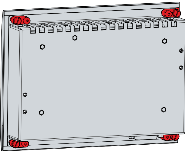
Abb. 10: Auslieferungszustand Klemmhebel
