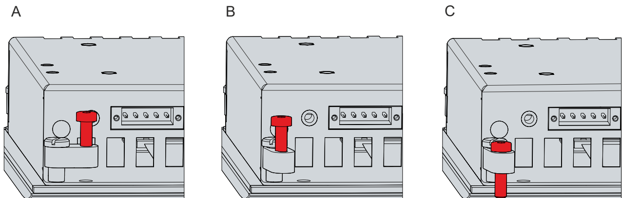
Abb. 12: Schaltschrankeinbau
