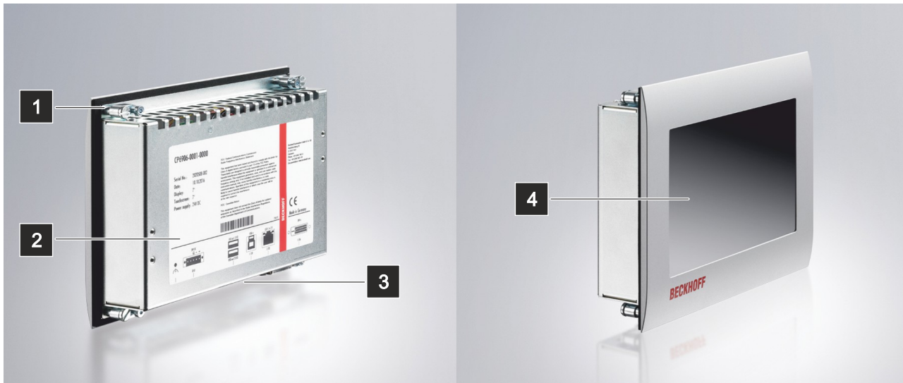
Abb. 2: Aufbau
