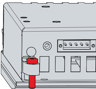
Abb. 16: Demontage aus dem Schaltschrank
