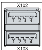
Abb. 5: USB-Schnittstelle Pin-Nummerierung
