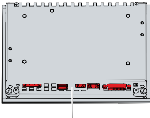
Abb. 3: Anschlussbereich
