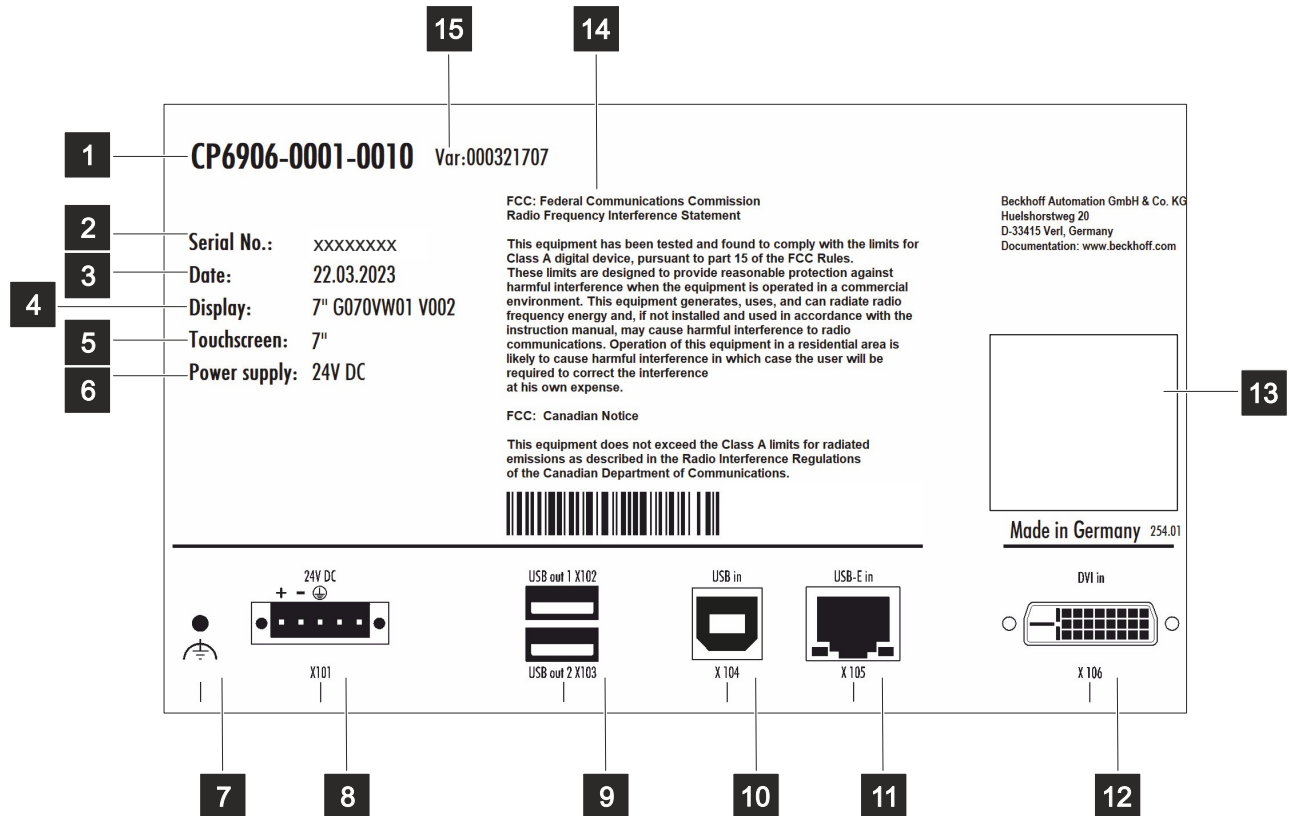
Abb. 9: Typenschild
