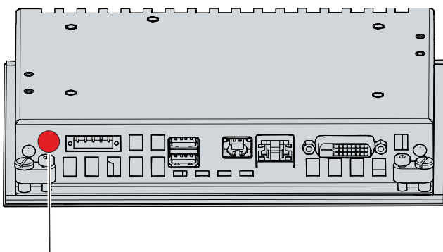
Abb. 13: Erdungsverbindung Funktionserdung
