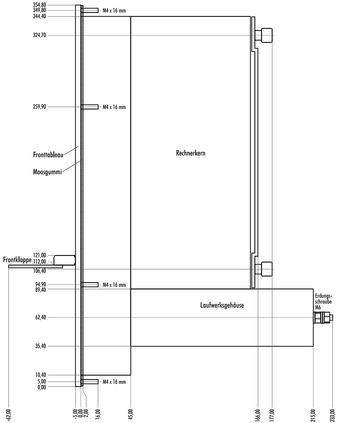
Diese Abbildung zeigt die Seitenansicht des Industrie-PCs MIC3110.
