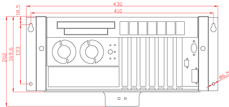
Frontansicht
