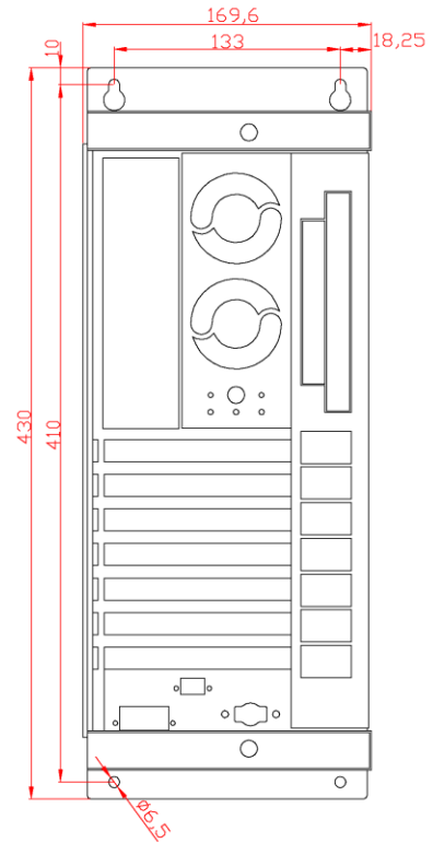
Frontansicht
