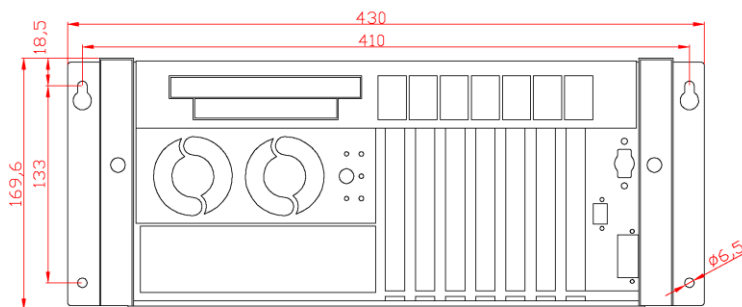
Frontansicht
