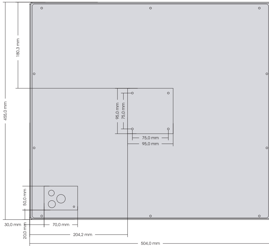
Rückansicht CP7903-M233
